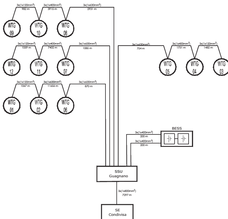
Figura 1 - Schema di collegamento tra WTG - SSU - SE Condivisa
