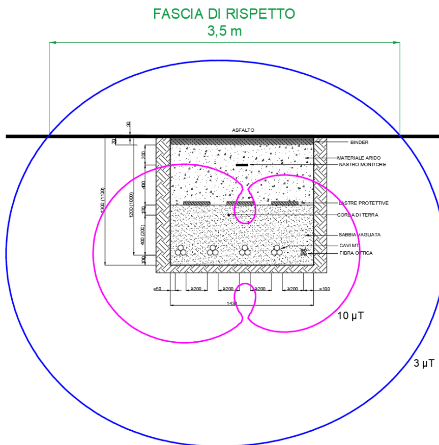
Figura 9: Curve Equicampo –4 Terne cavi MT (su strada asfaltata)
