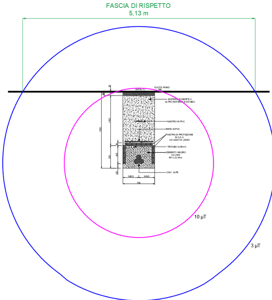
Figura 12: Curve Equicampo -1 Terna cavi AT (su strada asfaltata) - Tratta tra SE Condivisa e Stazione RTN
