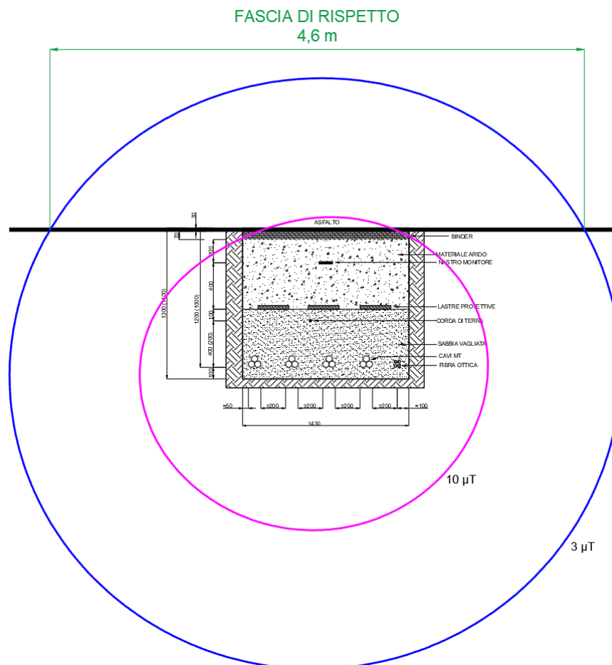
Figura 10: Curve Equicampo -4 Terne cavi MT (su strada asfaltata)
