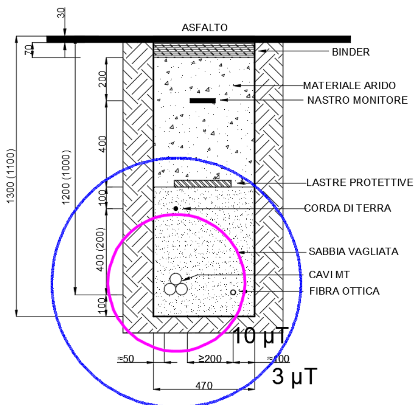
Figura 5: Curve Equicampo -Una Terna cavi MT - Tratta 1 (su strada asfaltata)
