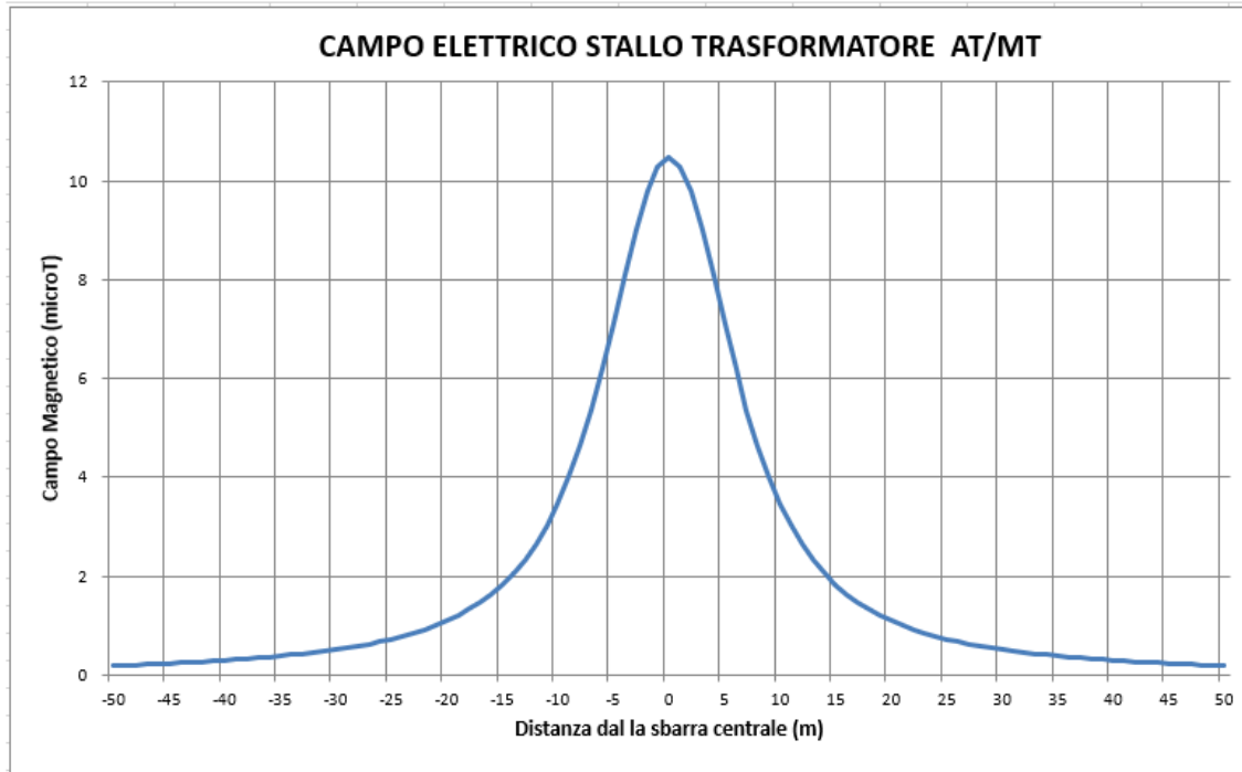
Figura 15: Valori del campo magnetico stallo Trafo AT/MT
