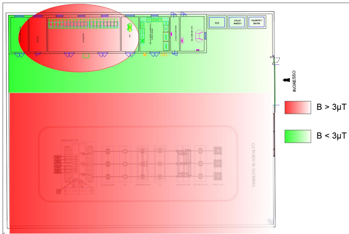
Figura 13: Limiti di esposizione all'interno dell'Area di Sottostazione
