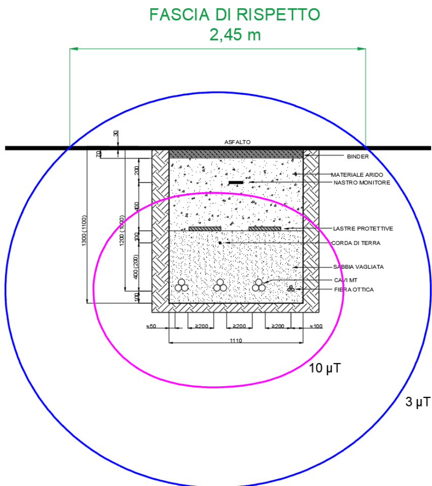
Figura 7: Curve Equicampo –Tre Terne cavi MT (su strada asfaltata)
