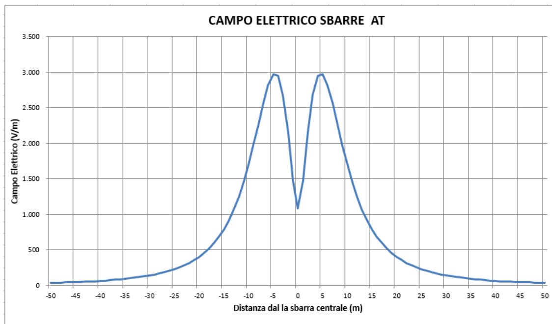
Figura 16: Valori del campo elettrico stallo Trafo AT/MT
