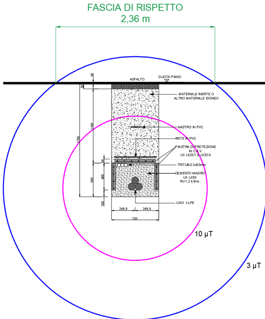
Figura 11: Curve Equicampo -1 Terna cavi AT (su strada asfaltata) - Tratta tra SSU e SE Condivisa
