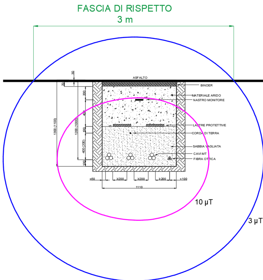
Figura 8: Curve Equicampo –3 Terne cavi MT (su strada asfaltata)
