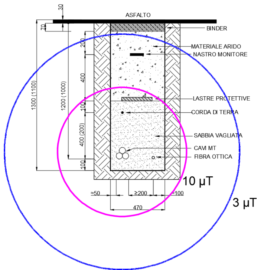
Figura 6: Curve Equicampo -Una Terna cavi MT - Tratta 2 (su strada asfaltata)
