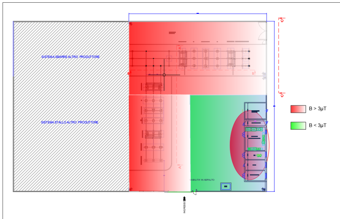
Figura 14: Limiti di esposizione all'interno dell'Area di Sottostazione Condivisa
