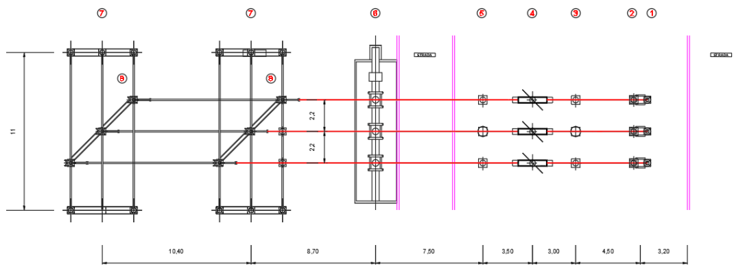
Figura 13 - Planimetria apparecchiature stallo 150 kV nella SE Terna
