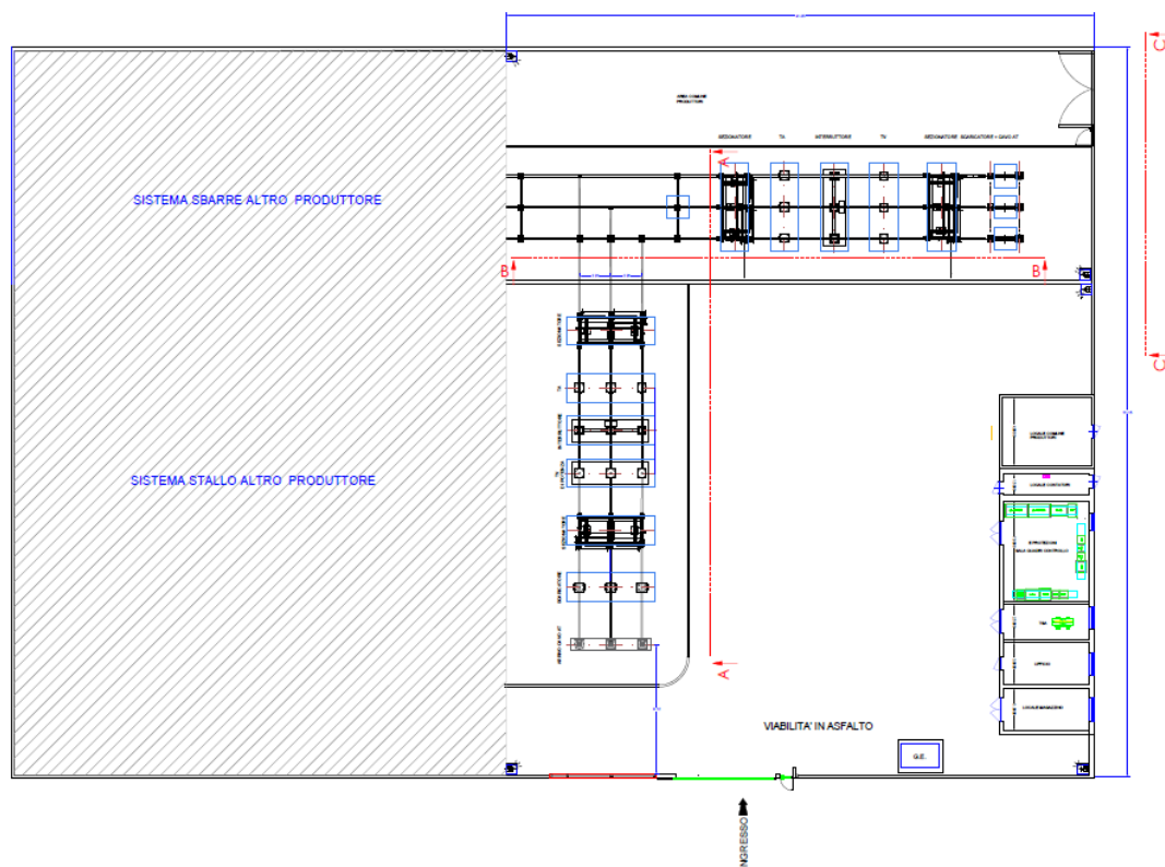
Figura 5 - Planimetria SE condivisa.
