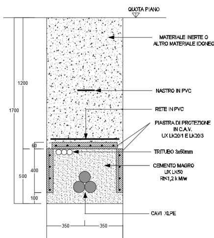
Figura 11 - Sezione tipo cavi AT.
