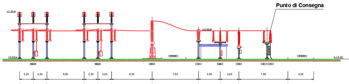
Figura 14 - Sezione apparecchiature stallo 150 kV nella SE Terna.
