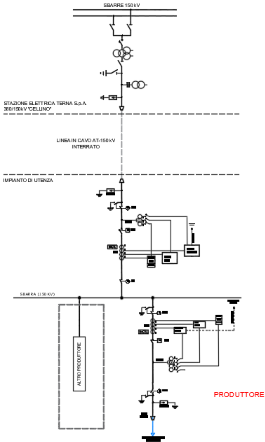
Figura 10 - Schema elettrico.
