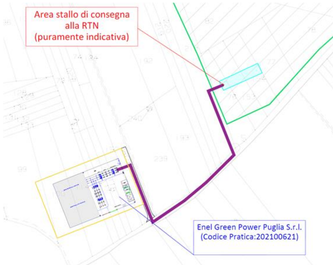
Figura 12 - Individuazione su ortofoto Stallo AT nella SE Terna
