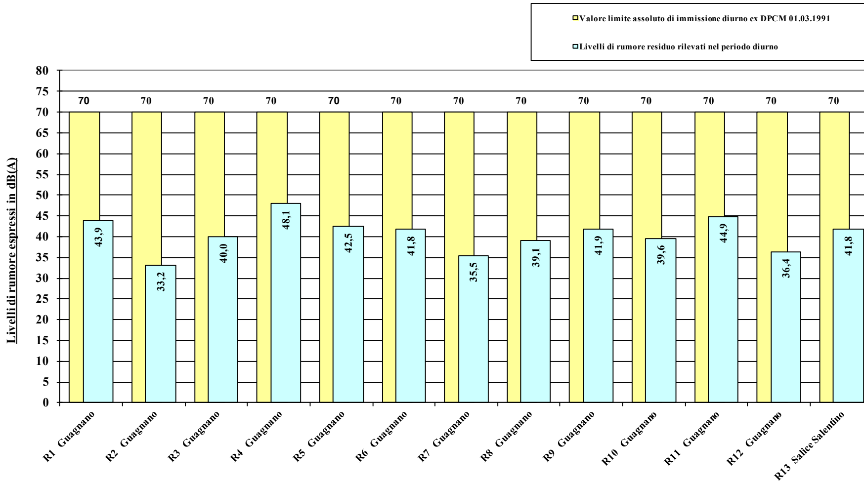
Figura 2 - Livelli di rumore ambientale (residuo) - La[ \text{dB(A)} ] - in esterno - nel tempo di riferimento diurno
