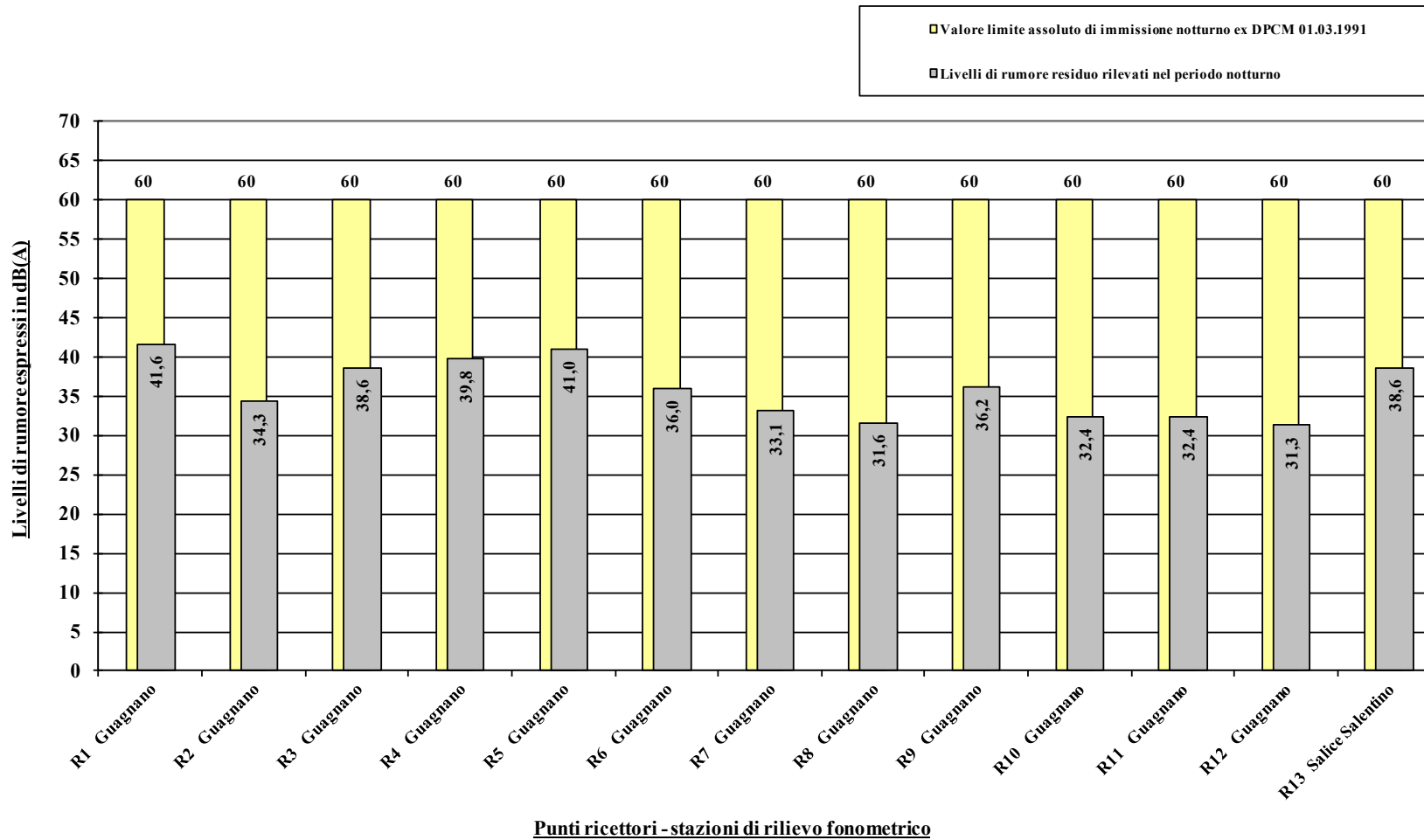
Figura 3 - Livelli di rumore ambientale (residuo) - La[dB(A)] - in esterno - nel tempo di riferimento notturno
