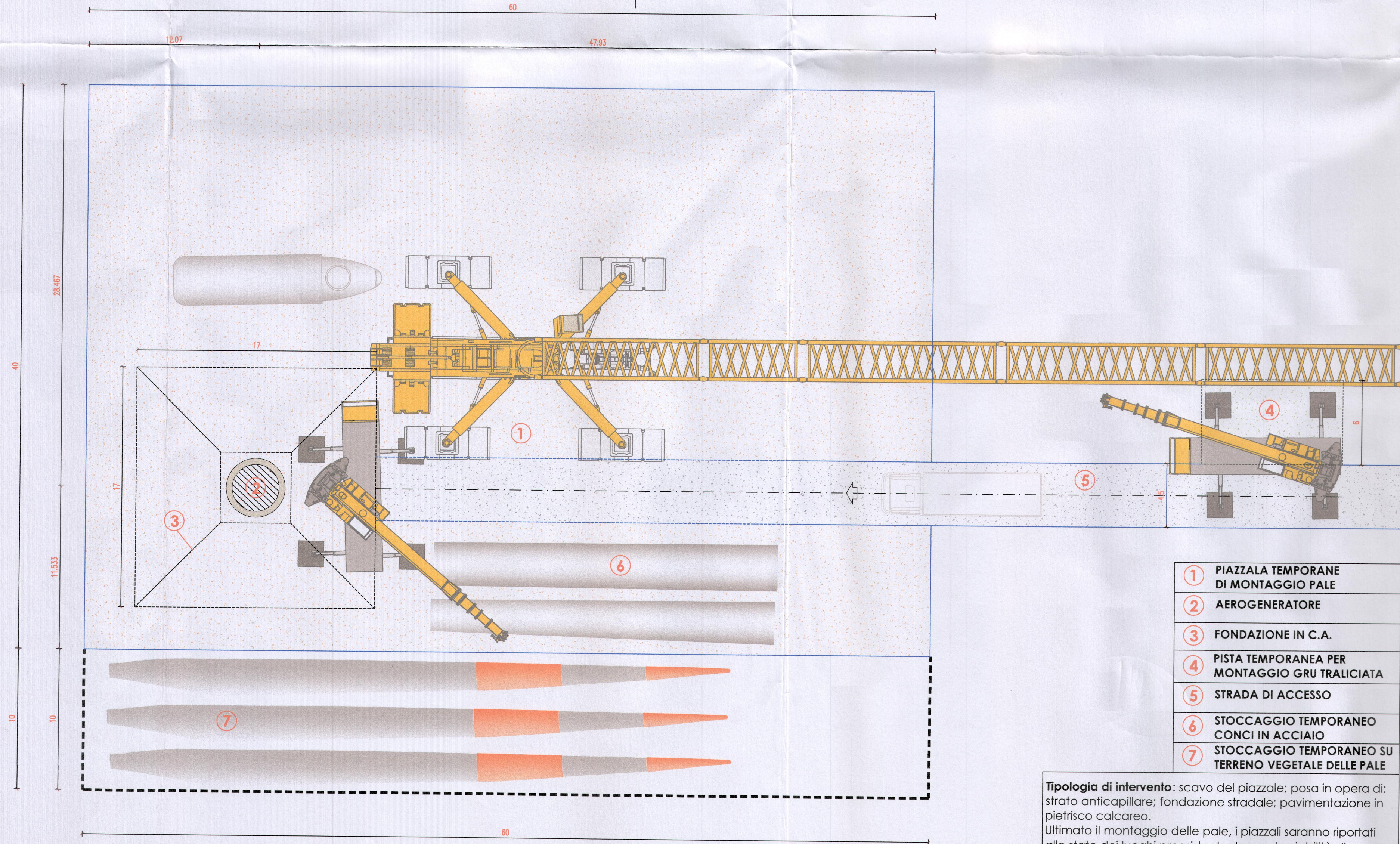
SEZIONE TIPO PIAZZOLA DI MONTAGGIO Scala 1:100
