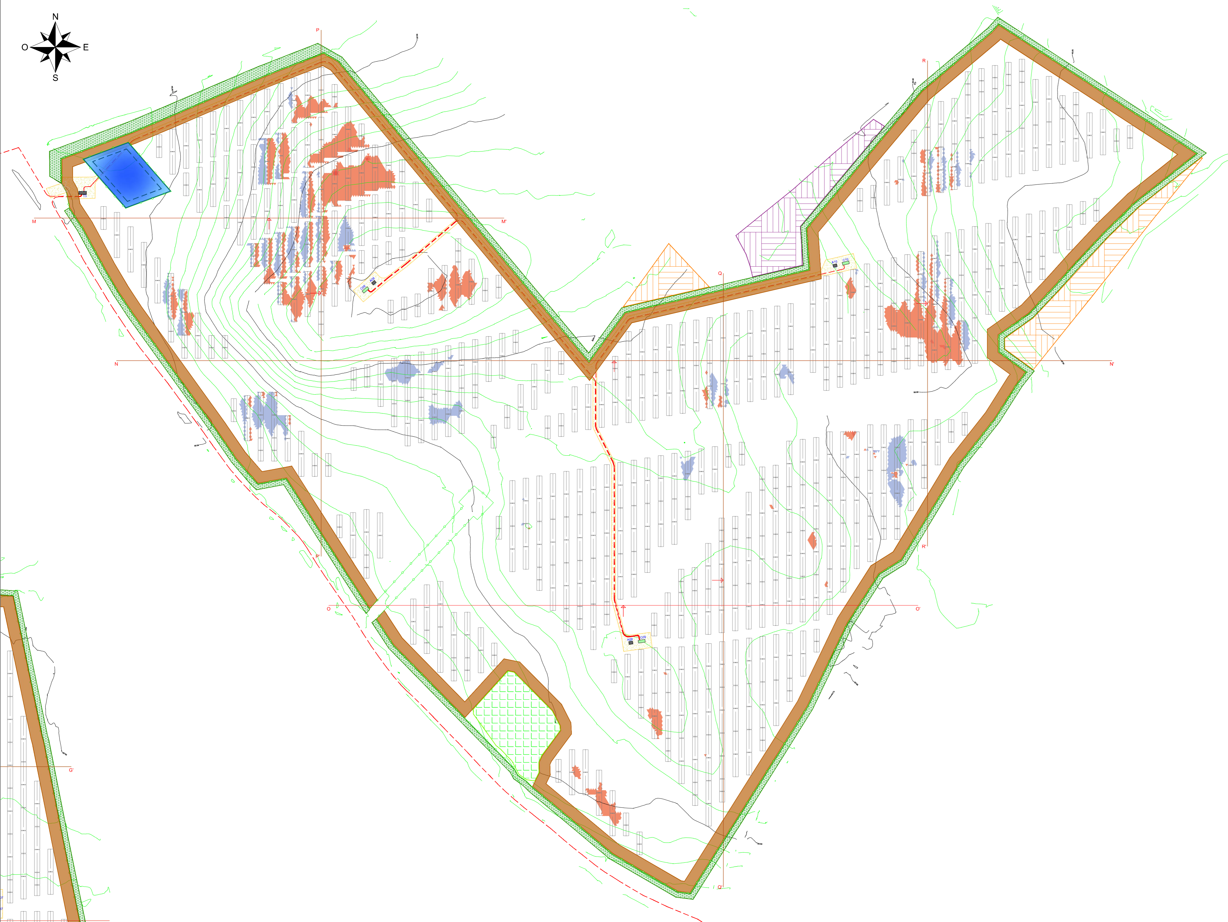
Layout impianto Area 3 - Scala 1:2000
