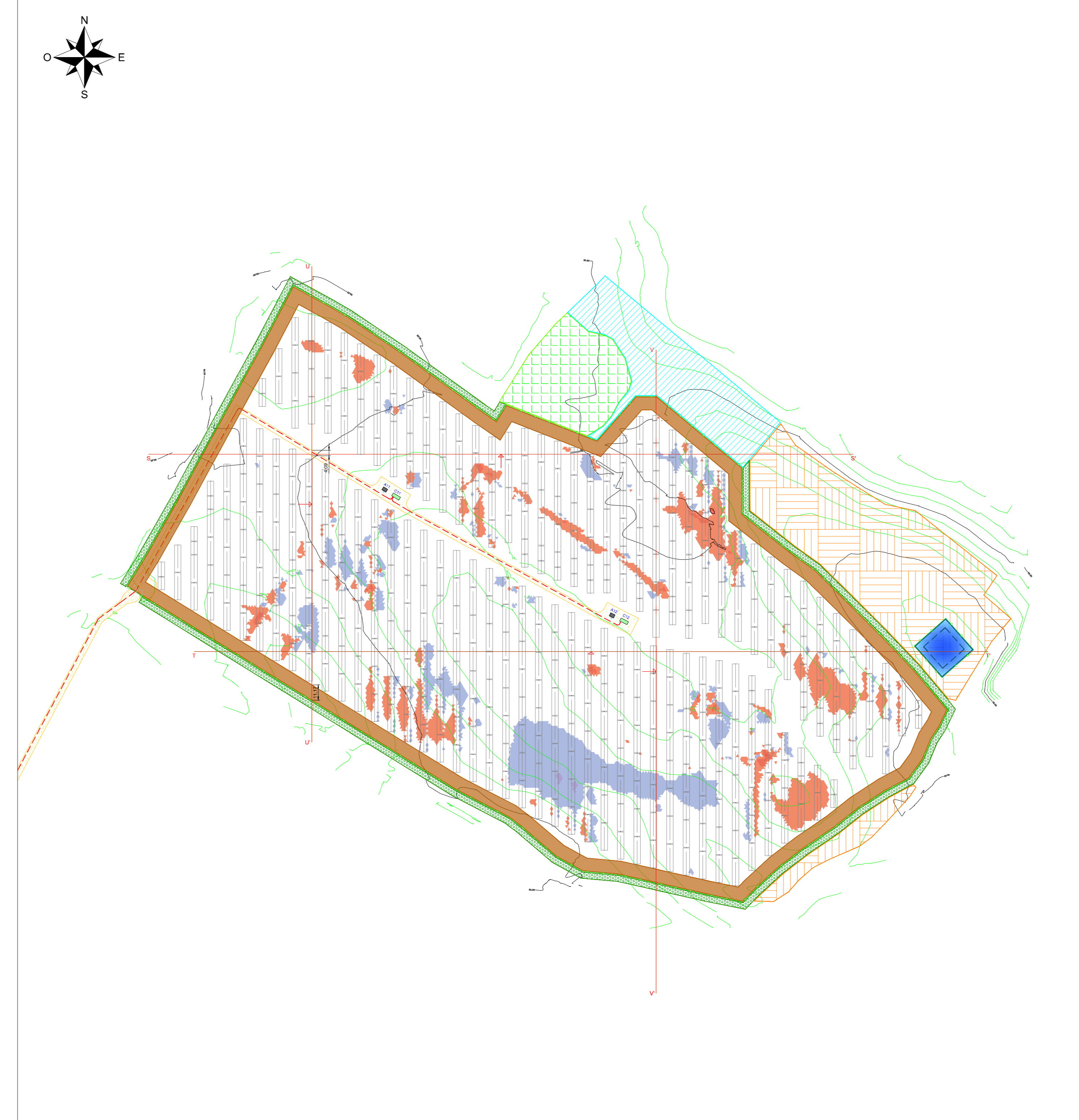
Layout impianto Area 4 - Scala 1:2000
