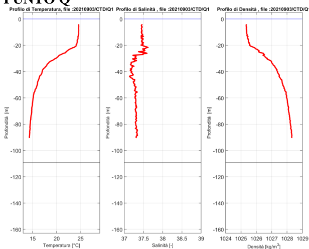
Figura 7 – Profili di temperatura (sinistra), salinità (centro) e densità (destra) misurati in D, E, F, G, O, Q in settembre 2021
