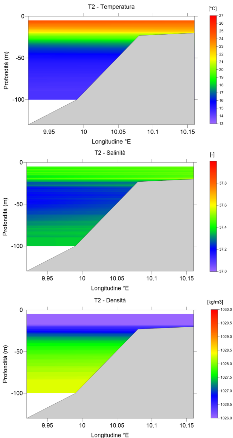
Figura 11 – Transetto T2 – Settembre 2021 – Valori caratteristici della temperatura (sopra) salinità (centro) e densità (sotto)
