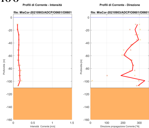
Figura 4 – Profili di corrente misurati in D, E, F, G, O, in settembre 2021
