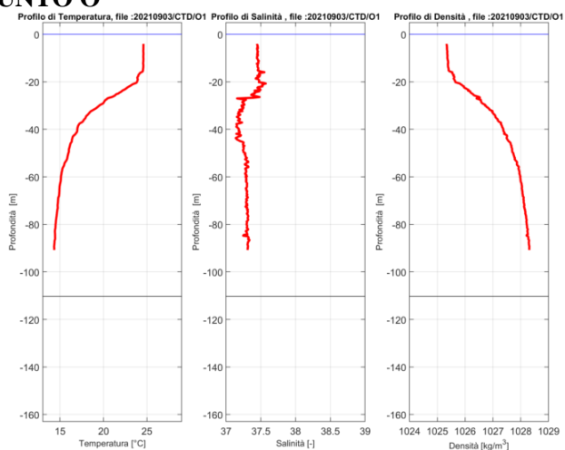
Figura 7 – Profili di temperatura (sinistra), salinità (centro) e densità (destra) misurati in D, E, F, G, O, Q in settembre 2021
