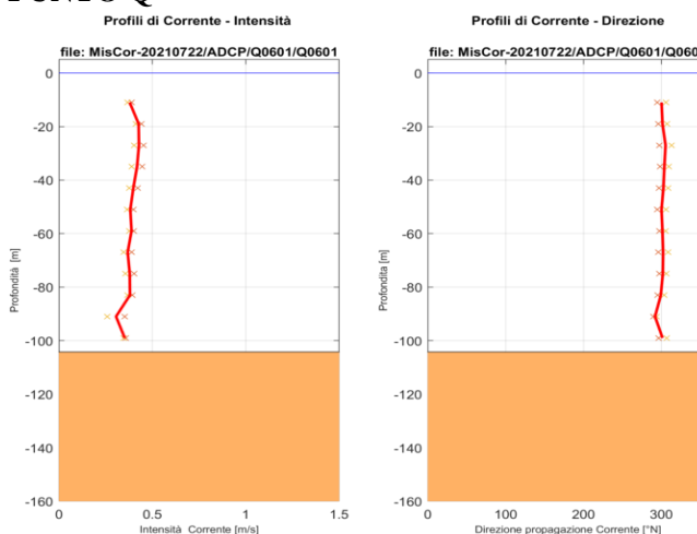
Figura 3 – Profili di corrente misurati in D, E, F, G, O, Q in luglio 2021
