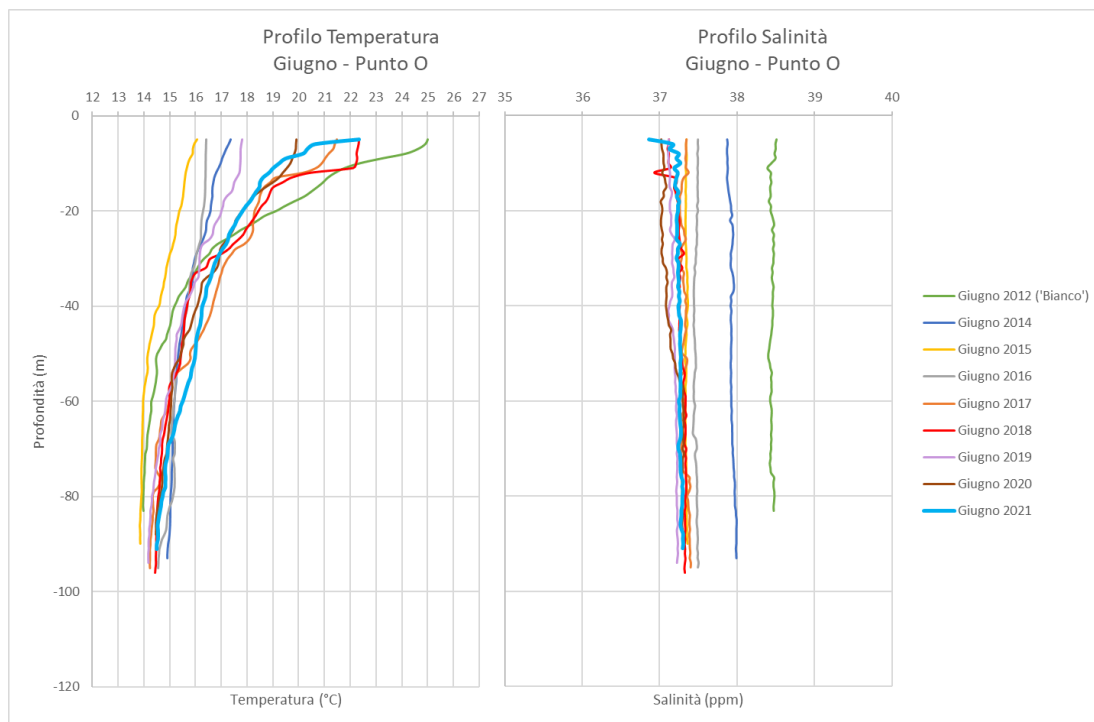
Figura 12 – Confronto tra campionamenti effettuati nel mese di giugno 2012, 2014, 2015, 2016, 2017, 2018, 2019, 2020 e 2021 al punto O
