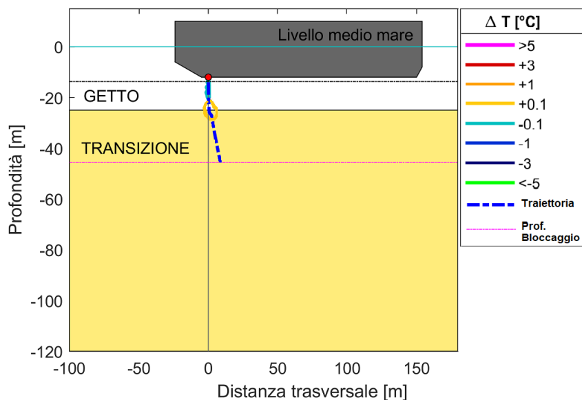
Figura 14 – Risultati modello dispersivo, scenario giugno 2021
