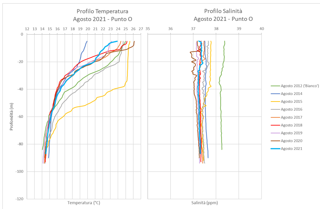
Figura 13 – Confronto tra campionamenti effettuati nel mese di agosto 2012, 2014, 2015, 2016, 2017, 2018, 2019, 2020 e 2021 (inizio settembre) al punto O
