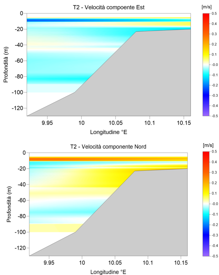
Figura 8 – Transetto T2 – Luglio 2021 – Valori caratteristici delle componenti Est (sopra) e Nord (sotto) della velocità di corrente
