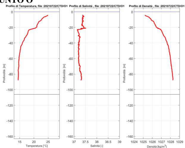
Figura 6 – Profili di temperatura (sinistra), salinità (centro) e densità (destra) misurati in D, E, F, G, O, Q in luglio 2021
