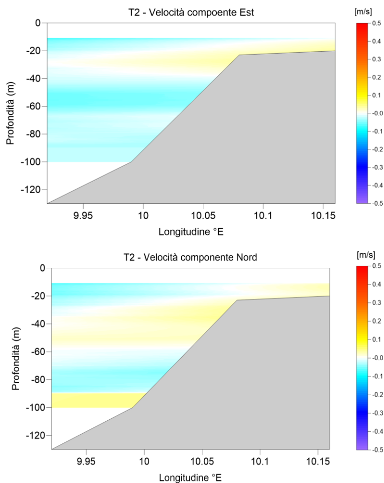
Figura 10 – Transetto T2 – Settembre 2021 – Valori caratteristici delle componenti Est (sopra) e Nord (sotto) della velocità di corrente
