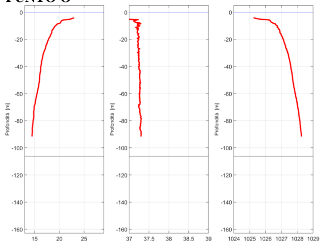
Figura 5 – Profili di temperatura (sinistra), salinità (centro) e densità (destra) misurati in O in giugno 2021
