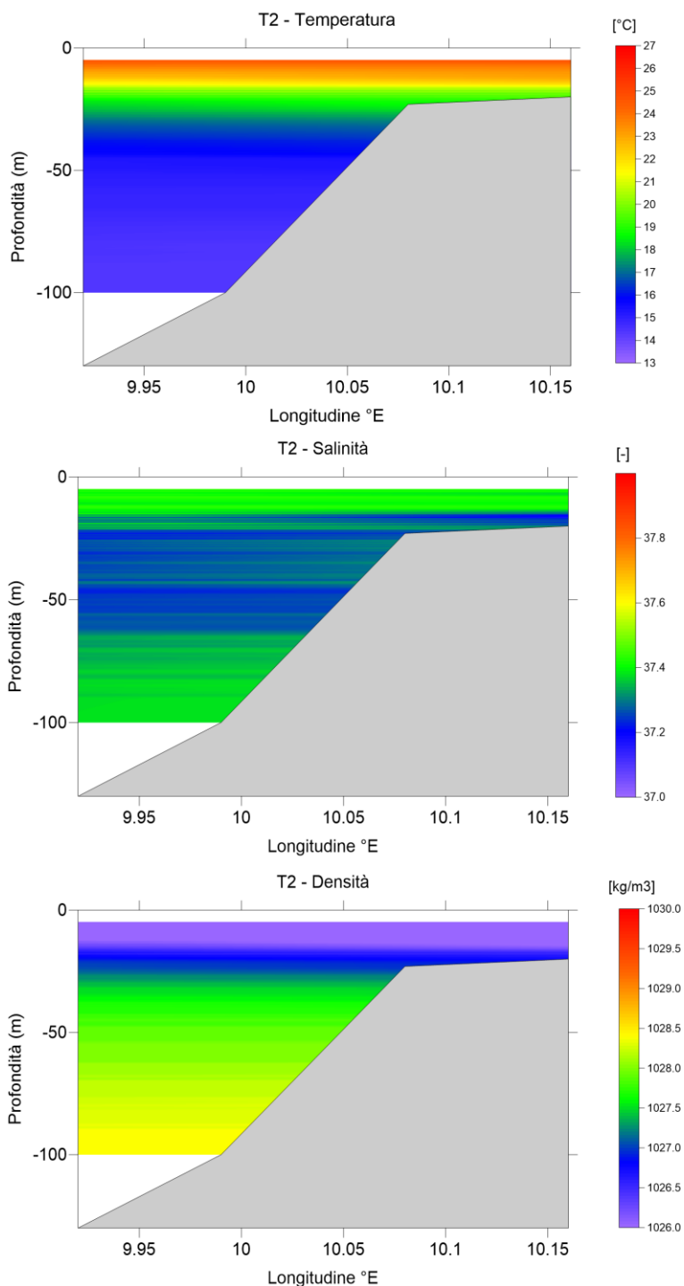
Figura 9 – Transetto T2 – Luglio 2021 – Valori caratteristici della temperatura (sopra) salinità (centro) e densità (sotto)
