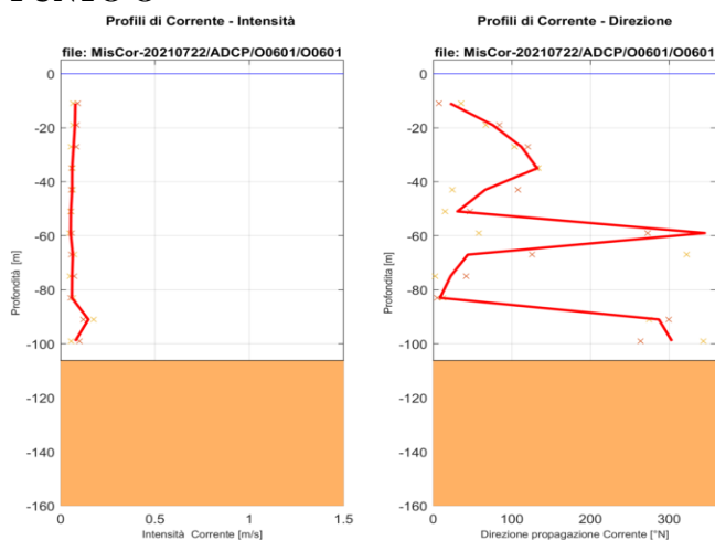
Figura 3 – Profili di corrente misurati in D, E, F, G, O, Q in luglio 2021
