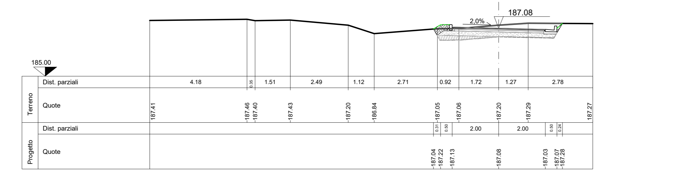
SEZ.NUM. 5 PROGR. 20.00 PARZ. 4.00
