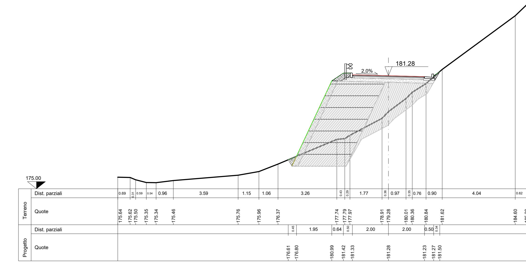
SEZ.NUM. 12 PROGR. 55.00 PARZ. 5.00
