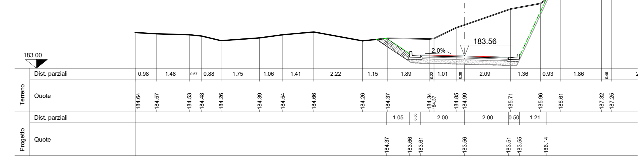
SEZ.NUM. 10 PROGR. 45.00 PARZ. 5.00
