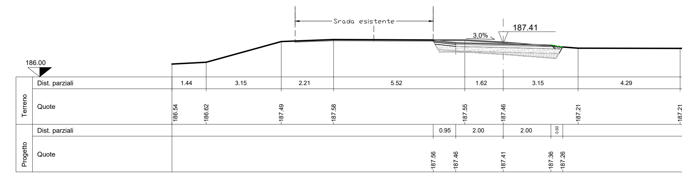
SEZ.NUM. 3 PROGR. 10.00 PARZ. 5.00
