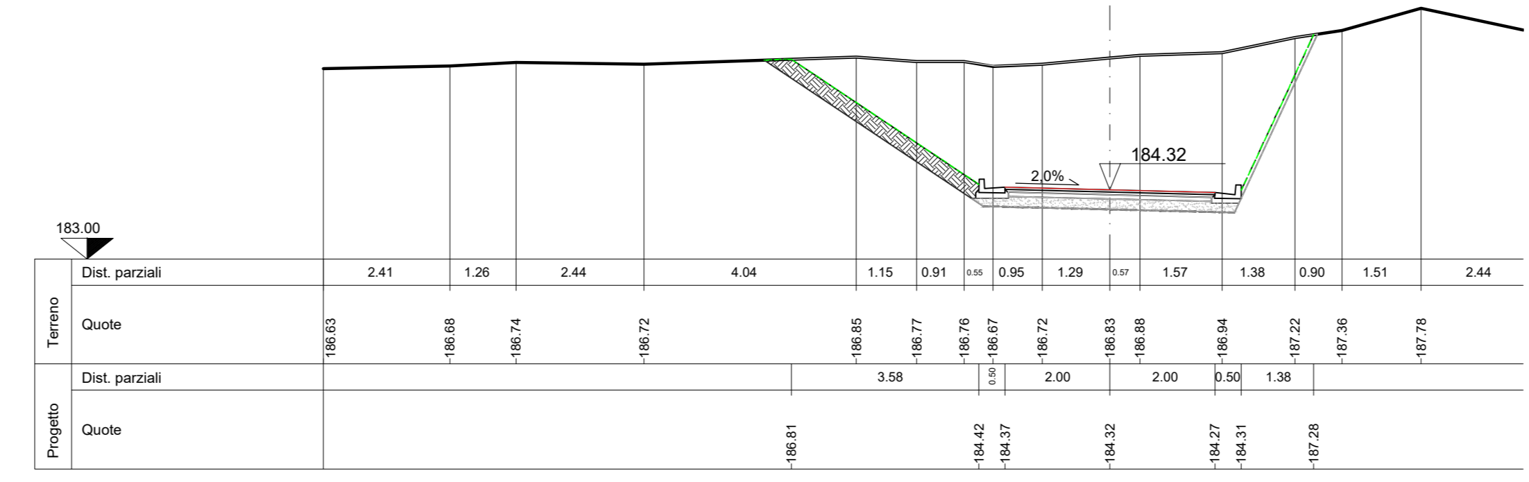
SEZ.NUM. 9 PROGR. 40.00 PARZ. 5.00
