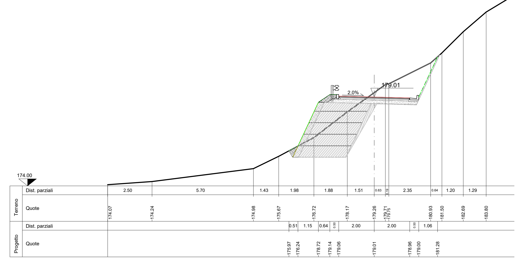
SEZ.NUM. 15 PROGR. 70.00 PARZ. 5.00
