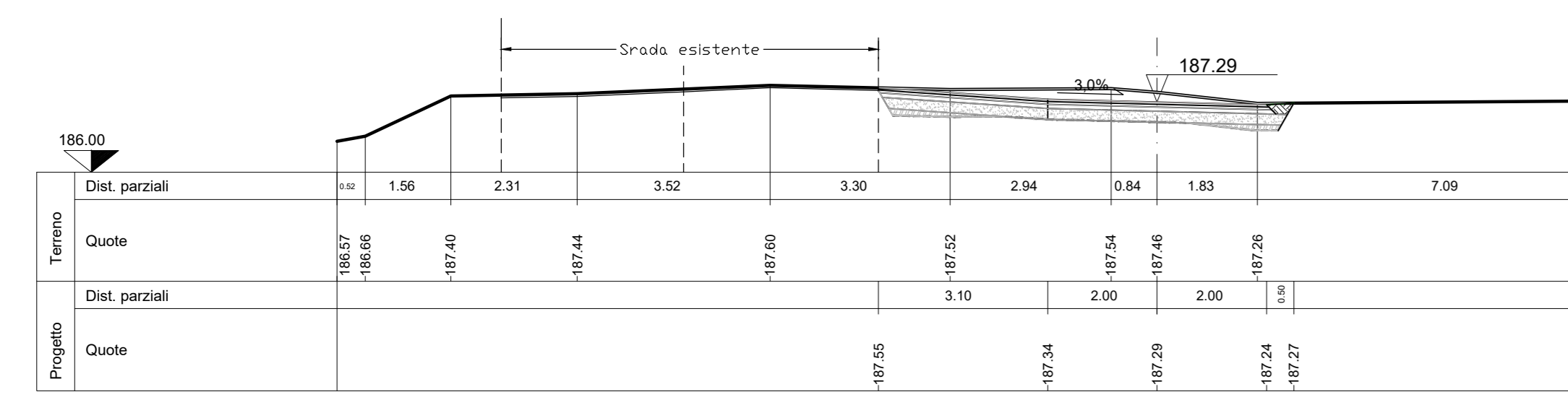
SEZ.NUM. 4 bis PROGR. 16.00 PARZ. 6.00
