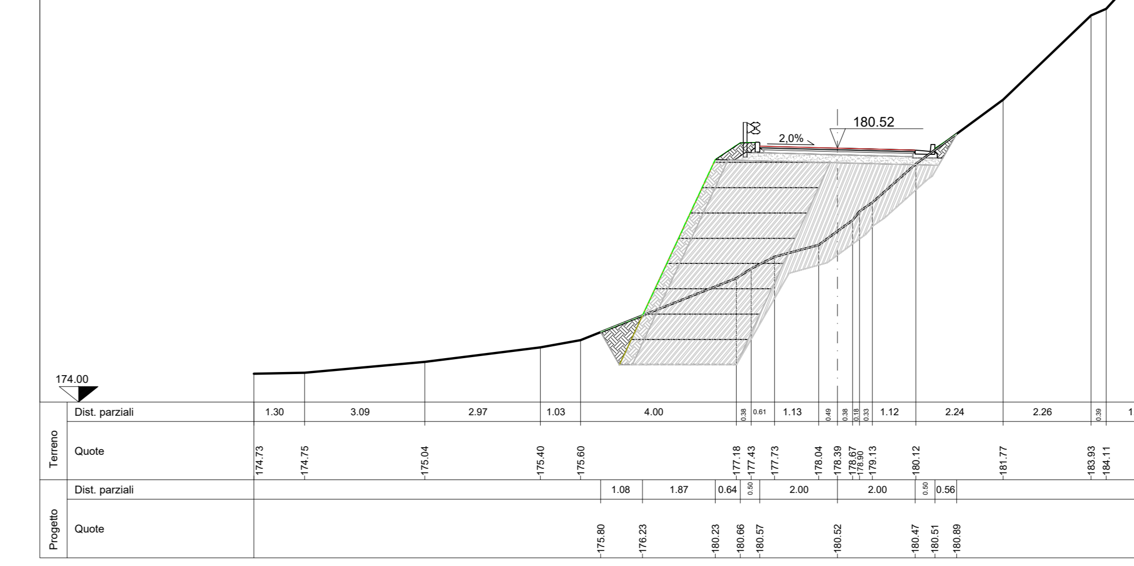
SEZ.NUM. 13 PROGR. 60.00 PARZ. 5.00
