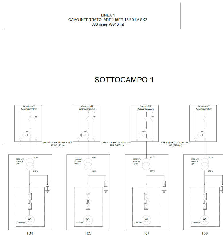
Schema a blocchi del parco eolico GRUPPO 1
