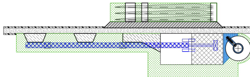
Schemi di piazzole con relative aree di montaggio gru di sollevamento e aree deposito materiali
