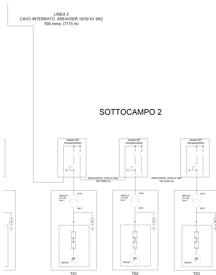
Schema a blocchi del parco eolico GRUPPO 2
