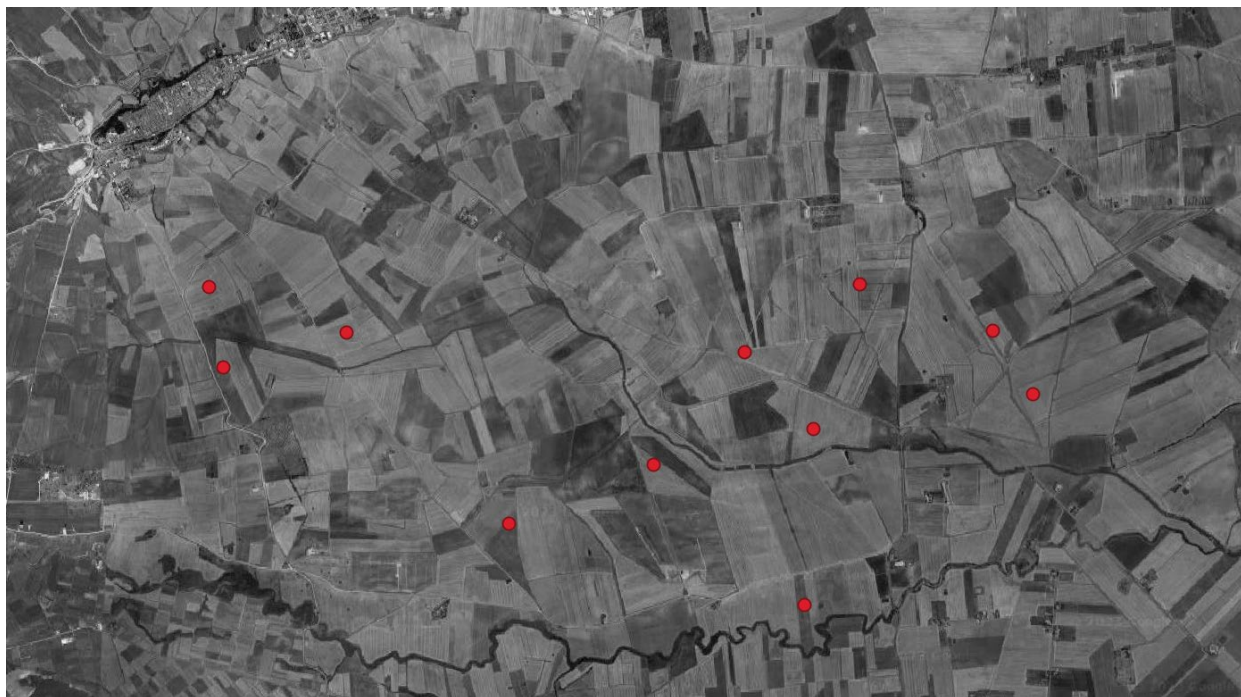
Ipotesi di layout composto da 11 aerogeneratori
