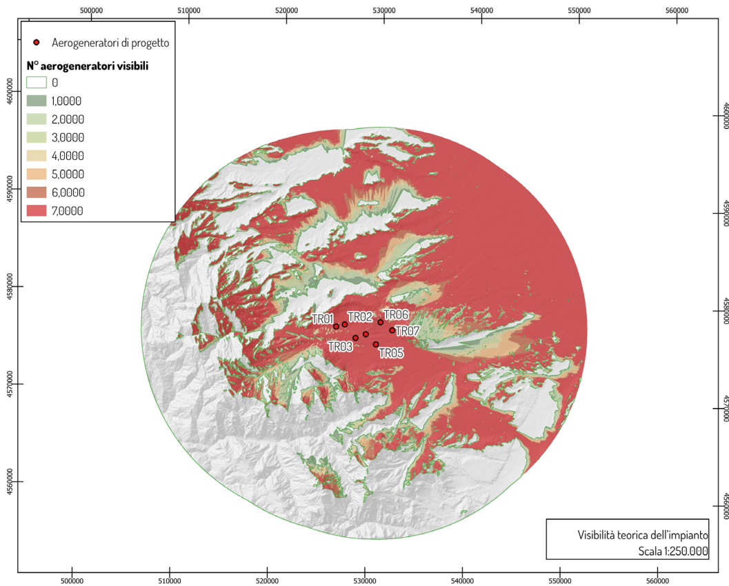
Morfologia del territorio e Visibilità teorica dell'impianto
