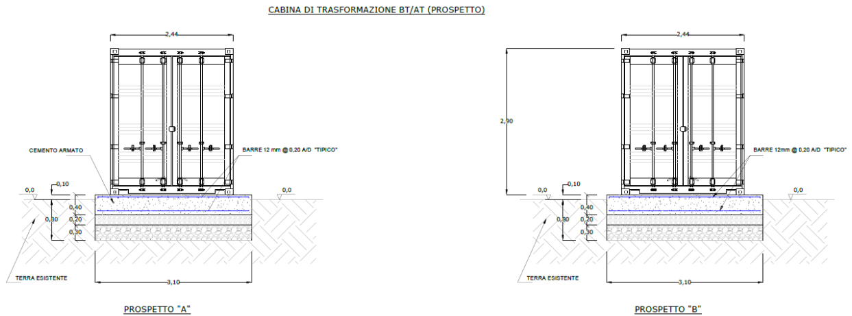
Fig. 19 - Cabina di trasformazione BT/AT
