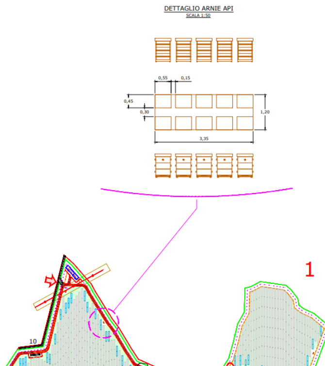
Fig. 4 – Esempio di “area di impianto” agrivoltaico
