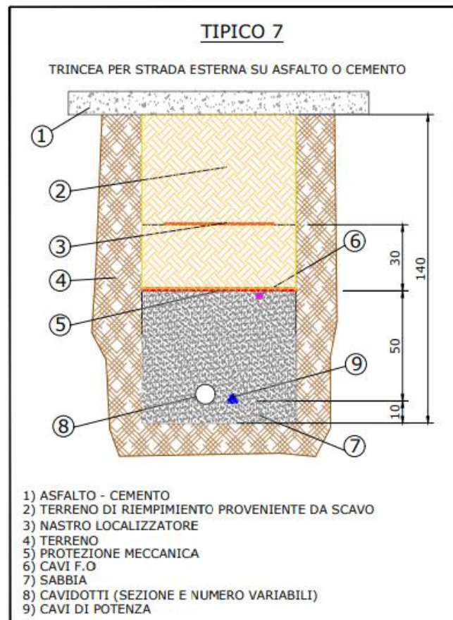
Fig. 18 – Tipici scavi e posa cavi
