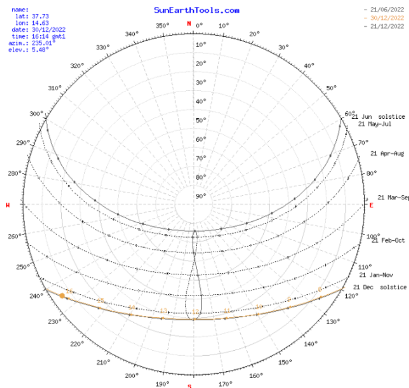
Fig. 25 - Diagramma Solare Polare (Troina)
