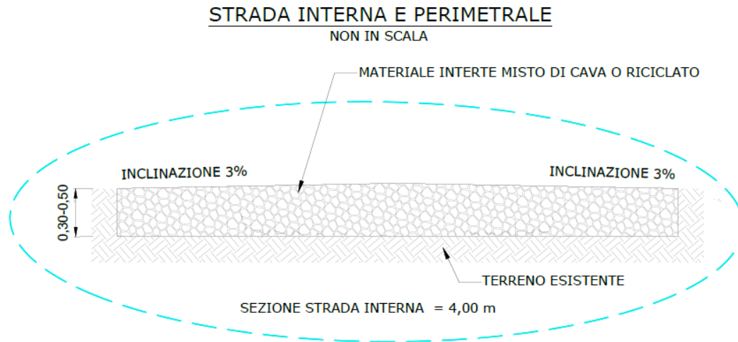
Fig. 18 – Sezione strada perimetrale
