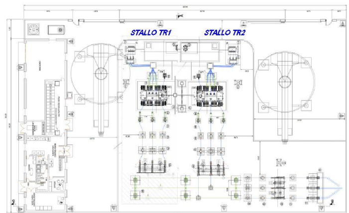
Figura 28 - Rappresentazione schematica stazione di connessione AT
