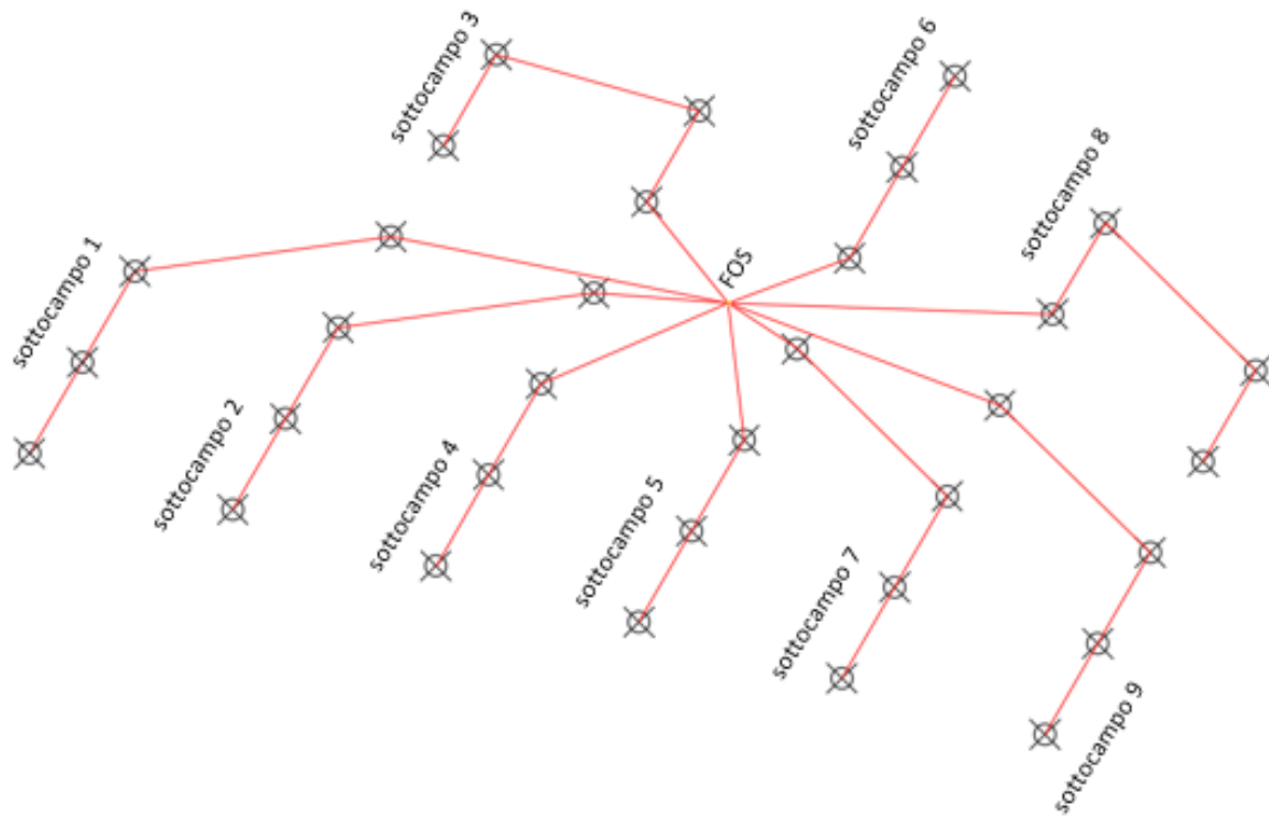
Figura 4 - Struttura del parco eolico con indicazione dei sottocampi e delle stazioni offshore
