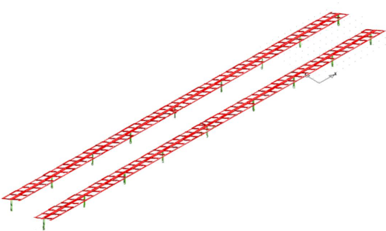
MODELLO TRIDIMENSIONALE
