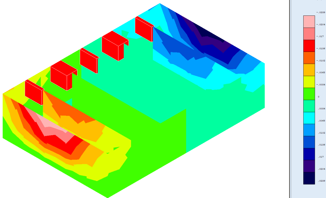
STATO DEFORMATIVO
