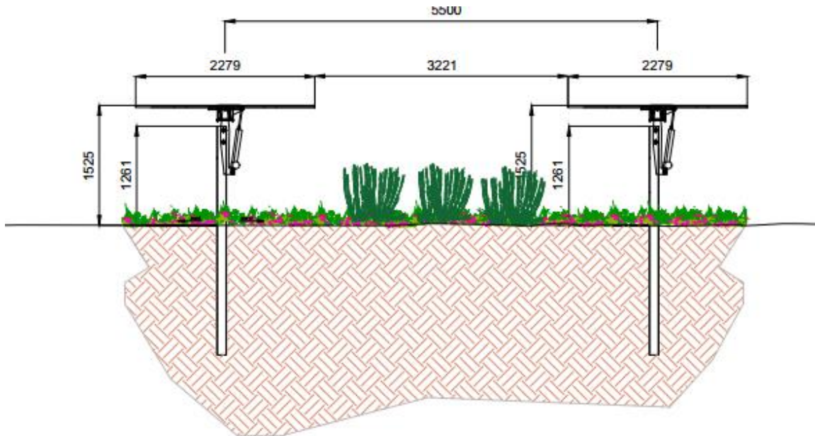
Fig. 2 - Schema della struttura – sezione
