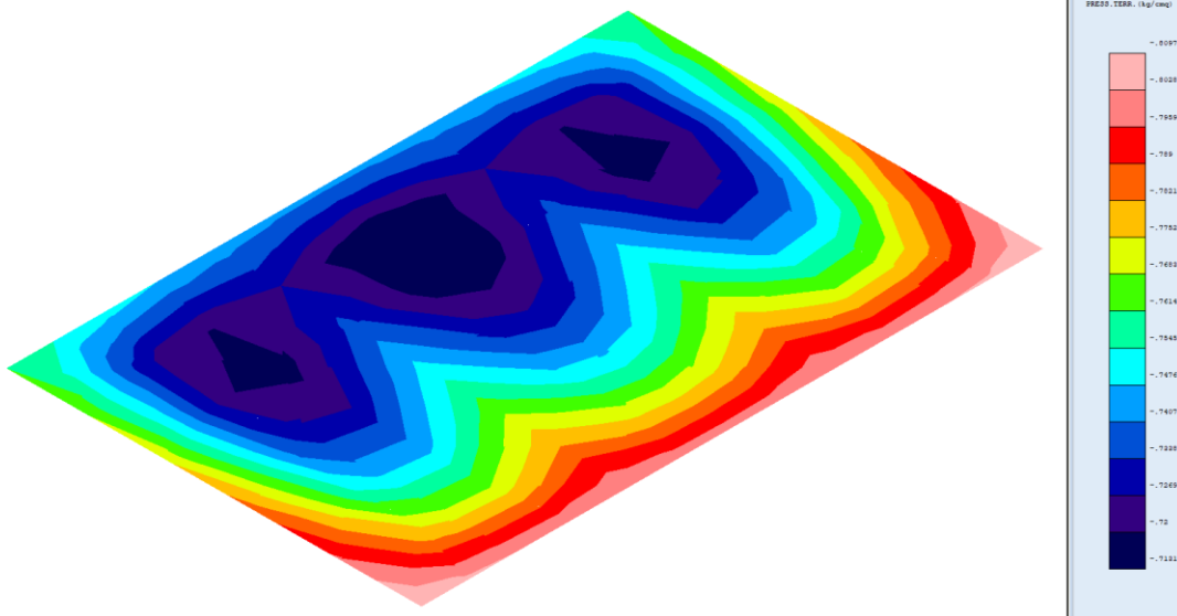
PRESSIONI TERRENO
