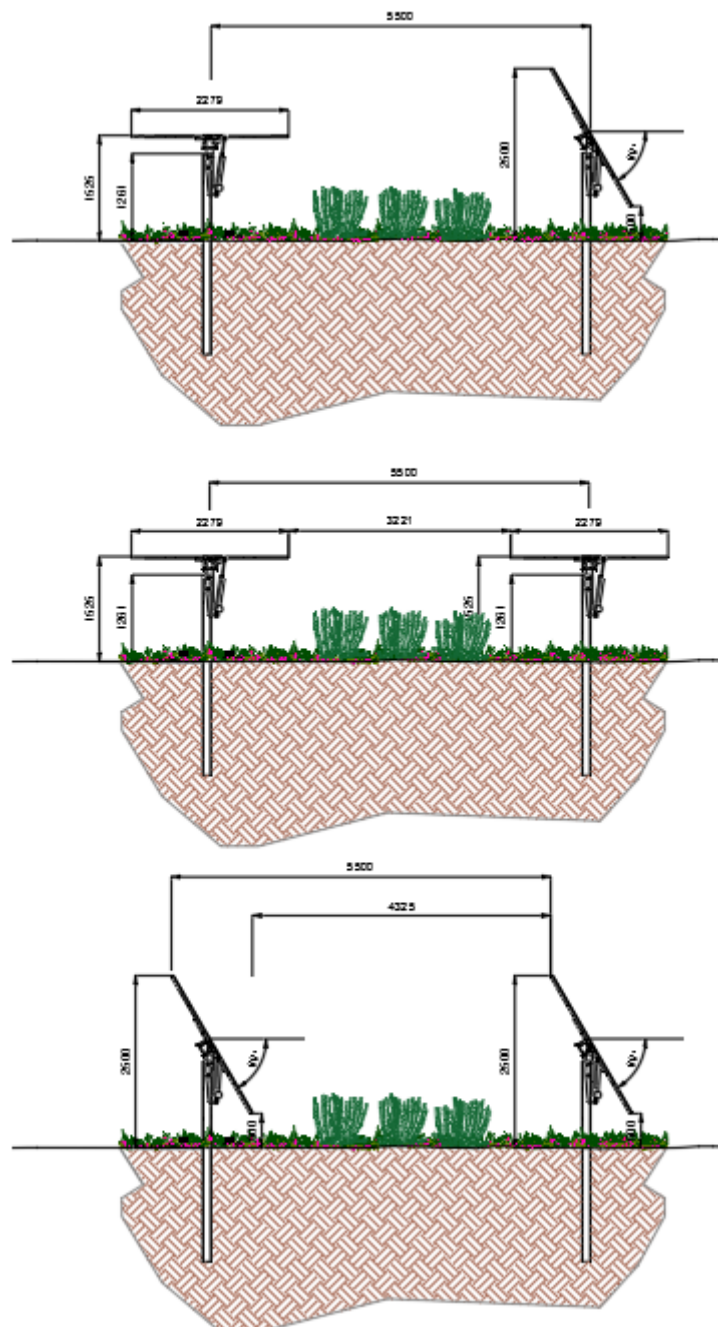
Figura 1 Dettaglio Tracker
