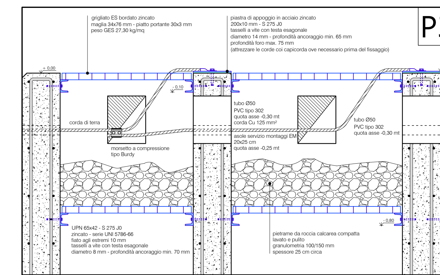
Particolare " 2 " scala 1:10
