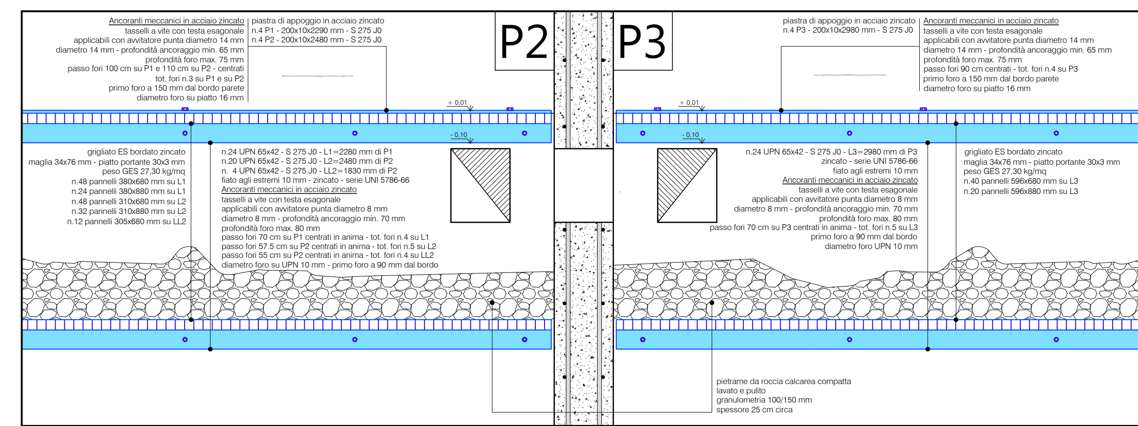
Particolare " 1 " scala 1:10
