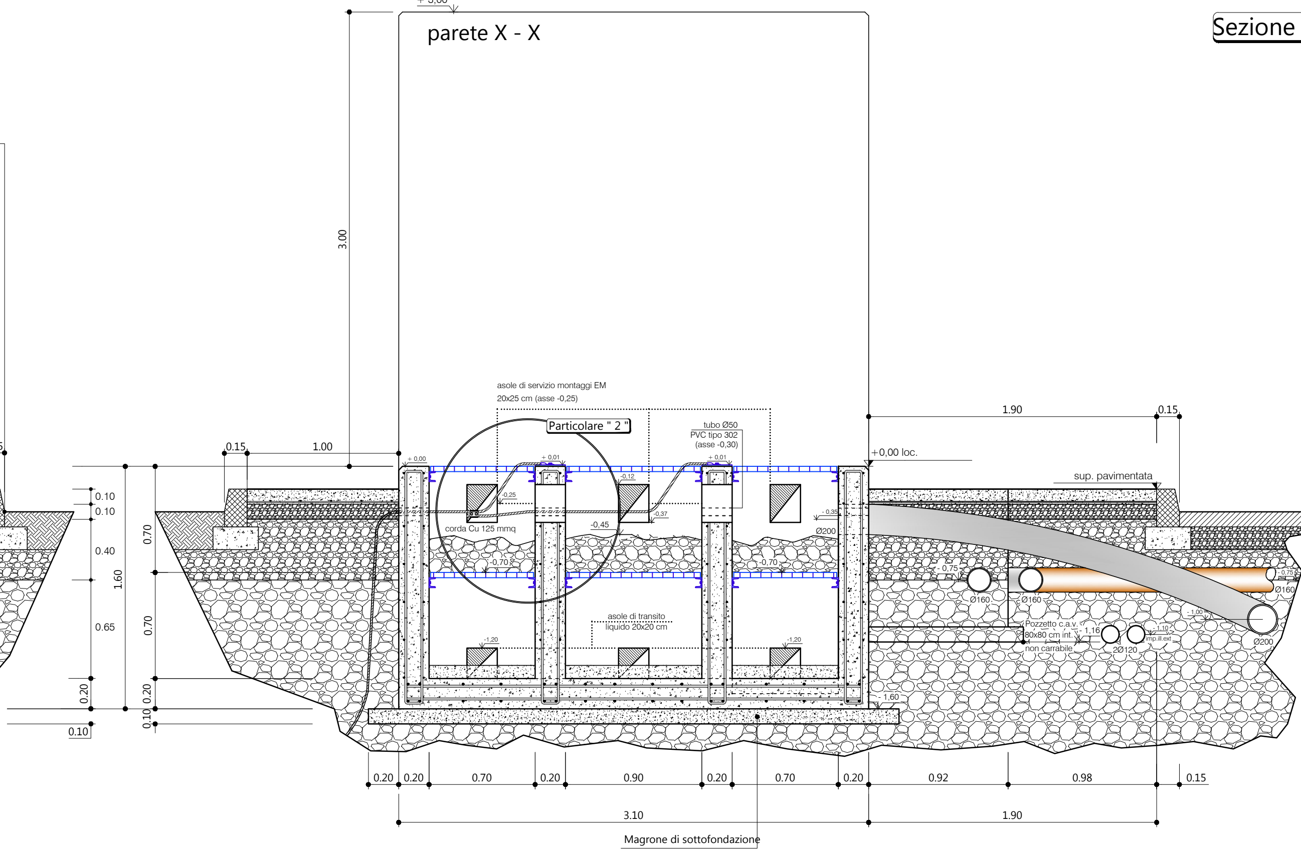
parete X - X
