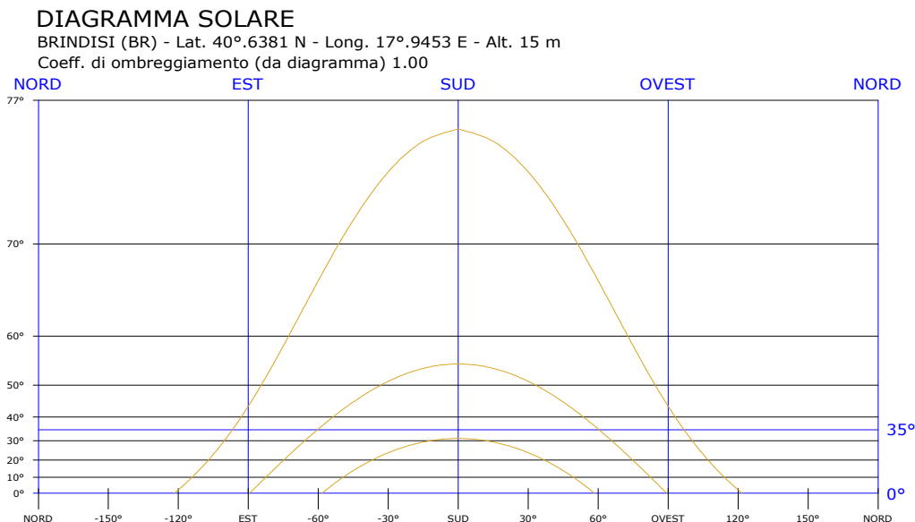
Fig. 2: Diagramma solare
