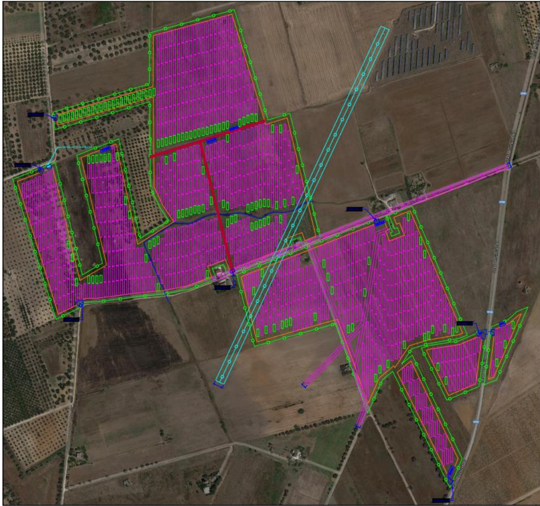
Fig. 2: Inquadramento Ortofoto
