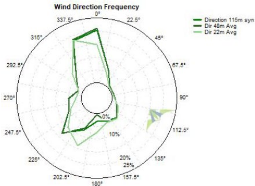
Figura 7-1: Frequenza della direzione del vento per la torre anemometrica "Gangi"
