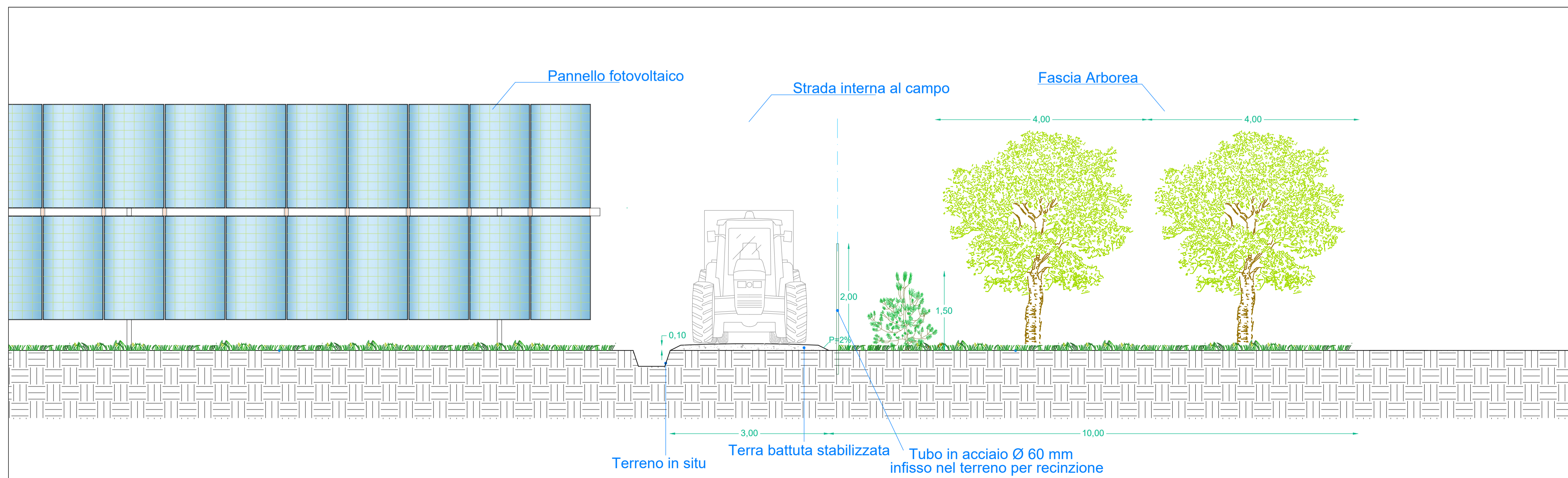
SEZIONE FASCIA ARBOREA 10 m - scala 1:50
