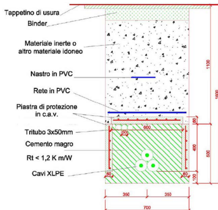
Figura 65 Sezione tipo di posa dei cavi elettrici
