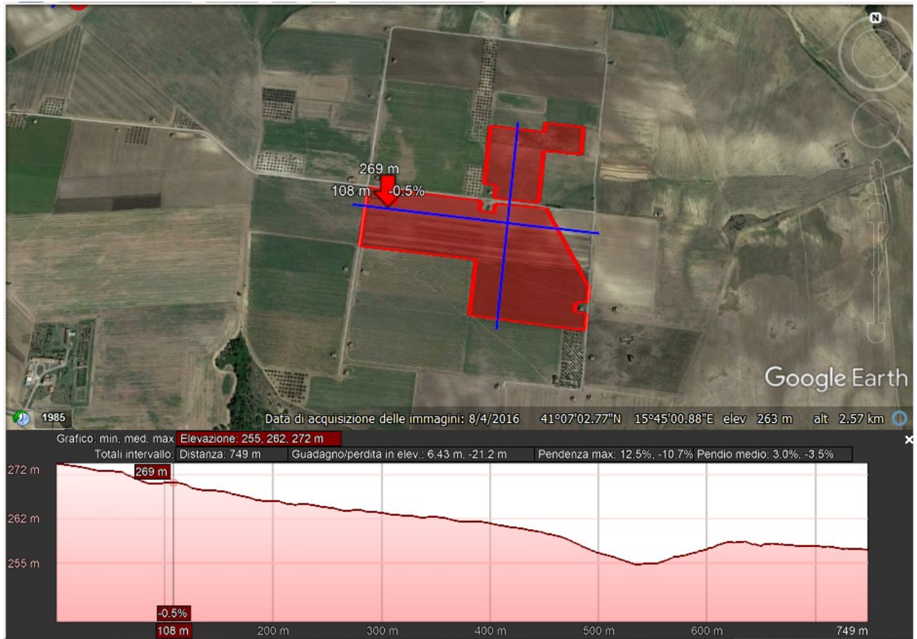
Figura 31 Profili altimetrici
