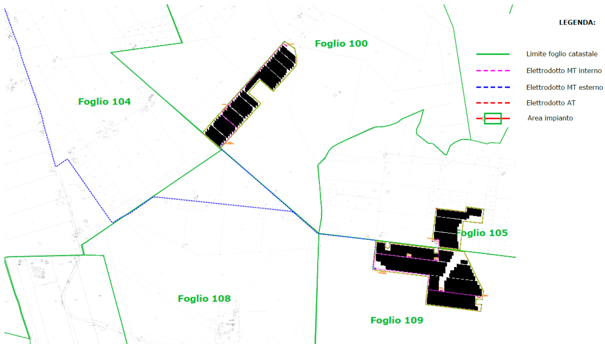
Figura 26 Stralcio elaborato DEF-TAV.06 – Layout su catastale
