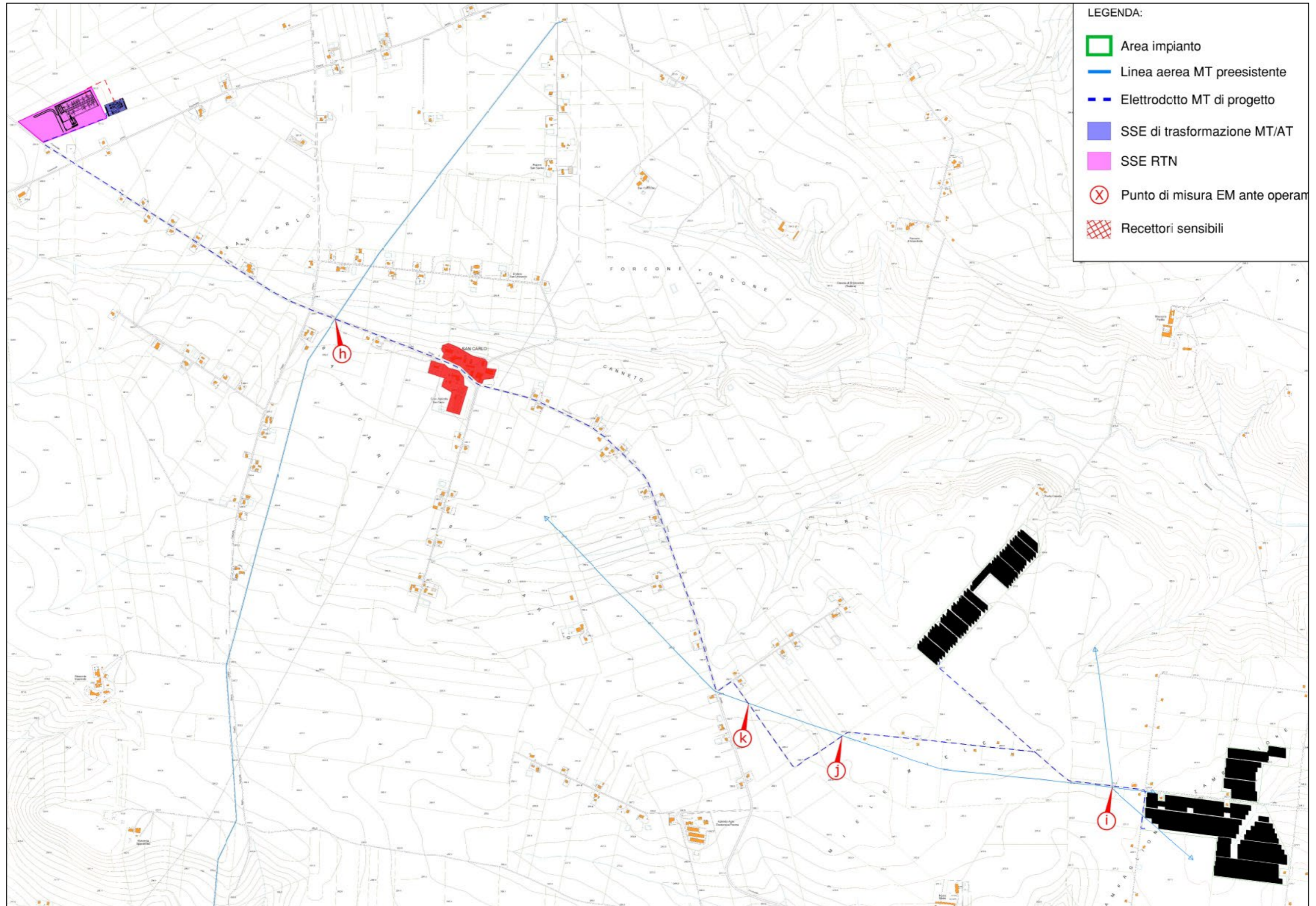
Figura 55 Stralcio planimetrico con rappresentazione del tracciato dell'elettrodotto MT di progetto.
