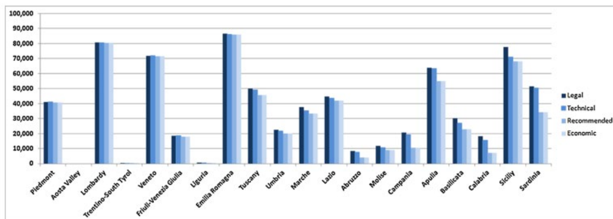
Figura 60 Schema tabellare e grafico da cui si evincono le potenziali superfici disponibili per la realizzazione del fotovoltaico e l'energia potenziale suddivisi per regioni
