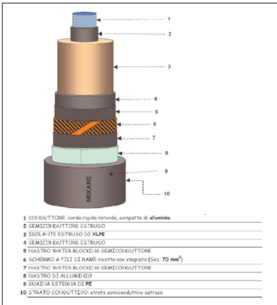
Figura 40 – Schema tipologico del cavo
