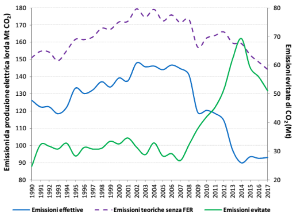
Figura 47 Andamento delle emissioni effettive per la produzione lorda di energia elettrica e delle emissioni teoriche per la produzione di energia elettrica da fonti rinnovabili con equivalente produzione da fonti fossili.
