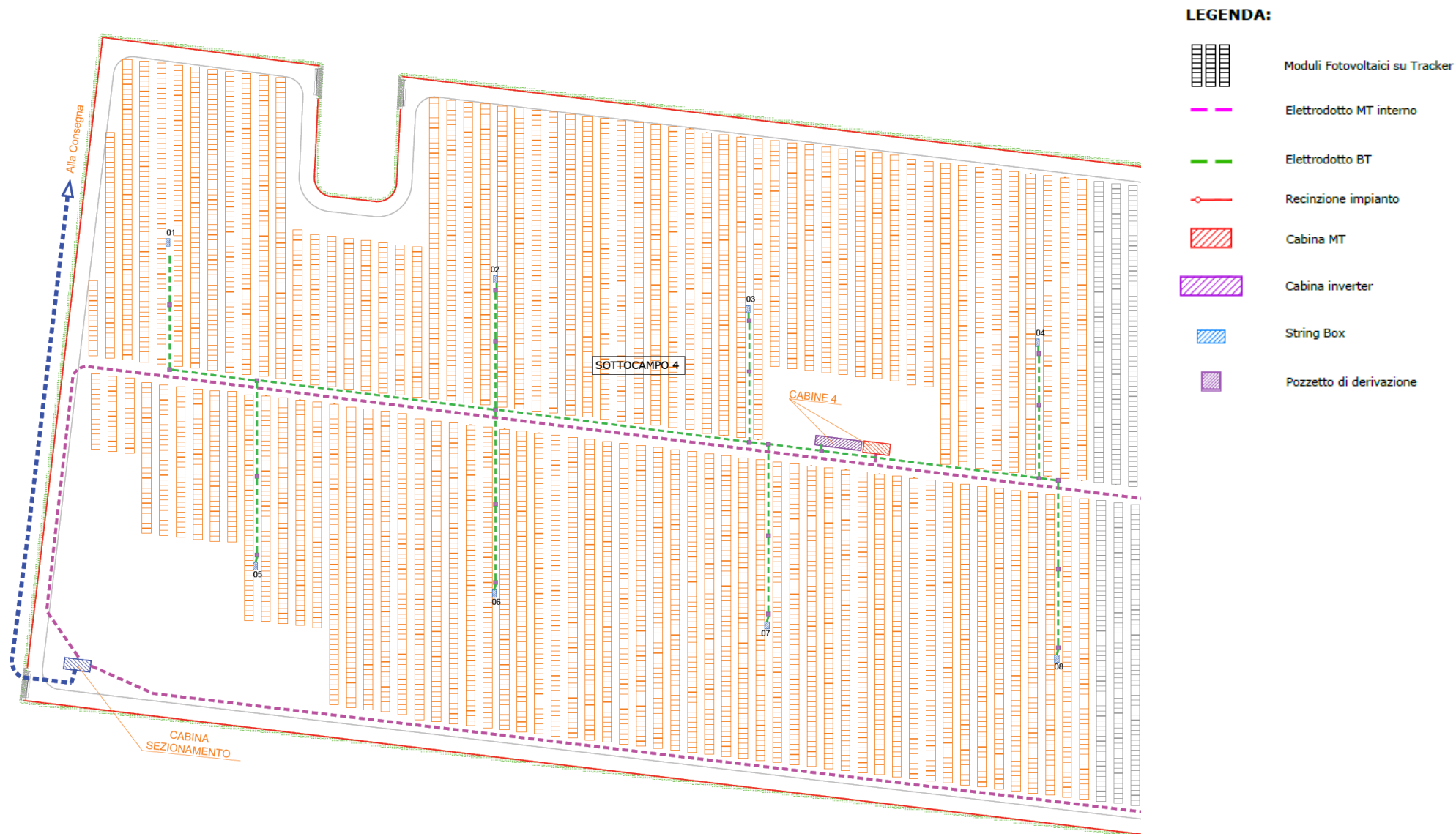
Figura 30 Stralcio elaborato DEF-TAV.12 – Particolare sottocampo
