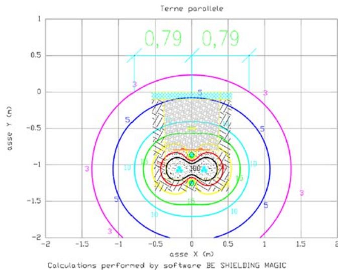
Fig. 32-33 – Livelli di campo magnetico per il cavidotto MT 30kV 14.3.5.2 CALCOLO DEL CAMPO MAGNETICO – CABINA UTENTE
