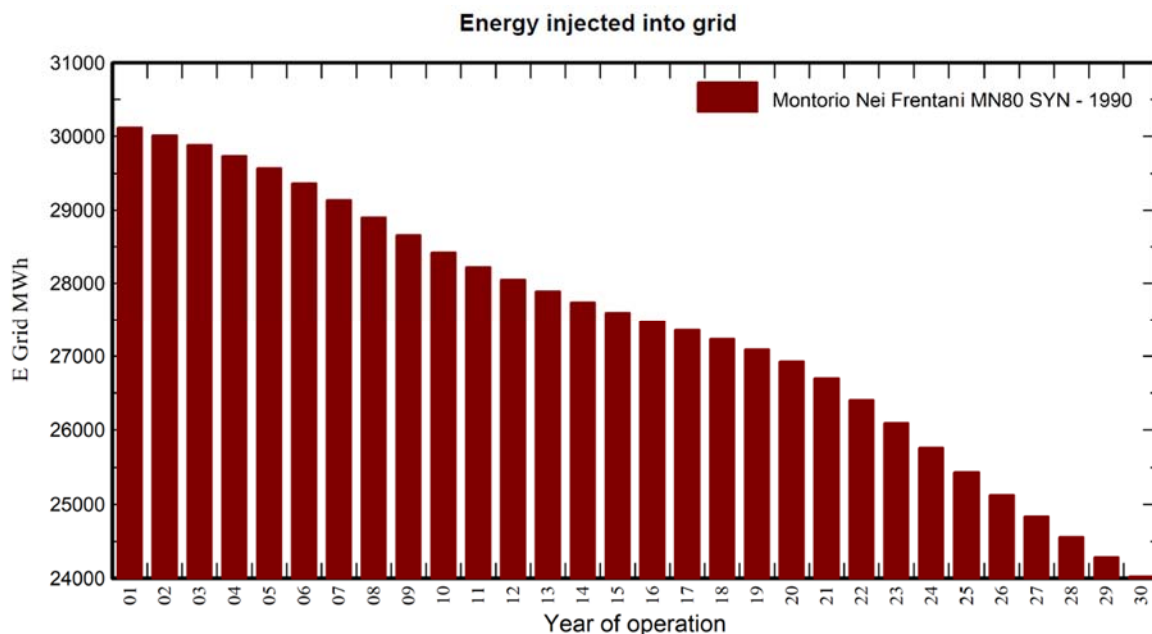
Fig. 23-24 – Producibilità dell’impianto con degrado moduli (30 anni)
