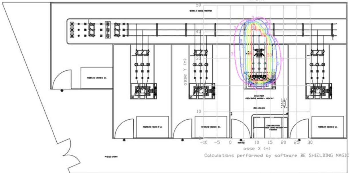
Fig. 38-39 – Calcolo dei livelli di campo magnetico a 5 m da terra
