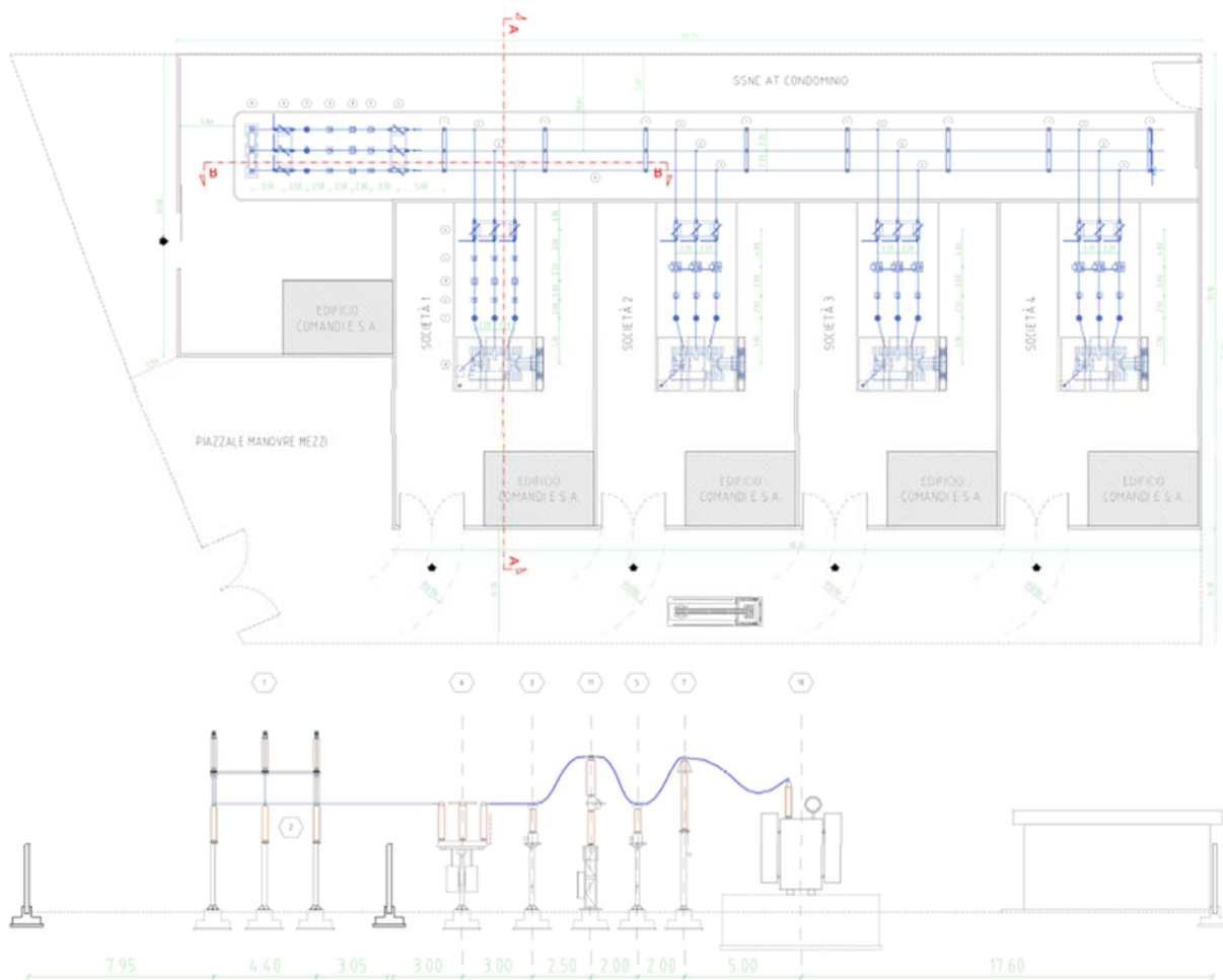
Fig. 45-16 – Stralcio planimetria e sezione elettromeccanica stallo utente – Rappresentazione non in scala
