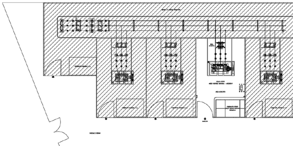
Fig. 33-34 – Planimetria della cabina utente (senza retino), all'interno del Punto di Raccolta (con retino)
