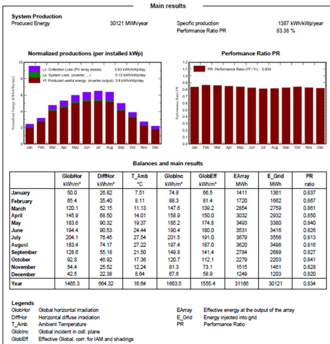
Fig. 22-23 - Risultati di calcolo (Fonte: PVsyst - Meteonorm)
