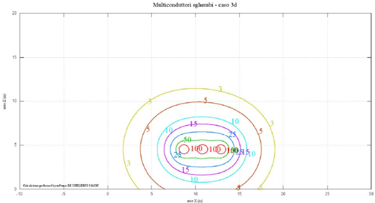
Fig. 36-37 – Livelli di campo magnetico sullo stallo AT
