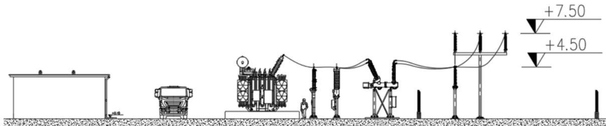
Fig. 34-35 – Sezione della cabina utente e Sbarra AT comune con individuazione delle altezze
