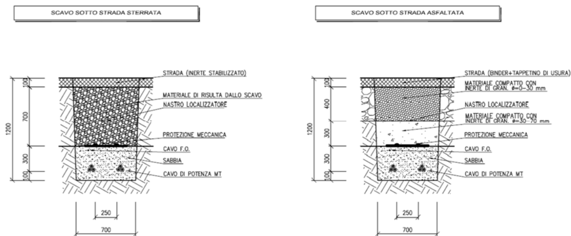
Fig. 11-12 – Posa cavi interrati
