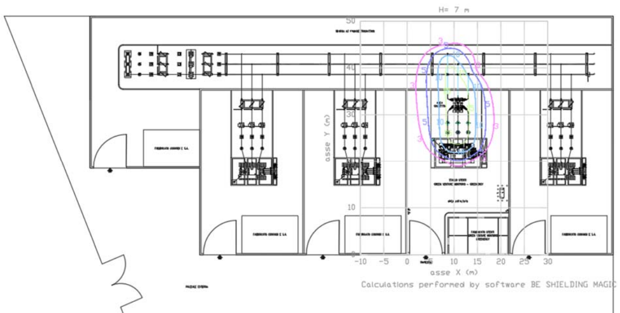
Fig. 39-40 – Calcolo dei livelli di campo magnetico a 7 m da terra
