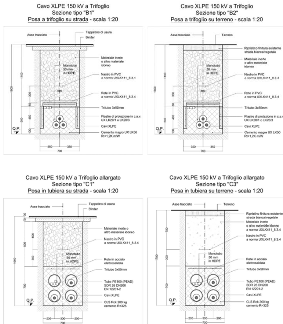
Fig. 46-17 – Modalità di posa
