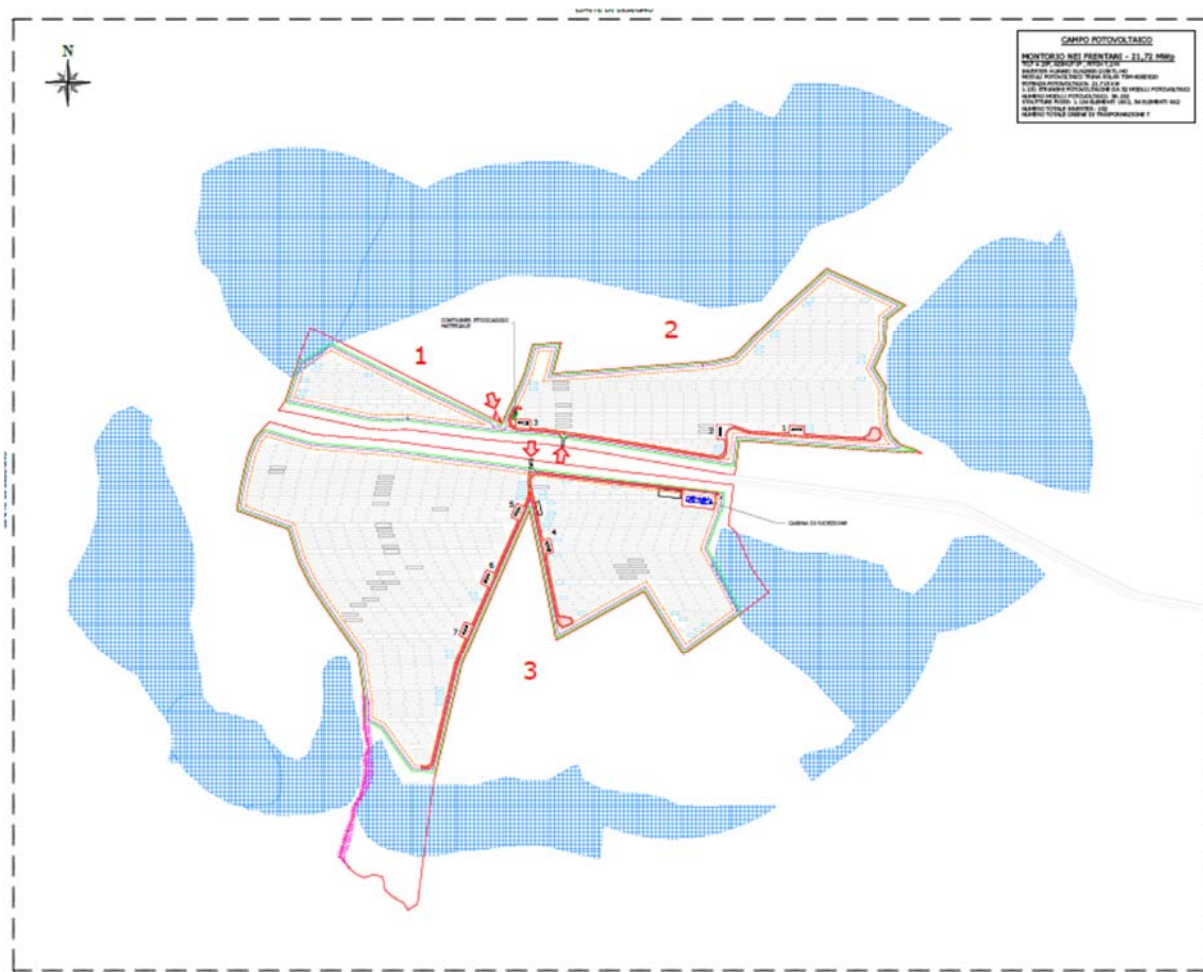
Fig. 9-10 - Layout di impianto
