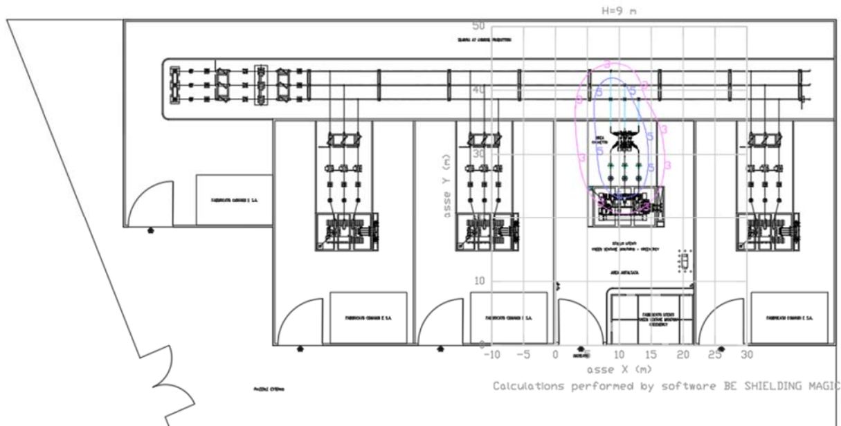
Fig. 40-41 – Calcolo dei livelli di campo magnetico a 9 m da terra
