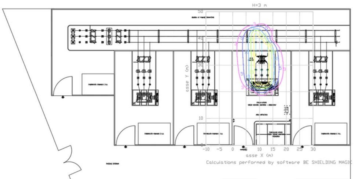
Fig. 37-38 – Calcolo dei livelli di campo magnetico a 3 m da terra
