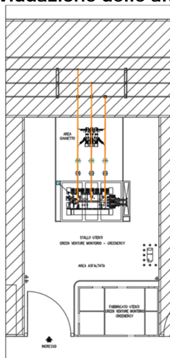
Fig. 35-36 – Planimetria della cabina utente con individuazione degli elementi attivi
