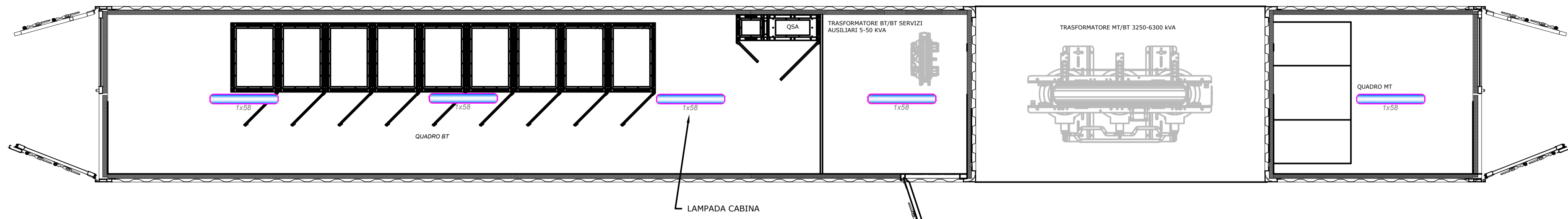
CABINA DI TRASFORMAZIONE BT/MT (VISTA IN PIANTA)
