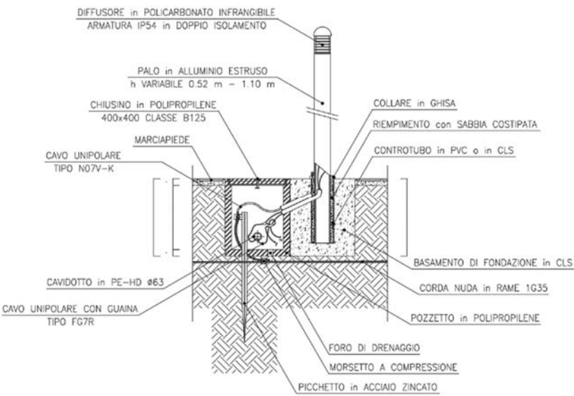
Fig. 3 - Tipologia di corpi illuminanti nei pressi delle cabine
