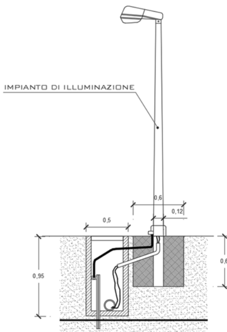
Fig. 2 - Tipologia di corpi illuminanti - perimetro impianto
