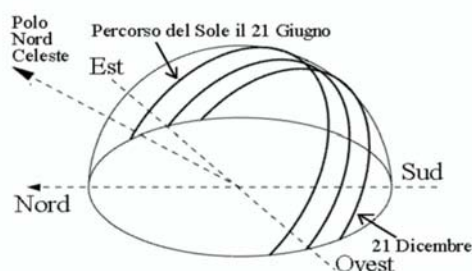
Fig. 4 - Movimento apparente del disco solare per un osservatore situato ad una latitudine nord attorno ai 45°. Per tutte le località situate tra il Tropico del Cancro e il Polo Nord Geografico il disco solare non raggiunge mai lo zenit.
