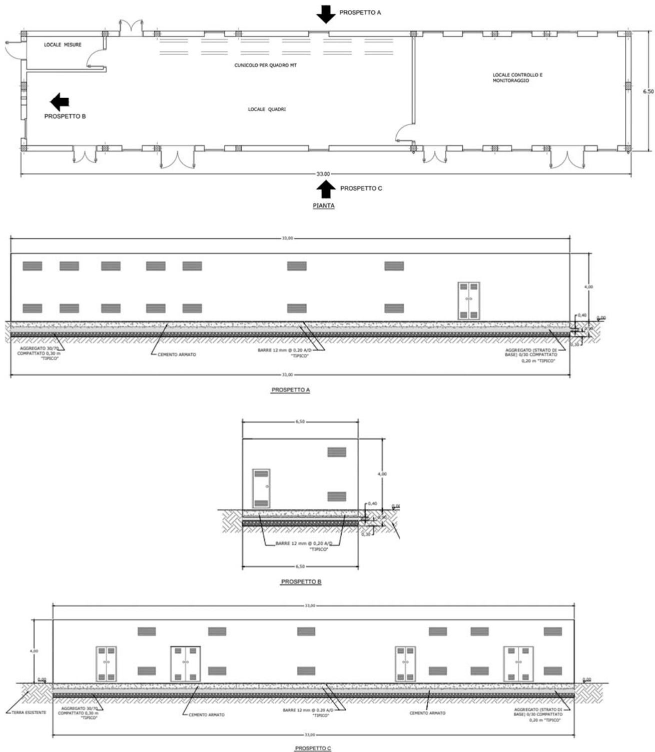
Fig. 15 - Cabina di ricezione
