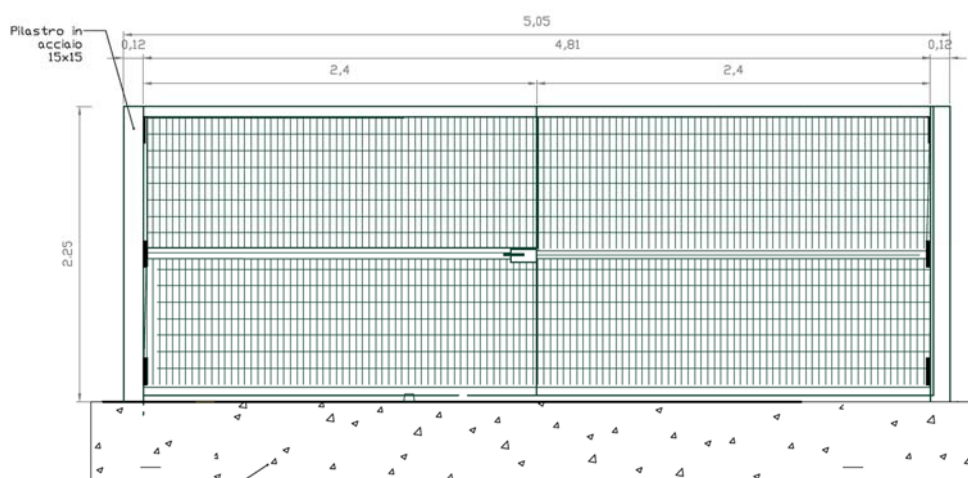
Fig. 19 – Cancello carrabile
