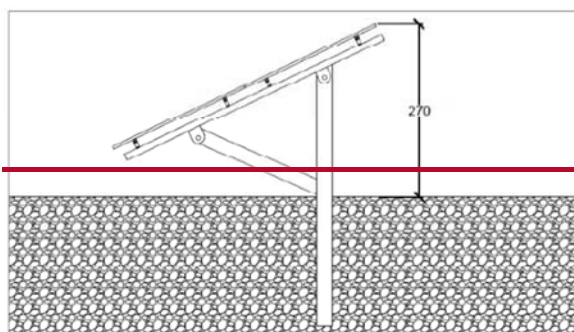
STRUTTURA DI SOSTEGNO MONOPALO
