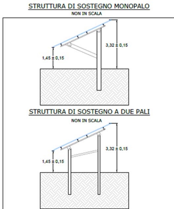
Fig. 2 - Struttura di supporto moduli
