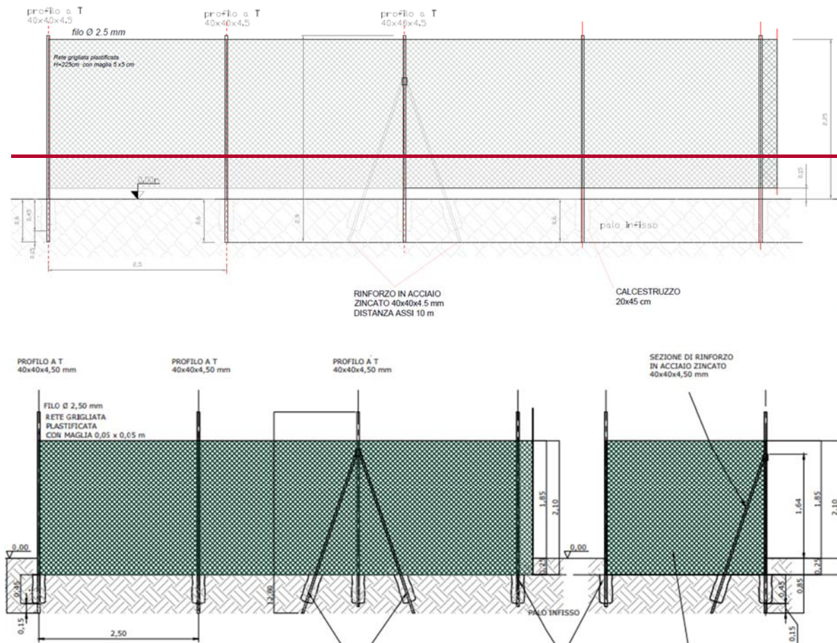
Fig. 18 – Particolare della recinzione
