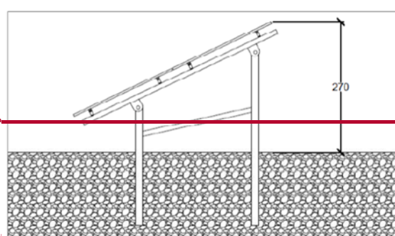
STRUTTURA DI SOSTEGNO A DUE PALI
