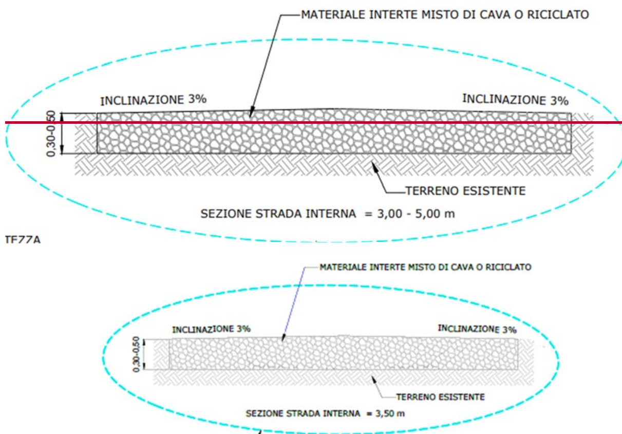
Fig. 20 – Sezione strada perimetrale
