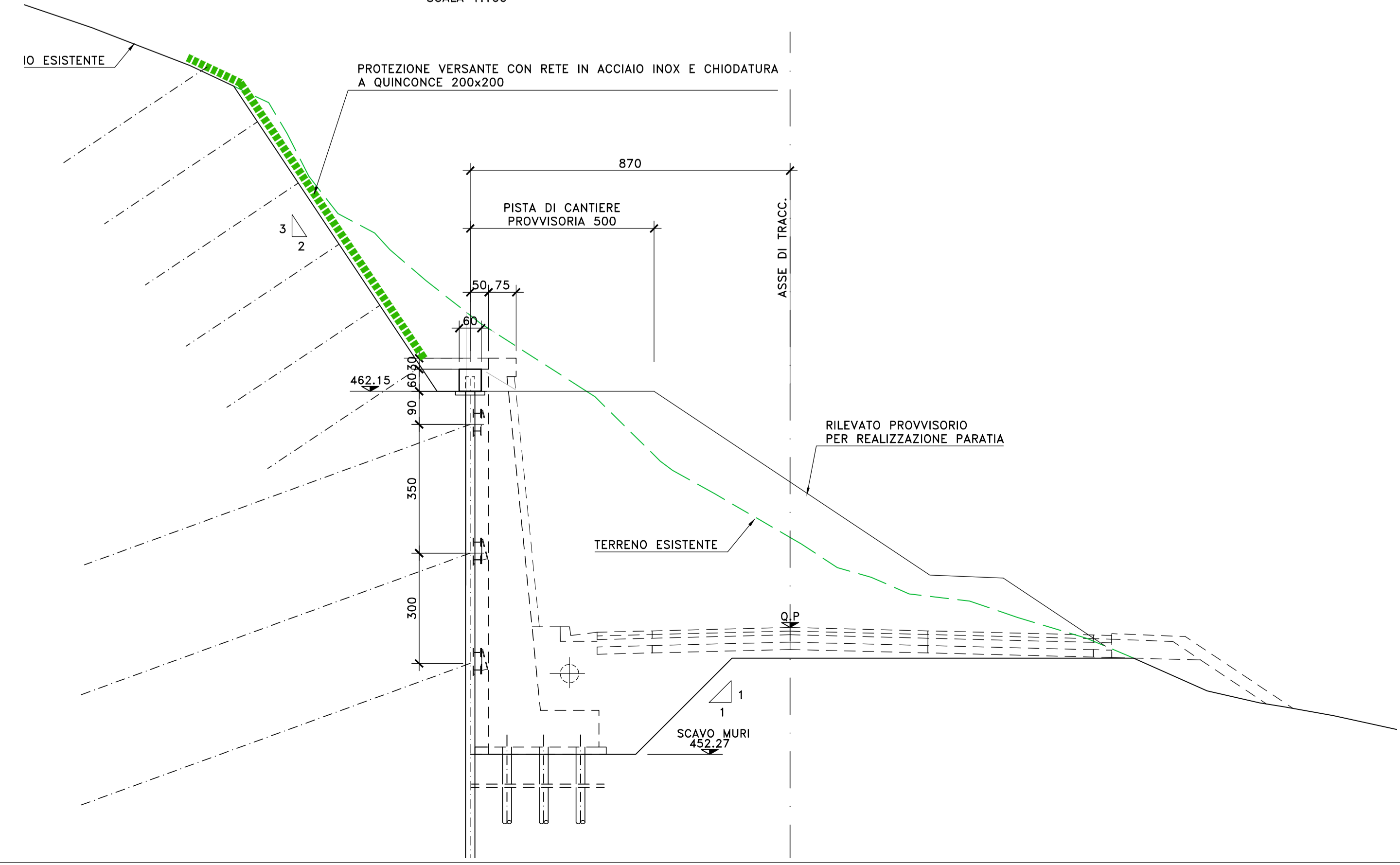
SEZIONE N.442 PR 9+140.00 SCALA 1:100
