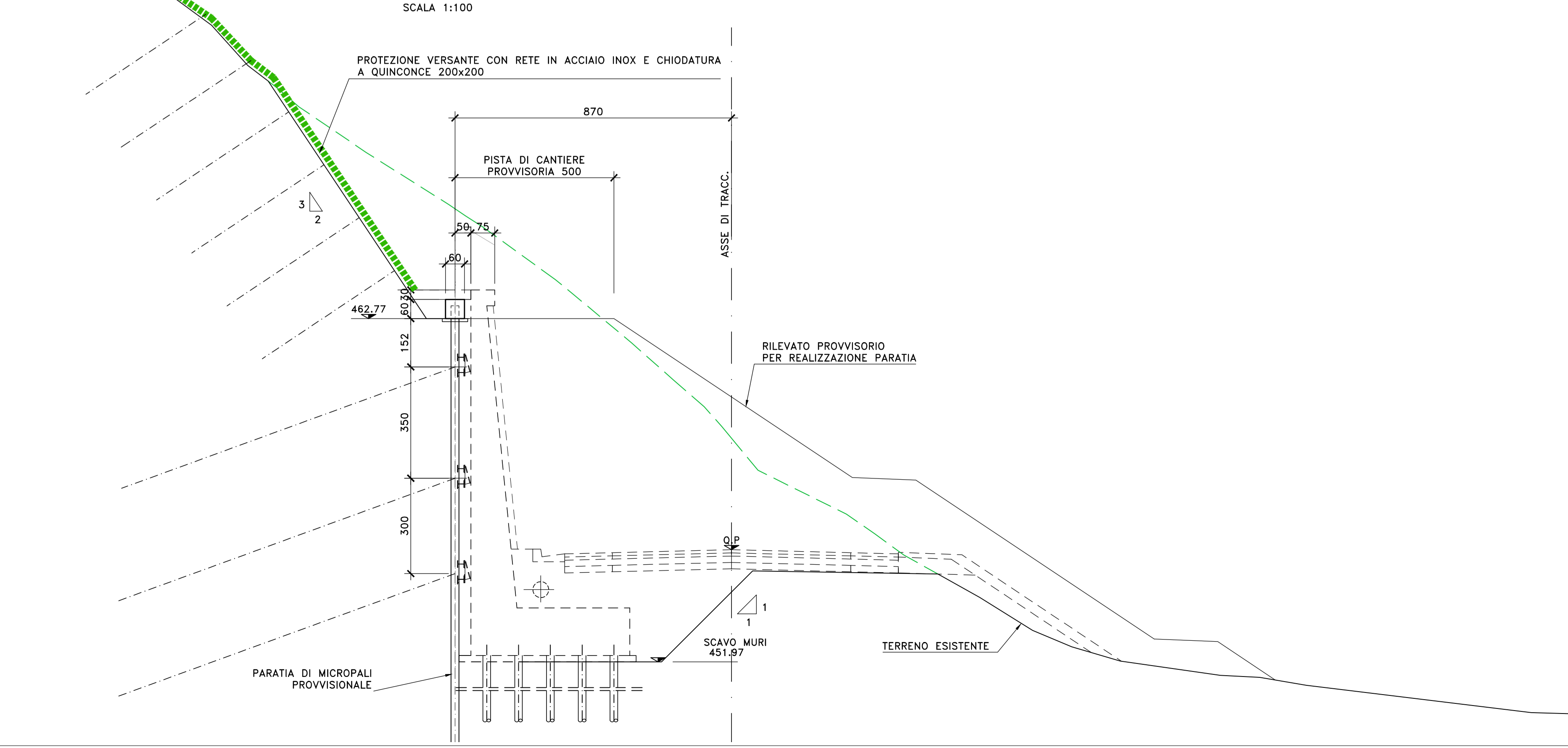
SEZIONE N.441 PR 9+120.00 SCALA 1:100
