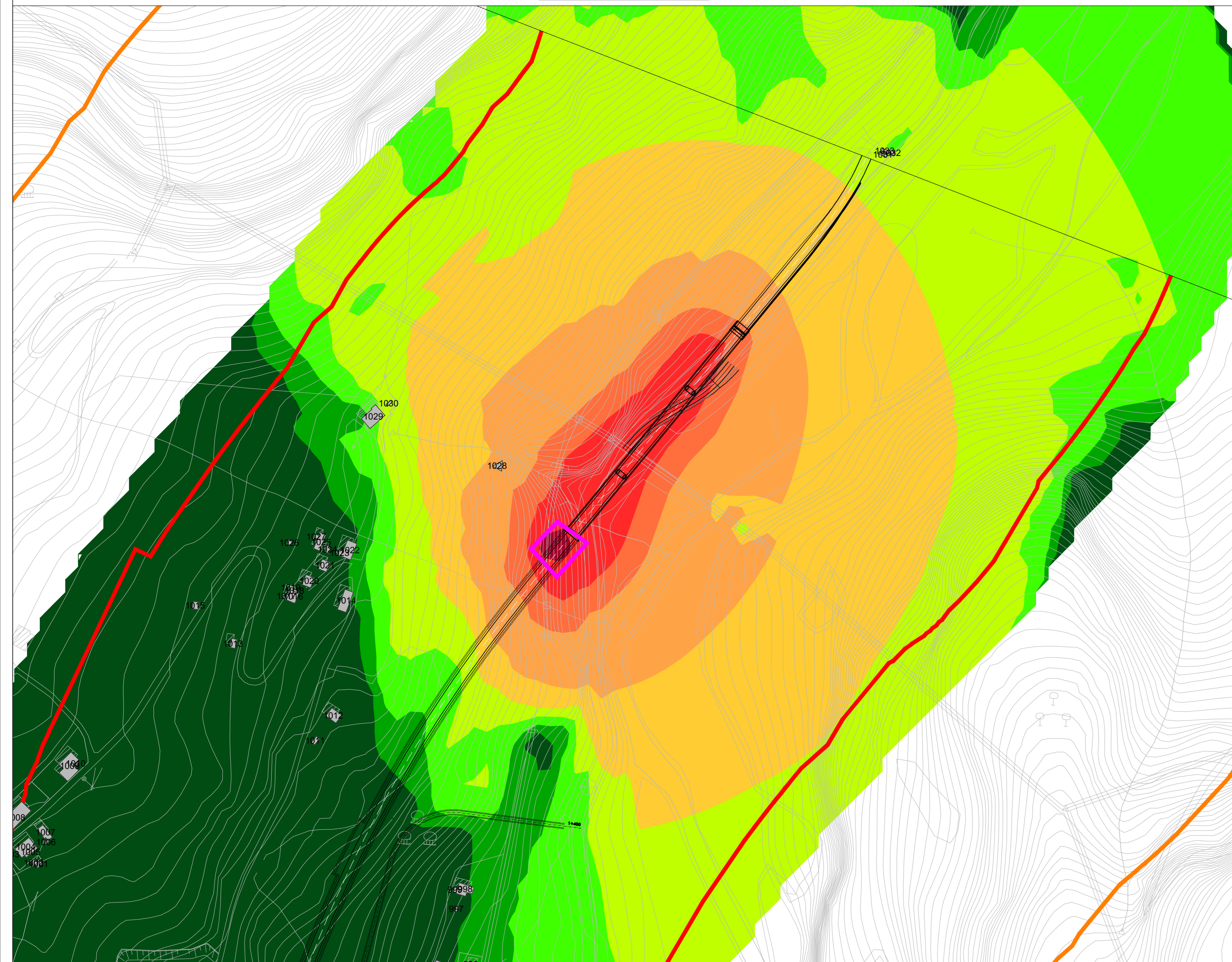
SIMULAZIONE ACUSTICA DEL CANTIERE LUNGOLINEA TIPOLOGICO GALLERIA
