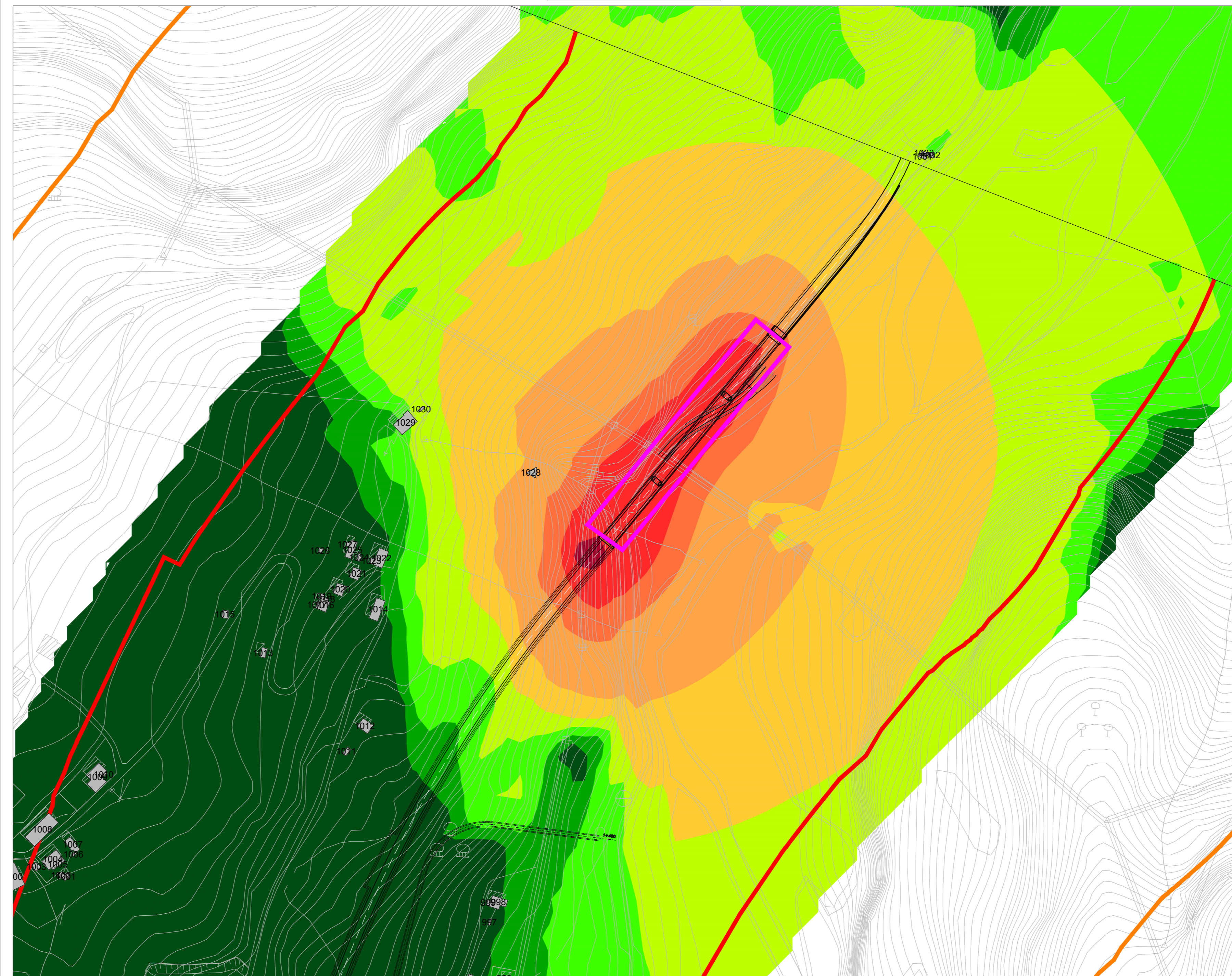
SIMULAZIONE ACUSTICA DEL CANTIERE LUNGOLINEA TIPOLOGICO VIADOTTO
