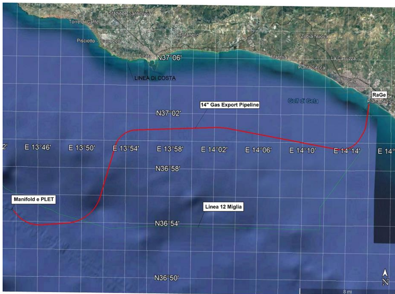
Figura 3-6: Planimetria di progetto
