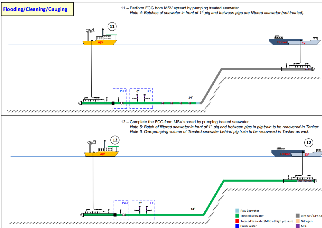
Figura 3-1: Fase 1 - Riempimento / Pulizia /Controllo Ovalità (1 di 2) (In inglese sono descritte le azioni sopra descritte per la Fase 1)
