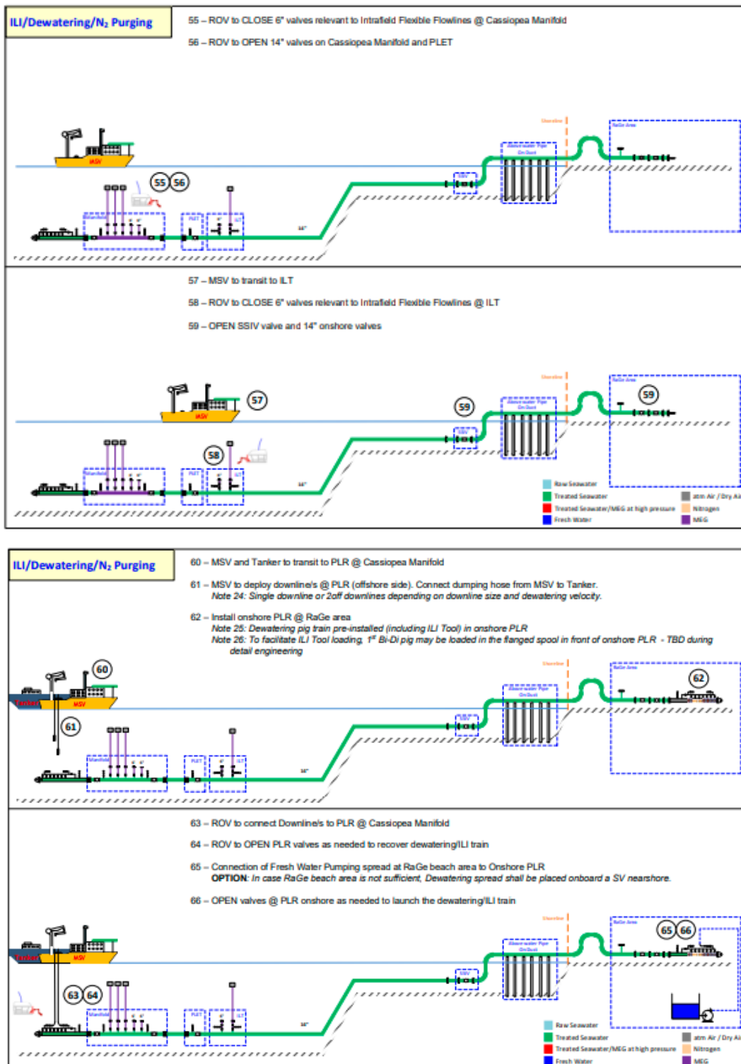
Figura 3-5: Fase 2 – Piggaggio intelligente + Svotamento ed Inertizzazione Condotta (In inglese sono descrizione le azioni sopra descritte per la Fase 2)
