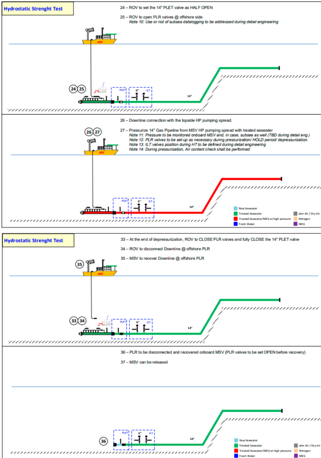
Figura 3-3: Fase 1 – Test in pressione (In inglese sono descritte le azioni sopra descritte per la Fase 1)
