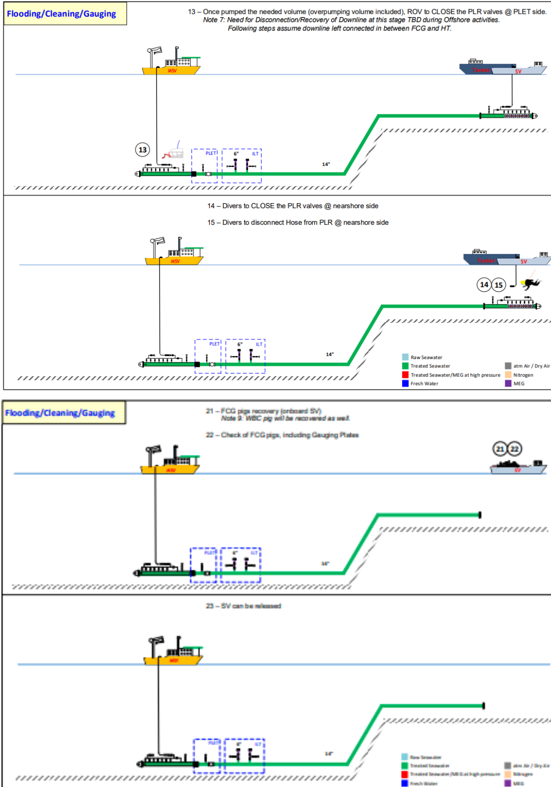
Figura 3-2: Fase 1 - Riempimento / Pulizia /Controllo Ovalità (2 di 2) (In inglese sono descritte le azioni sopra descritte per la Fase 1)
