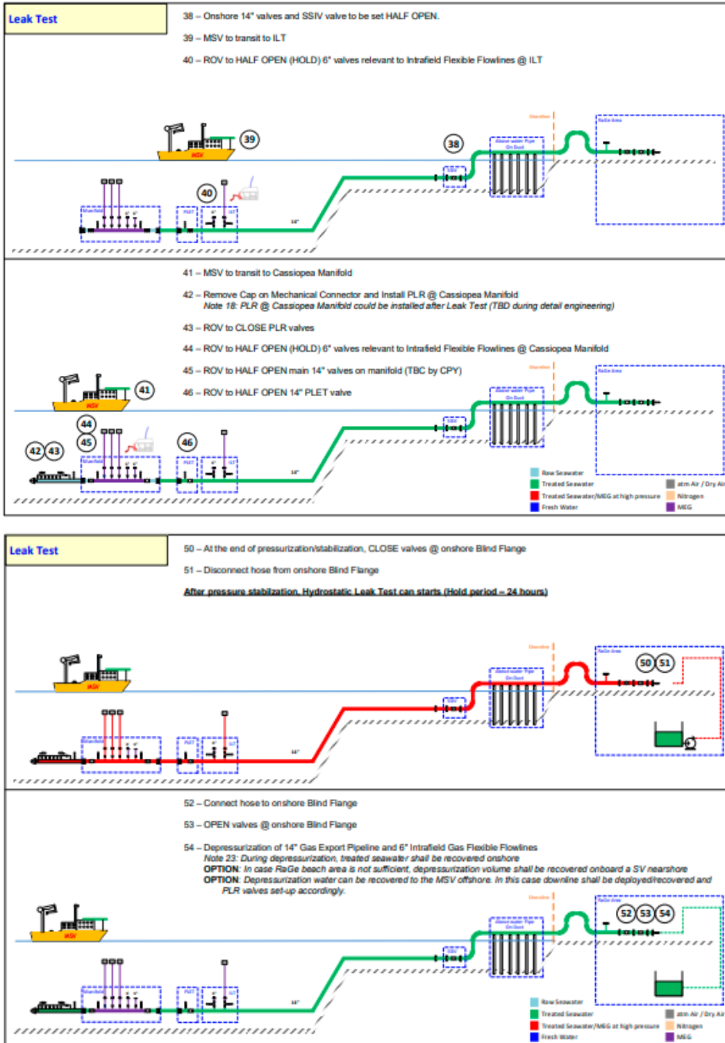
Figura 3-4: Fase 2 – Test di tenuta in pressione (In inglese sono descrizione le azioni sopra descritte per la Fase 2)
