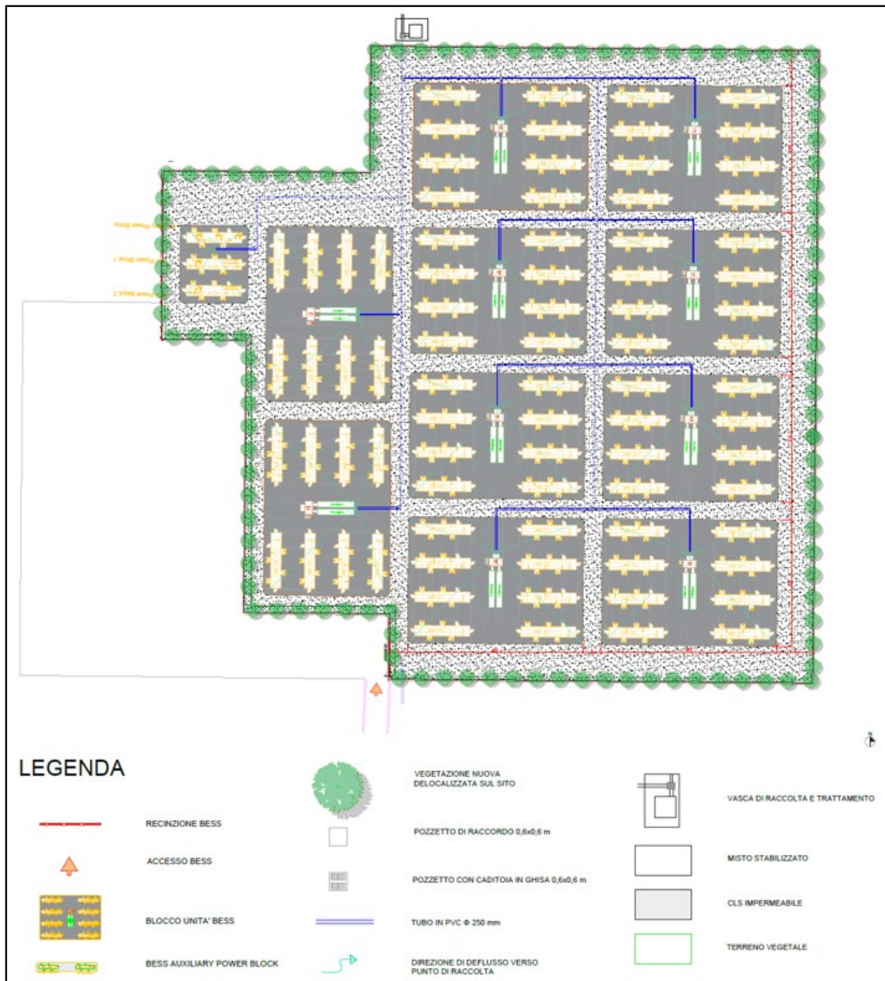
Figura 11.1: Planimetria architettonica BESS con sistema di smaltimento acque (maggiori dettagli sono riportati nell'elaborato di progetto "TSOE099 Planimetria BESS - Impianto raccolta acque meteoriche e di funzionamento")
