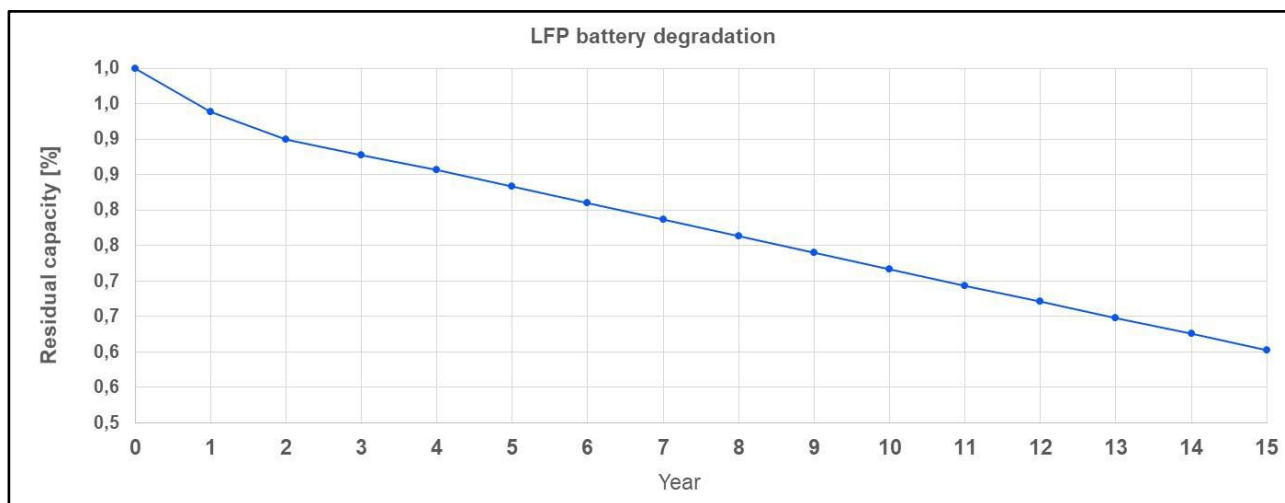
Figura 12.1: Decadimento tecnico del sistema di accumulo (BESS)
