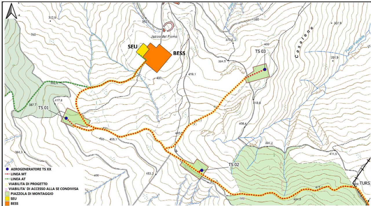
Figura 9.1.1: Area SEU 150/33 kV e BESS 35 MW
