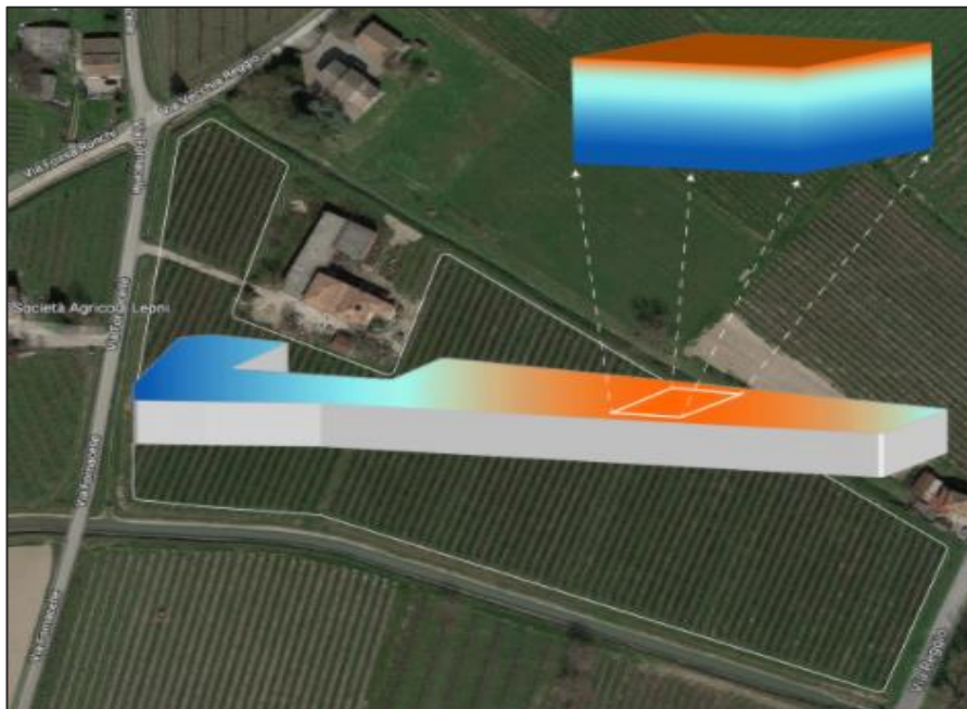
FIGURA 14 – ZONIZZAZIONE AREE IN BASE A VIGORE E/O STRESS IDRICO
