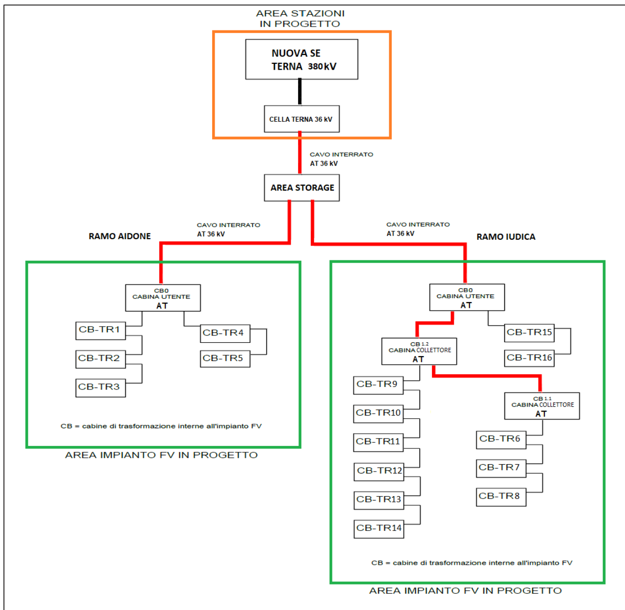
FIGURA 10: SCHEMA A BLOCCHI IMPIANTO
