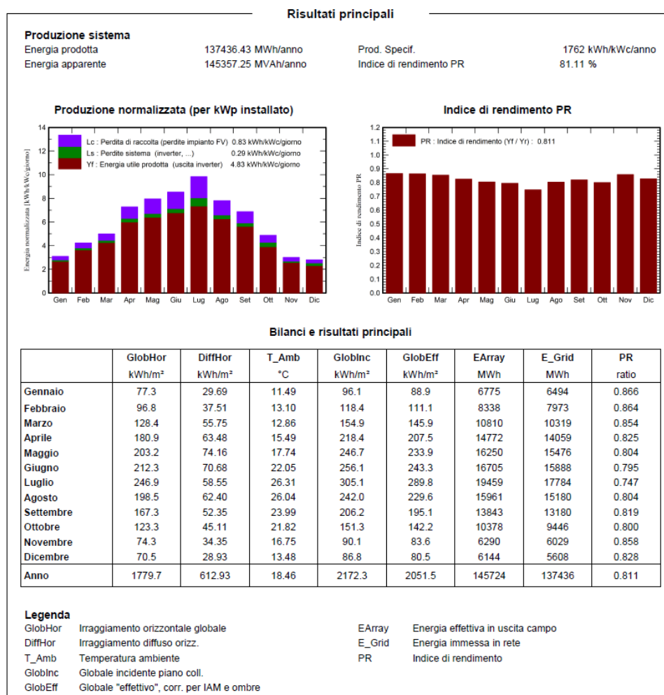
FIGURA 8: PRODUCIBILITA' ELETTRICA DELL'IMPIANTO AGRIVOLTAICO VALUTATA TRAMITE PVSYS
