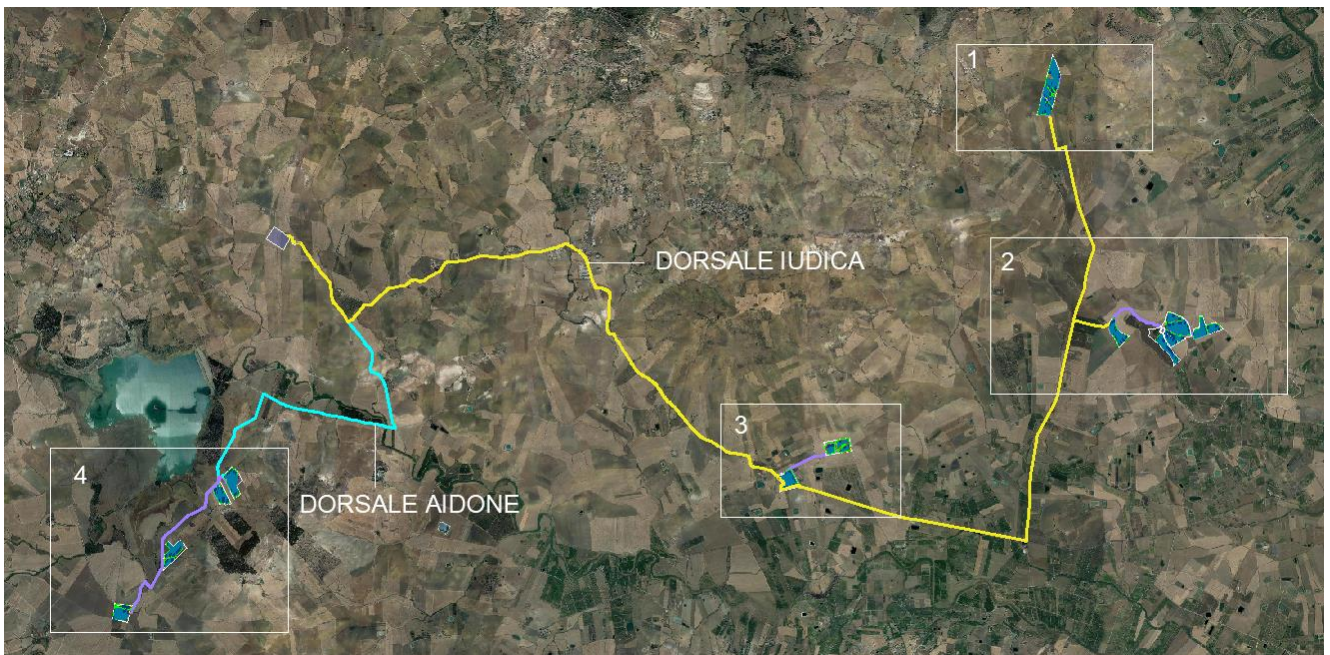
FIGURE 1: INQUADRAMENTO TERRITORIALE SU ORTOFOTO DELLE 4 MACROAREE DI IMPIANTO E DELLE 2 DORSALI ELETTRICHE
