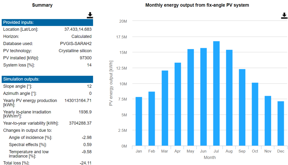
FIGURA 9: PRODUCIBILITA' ELETTRICA DELL'IMPIANTO FOTOVOLTAICO STANDARD VALUTATA TRAMITE PVGIS
