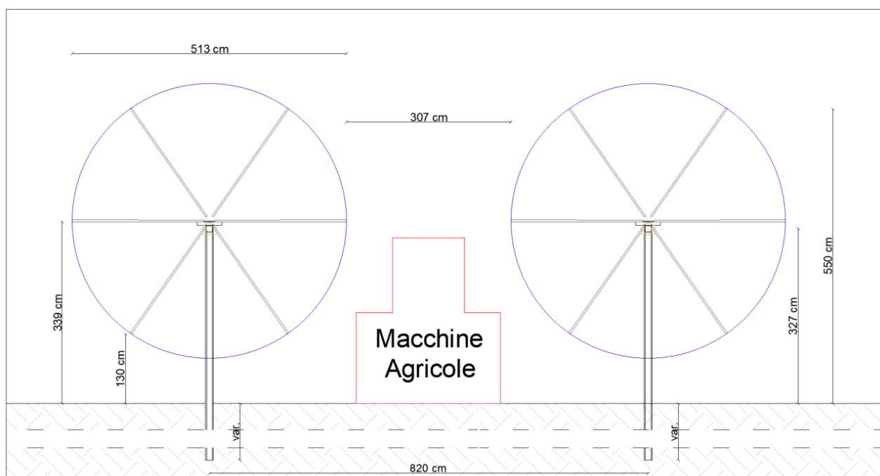
FIGURA 7: CONFIGURAZIONE STRUTTURE AD INSEGUIMENTO IMPIANTO AGRIVOLTAICO
