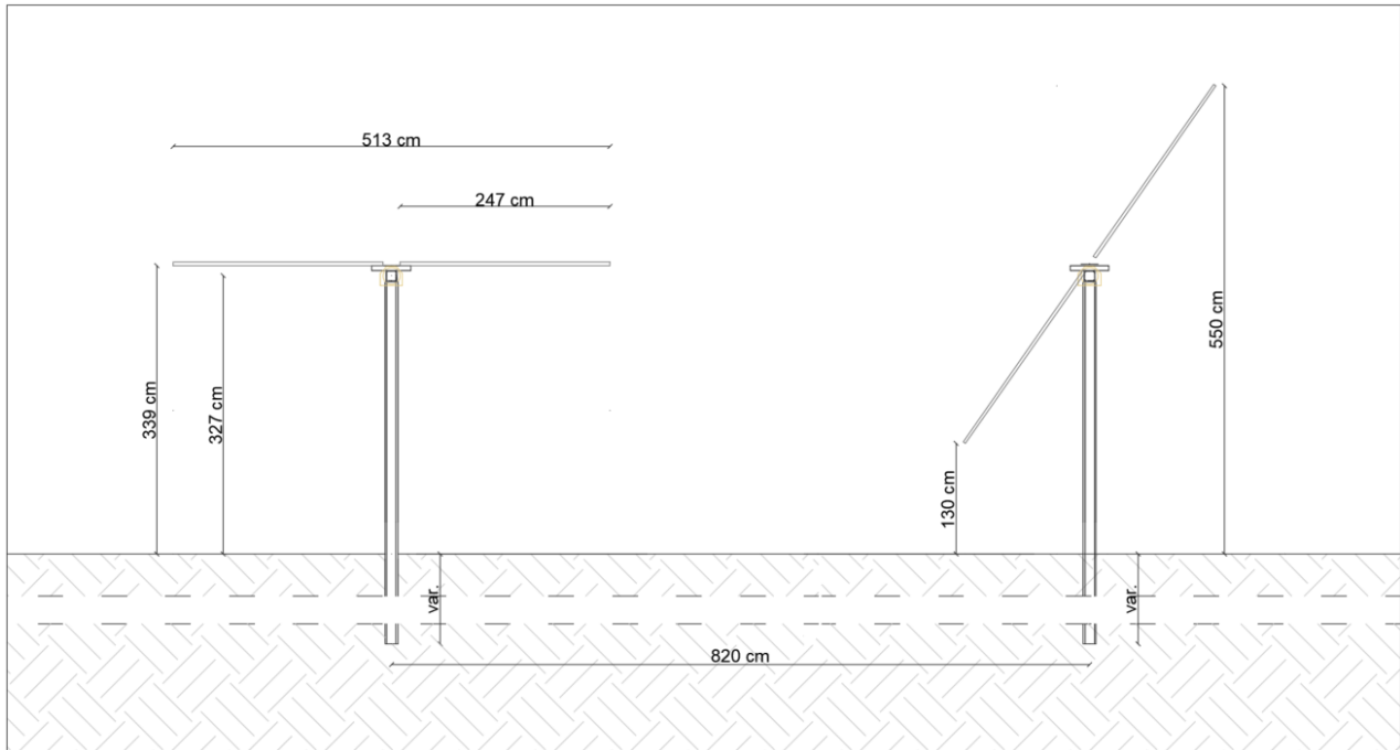
FIGURA 1: TRACKER TIPO AD ASSE VARIABILE
