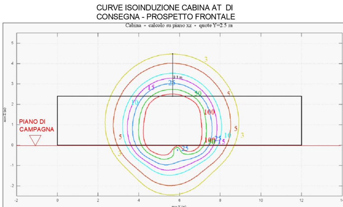
FIGURA 7: CURVE ISOINDUZIONE CABINA AT DI CONSEGNA (PROSPETTO FRONTALE)
