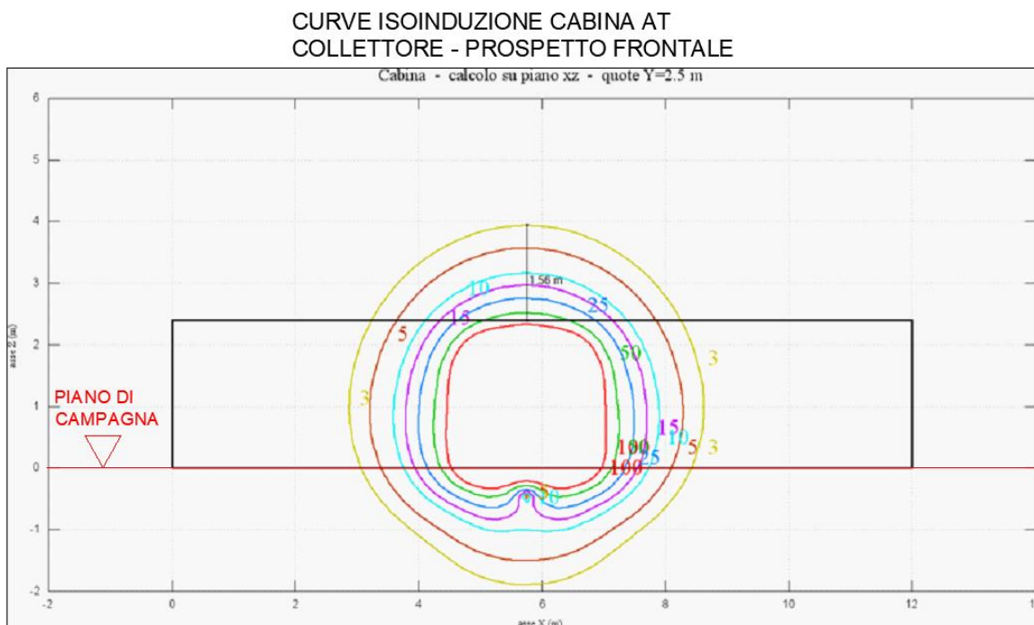
FIGURA 6: CURVE ISOINDUZIONE CABINA AT COLLETTORE (PROSPETTO FRONTALE)
