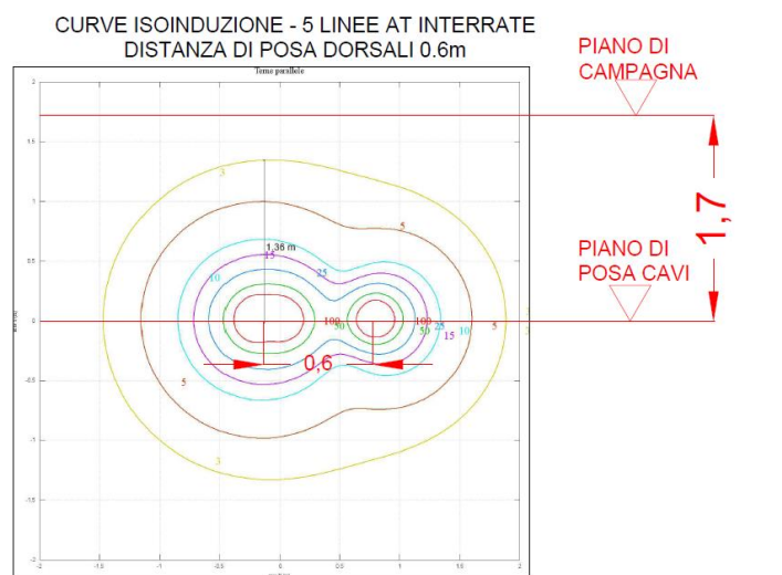
FIGURA 3: CURVE ISOINDUZIONE DOPPIA DORSALE - 2
