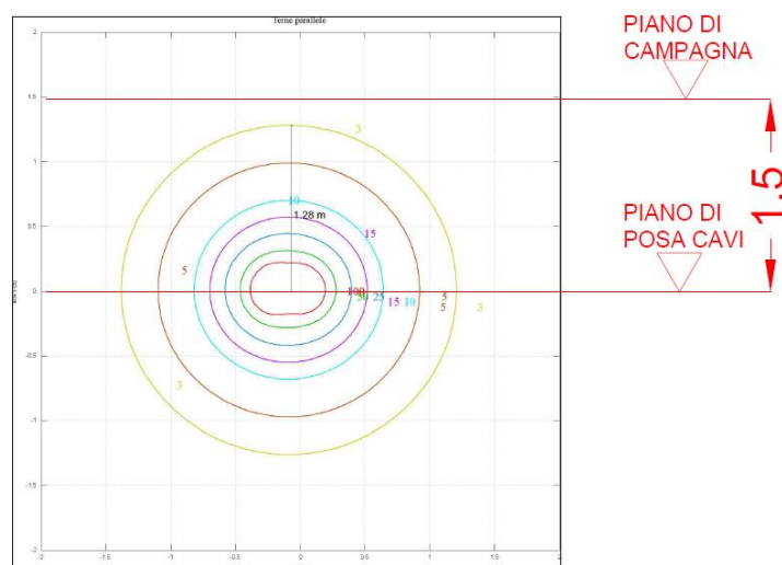
FIGURA 2: CURVE ISOINDUZIONE SINGOLA DORSALE - 1
