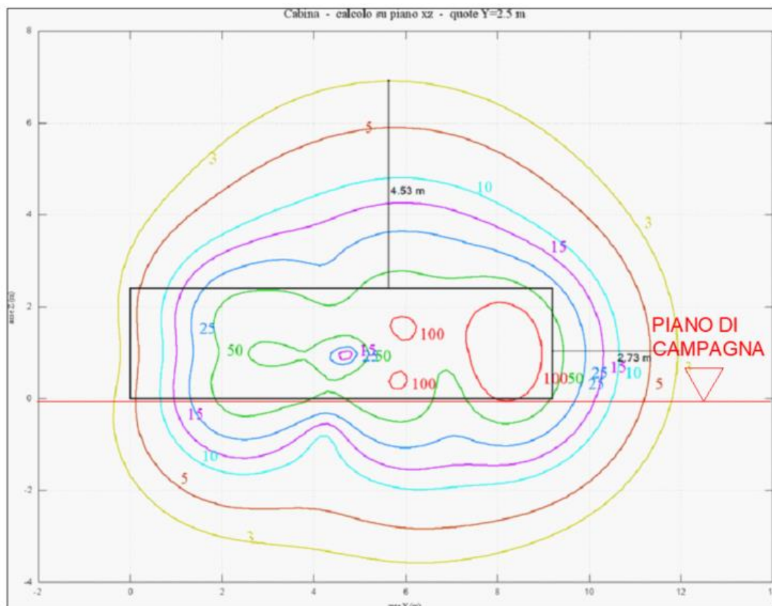
FIGURA 5: CURVE ISOINDUZIONE CABINA AT/BT DI SOTTOCAMPO (PROSPETTO FRONTALE)
