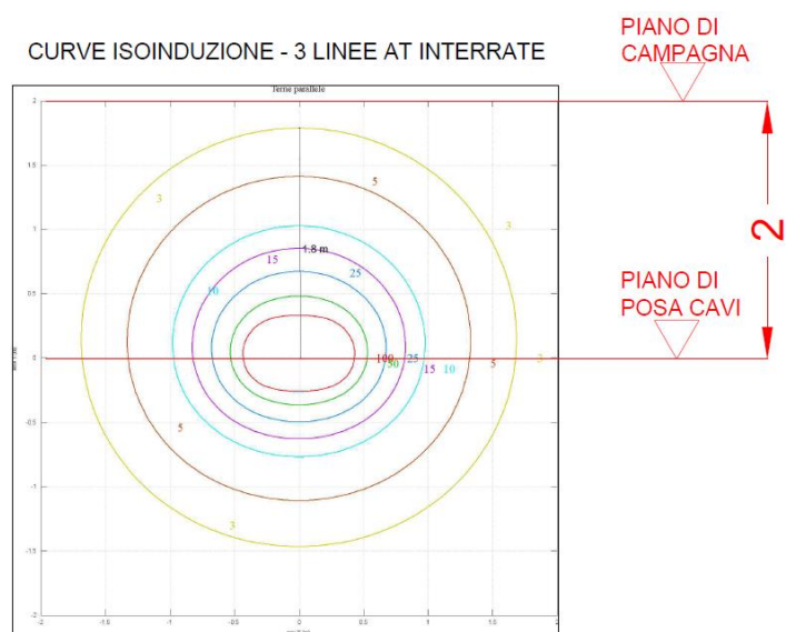
FIGURA 4: CURVE ISOINDUZIONE TRATTO CABINA DI CONSEGNA FINALE-SE TERNA - 3
