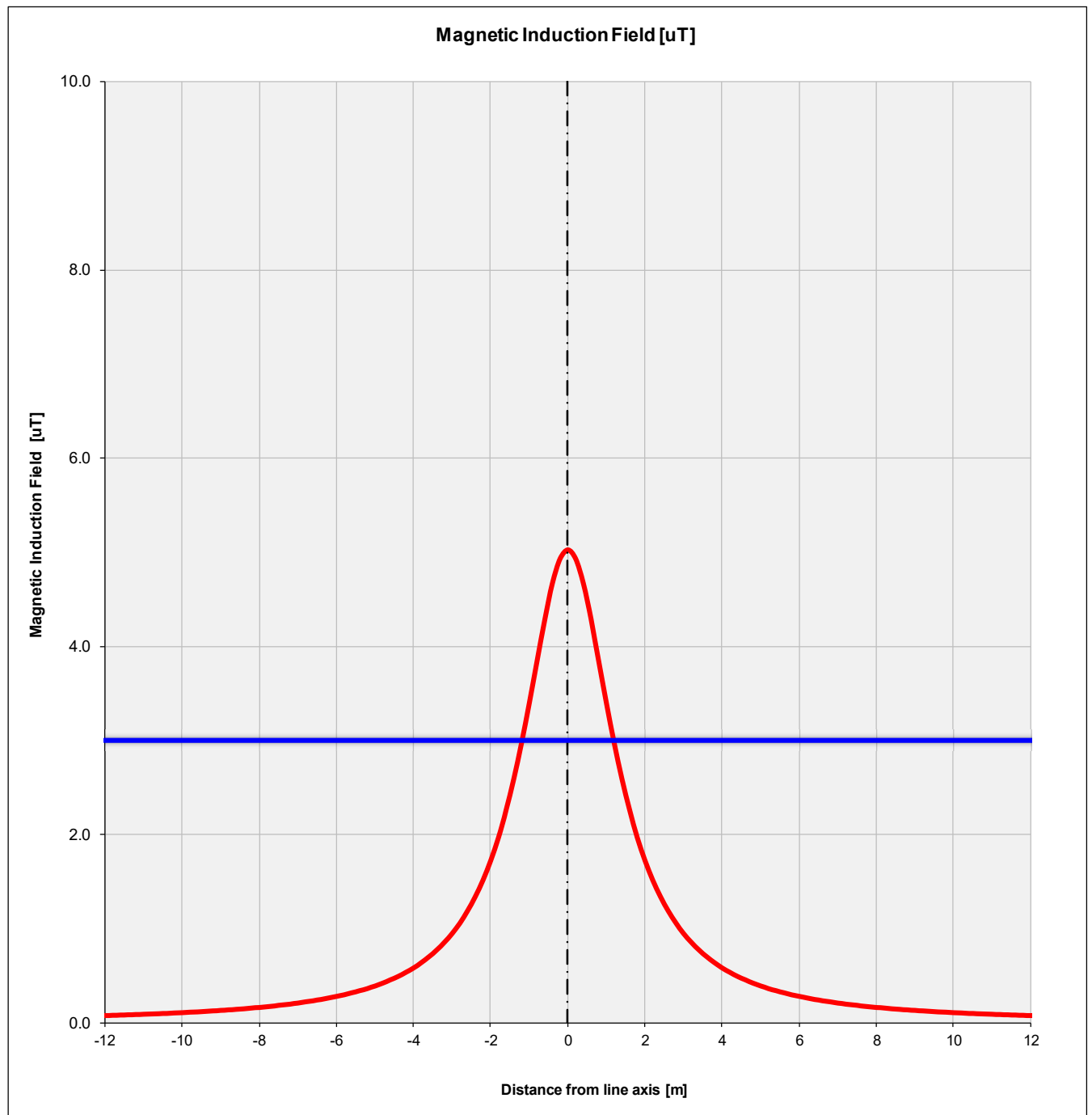
Figura 11: Andamento dell'induzione magnetica prodotta dalla linea in cavo AT
