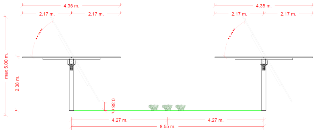
Schema coltivazione agro-fotovoltaico
