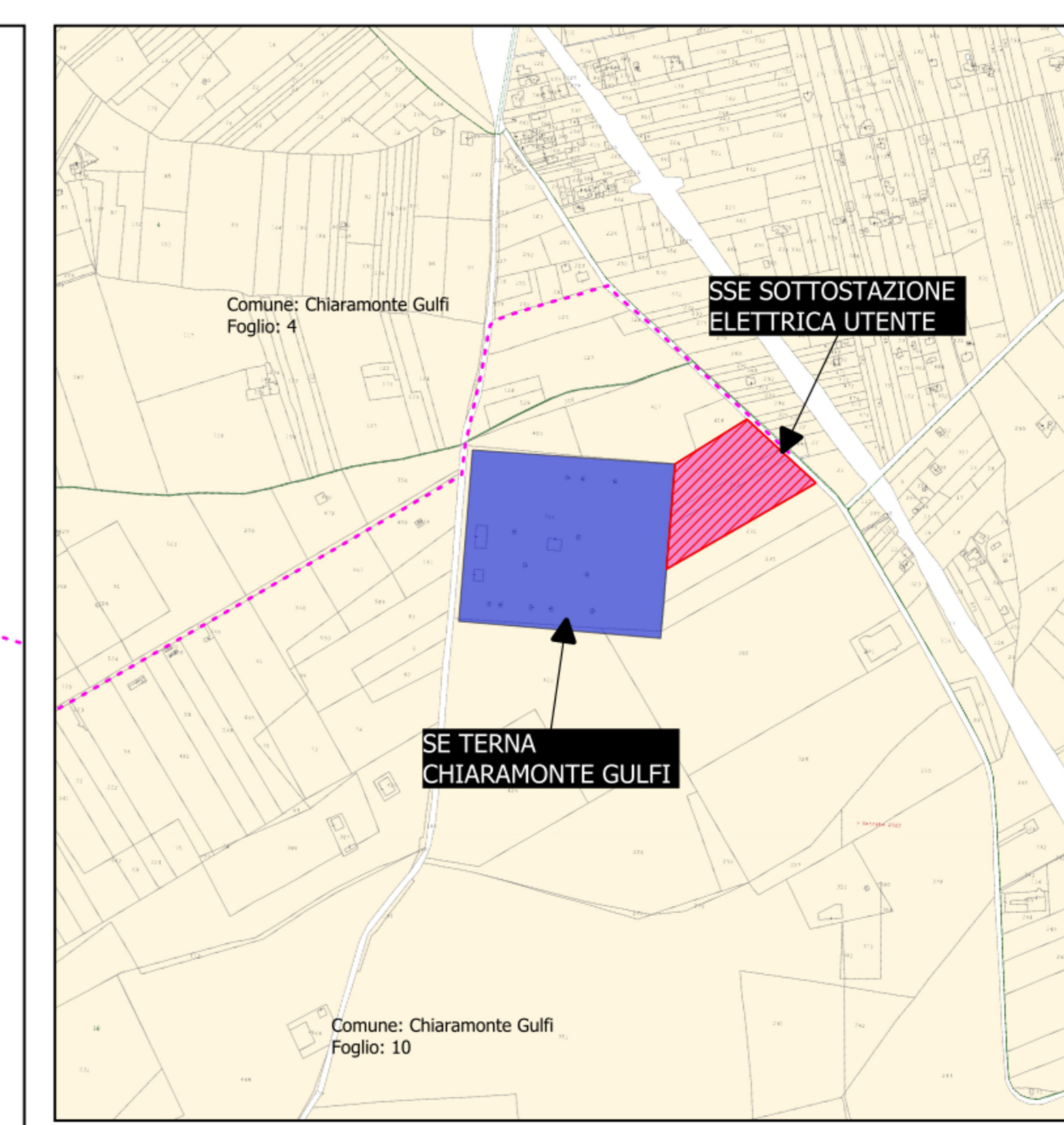
Planimetra Catastale con SE TERNA e SSE - Scala 1:7.000
