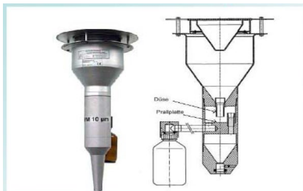
Fig. 5 - Testa di campionamento per il prelievo del particolato
