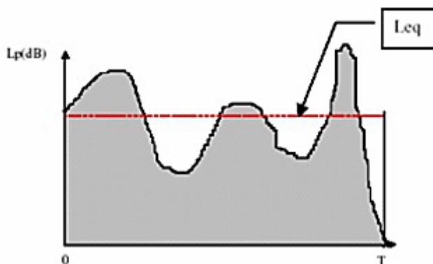
Fig. 27 - Schema rappresentativo del Leq
