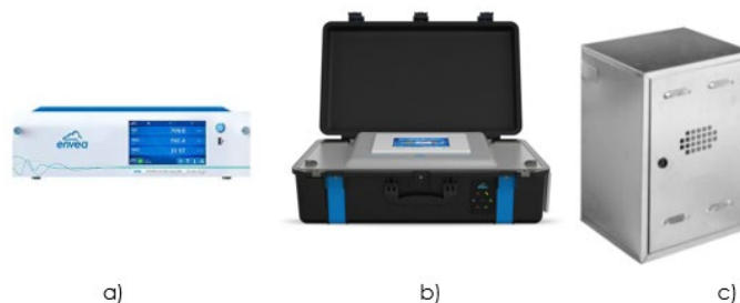
Fig. 8 - Stazione mobile per il monitoraggio degli inquinanti da traffico veicolare. a) Misuratore ossidi di azoto a chemiluminescenza; b) Misuratore CO a infrarossi; c) cassetta zincata protezione sonde.
