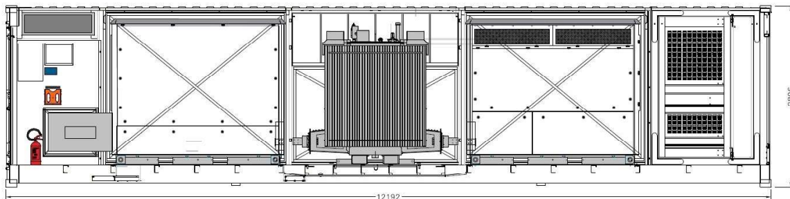
LAYOUT TIPOLOGICO CABINA DI CONVERSIONE
