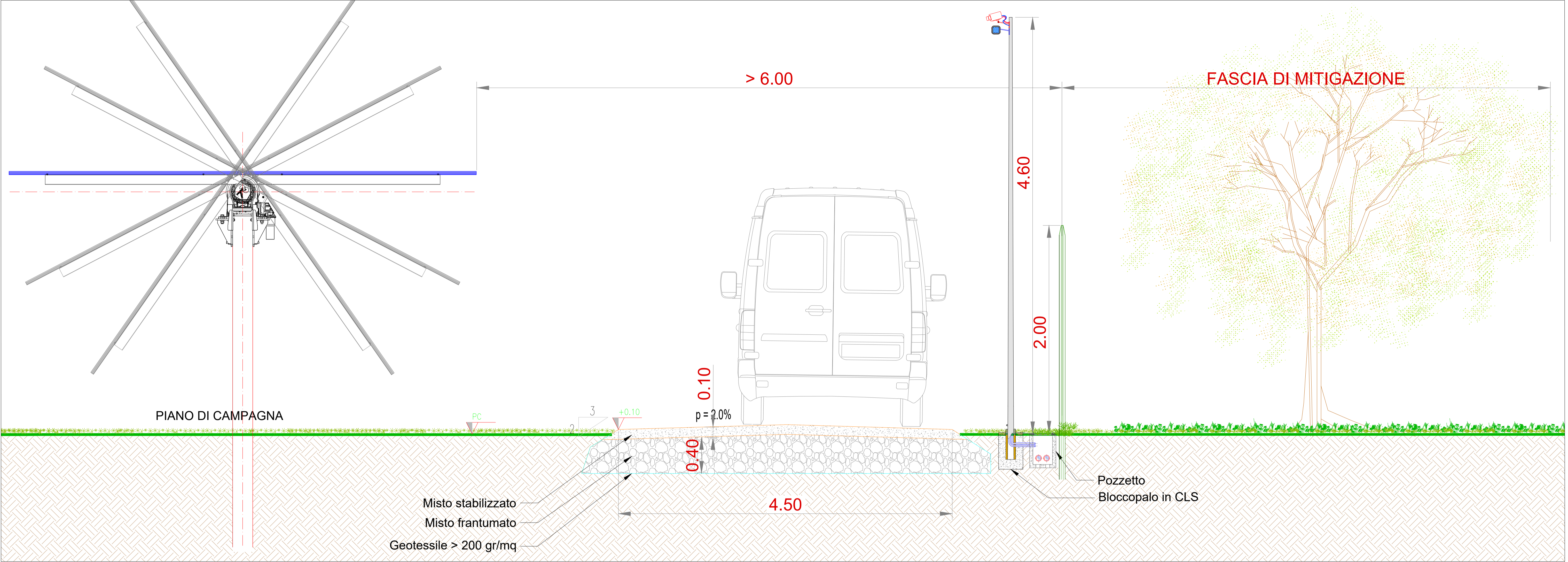
Viabilità di progetto a carattere rurale - Sezione tipologica viabilità interfilare - scala 1:20
