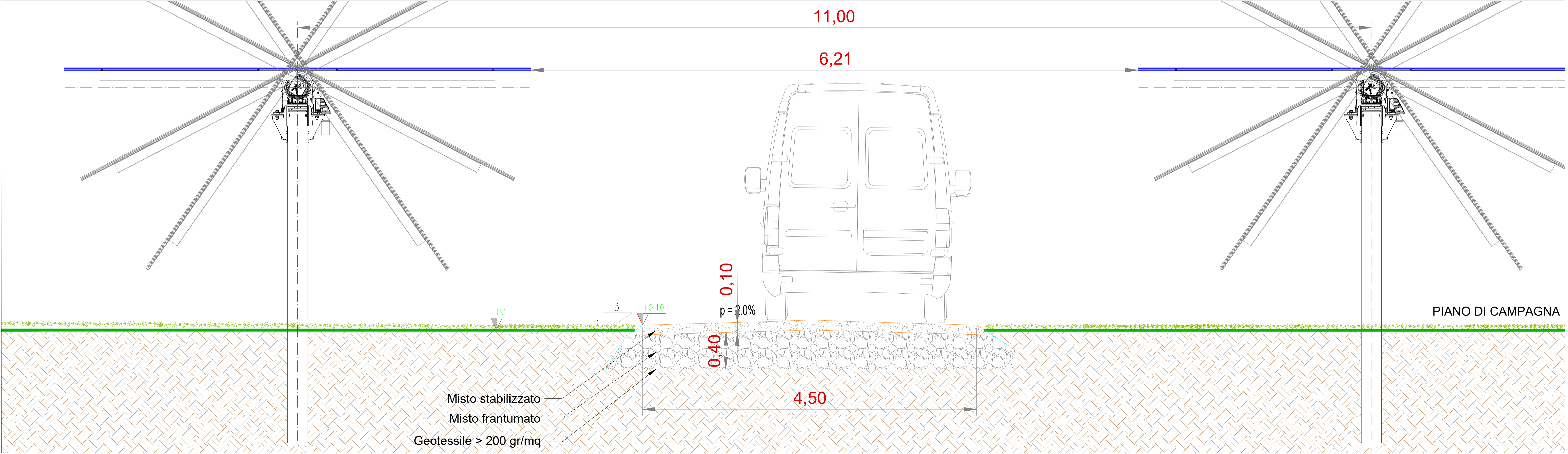
Viabilità di progetto a carattere rurale - Sezione tipologica viabilità interfilare - scala 1:20
