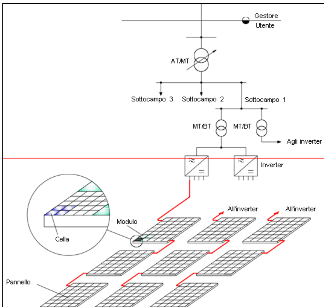
Fig1: Schema collegamento centrale fotovoltaica
