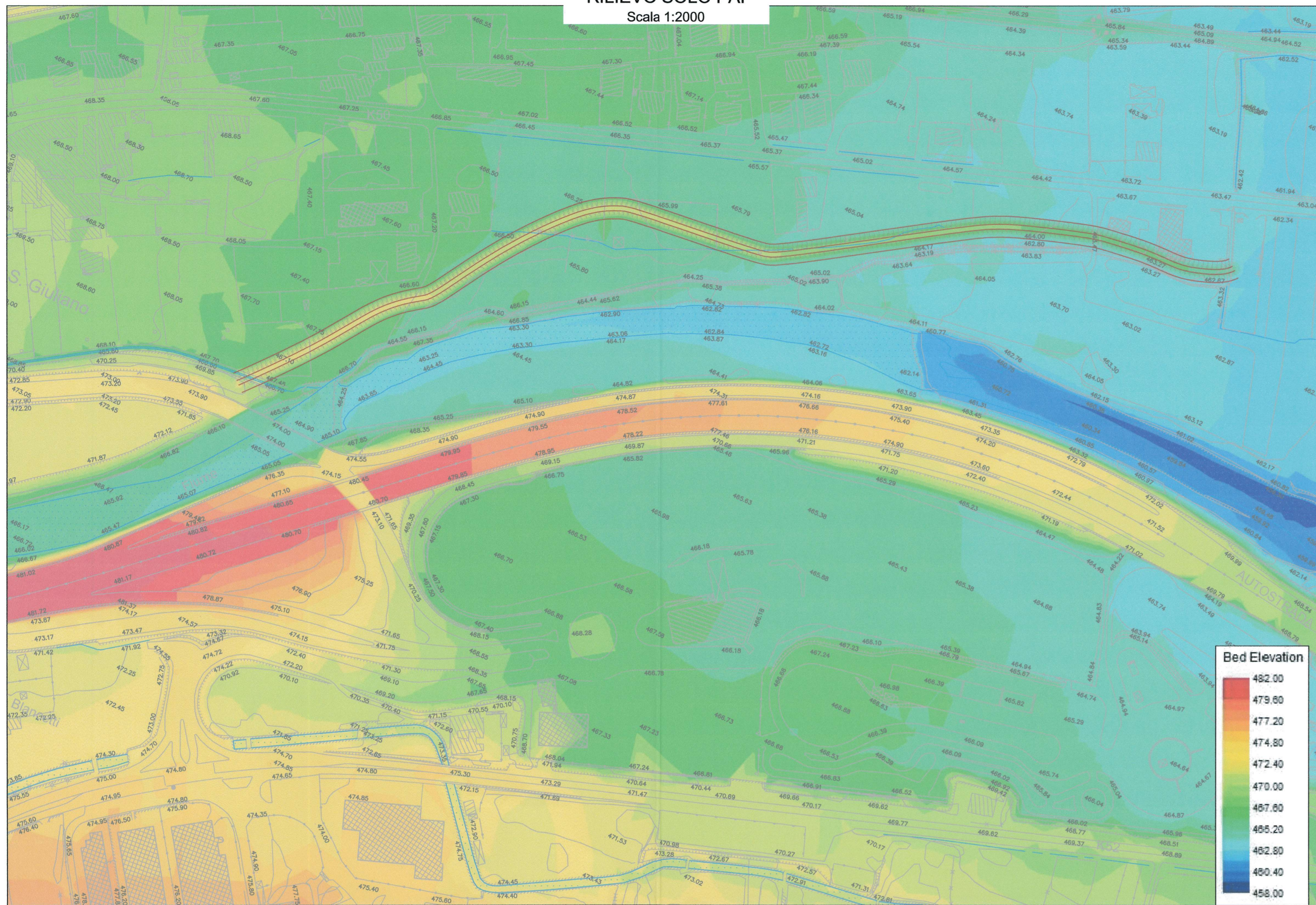
PROGETTO PAI E PONTE LTF SENZA FORNICI Scala 1:2000
