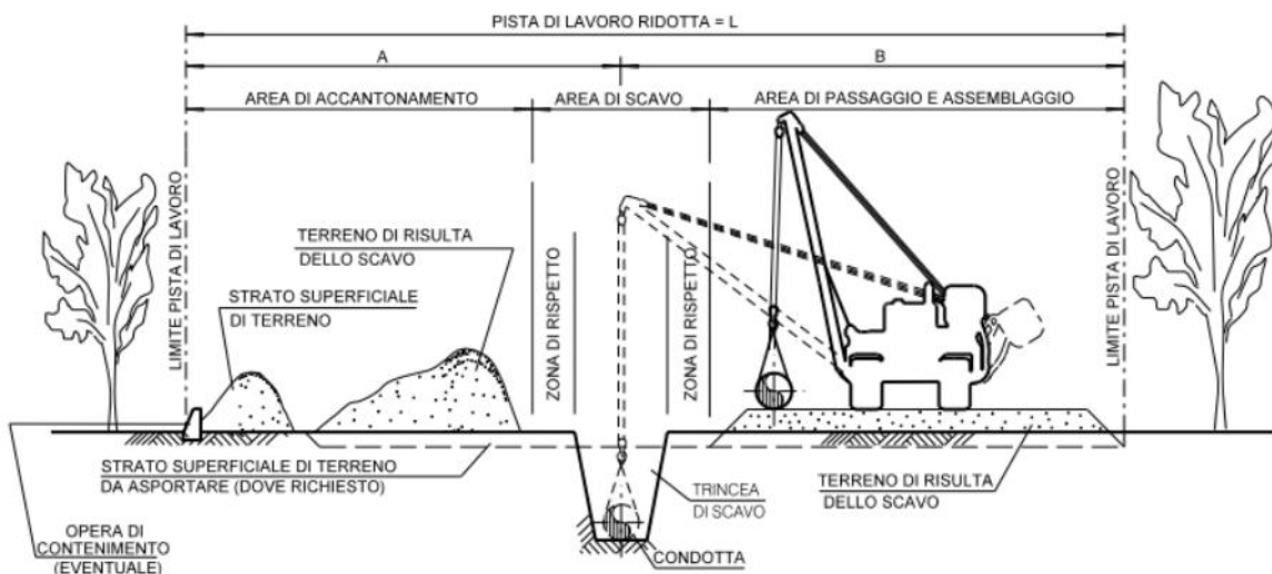
Figura 10: Disegno tipologico indicativo dei movimenti di terreno in fase di posa di cavidotti.
