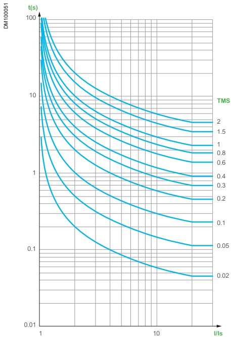
Curva IEC a Tempo Inverso (IEC/SIT o IEC/A)
