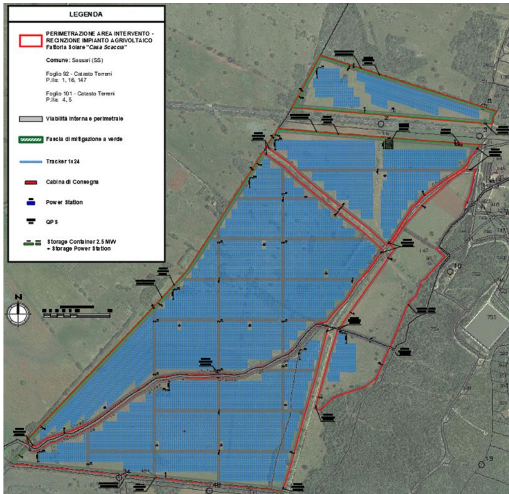
Figura 3: Layout di Impianto
