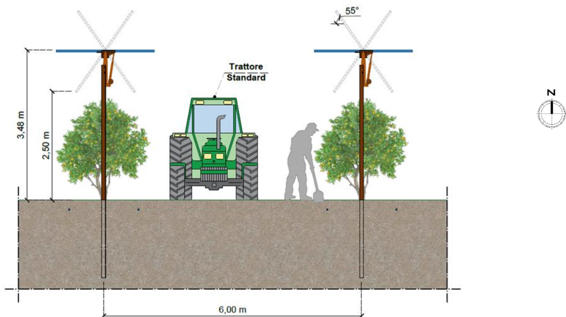
Figura 4: Dettaglio prospetto laterale tracker
