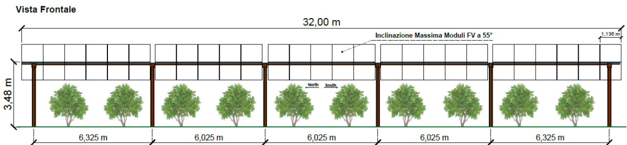
Figura 5: Dettaglio prospetto frontale tracker
