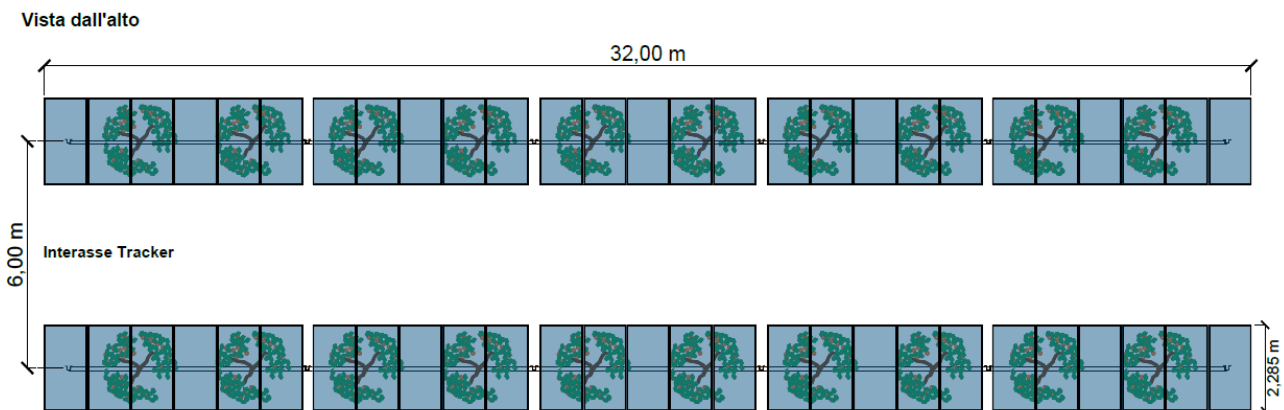
Figura 6: Dettaglio vista dall'alto tracker
