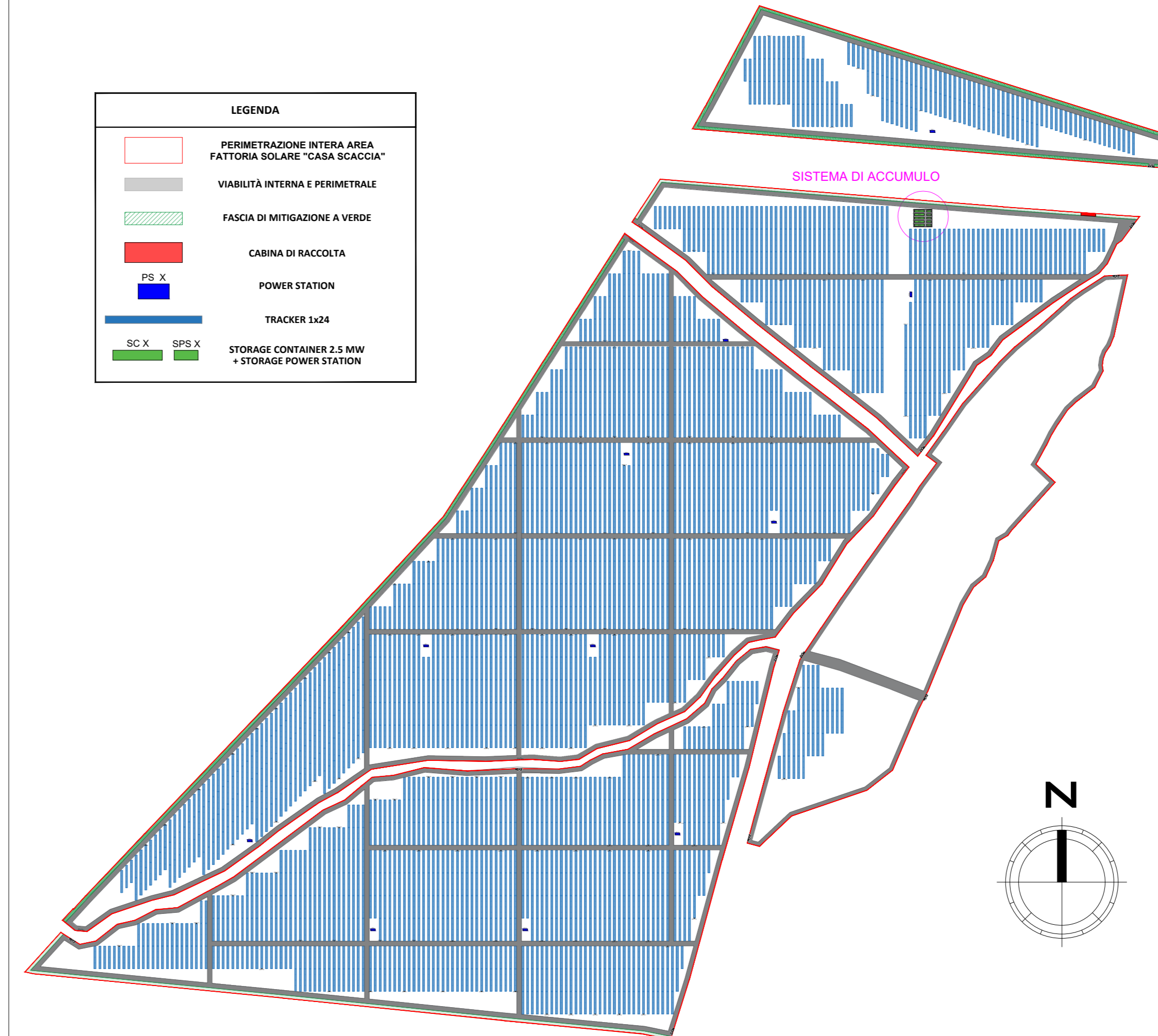
LAYOUT IMPIANTO CON EVIDENZA AREA SISTEMA DI ACCUMULO - SCALA 1:5.000
