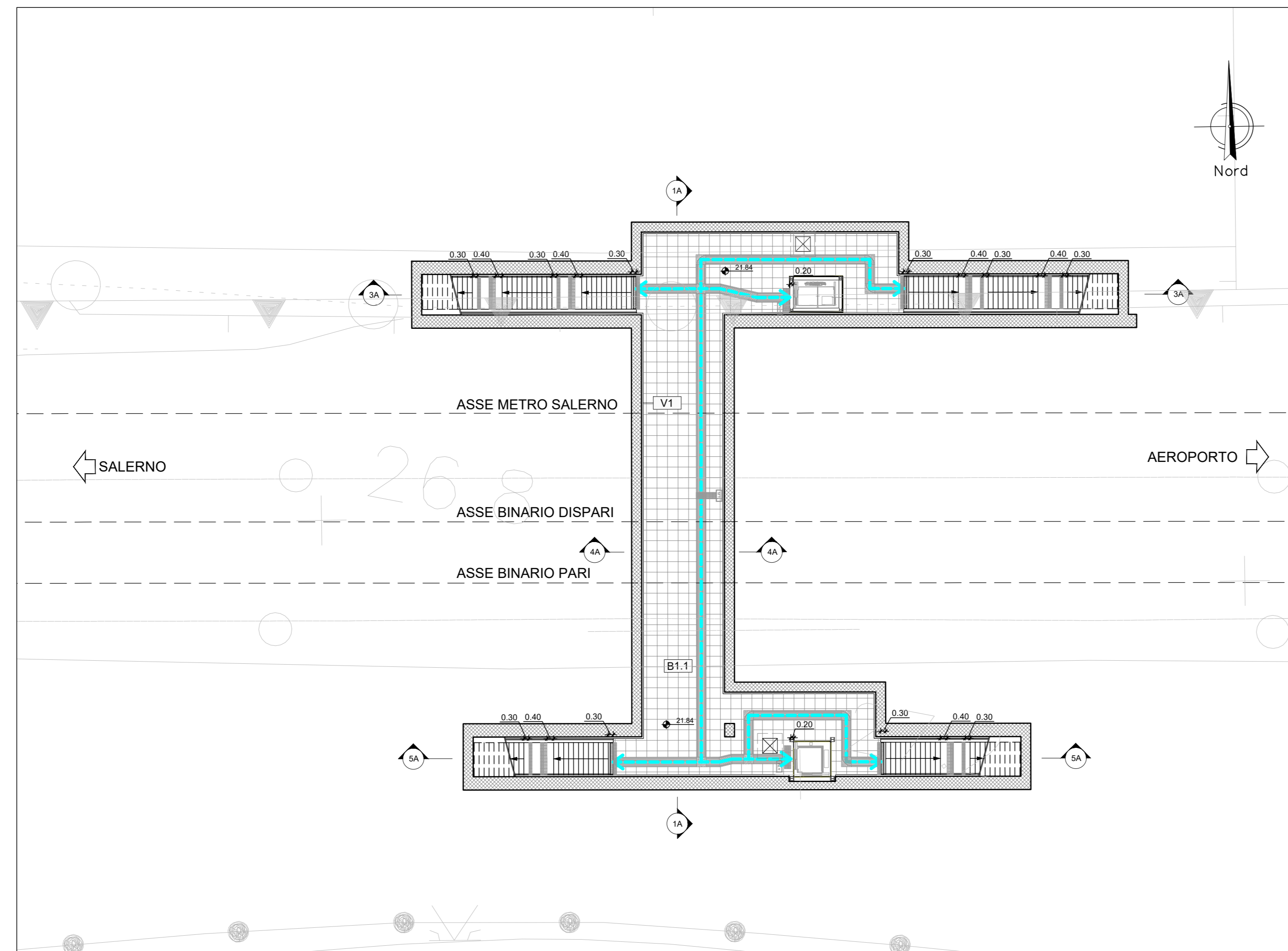
Pianta Quota Sottopasso con individuazione percorso privo di ostacoli 1 : 200
