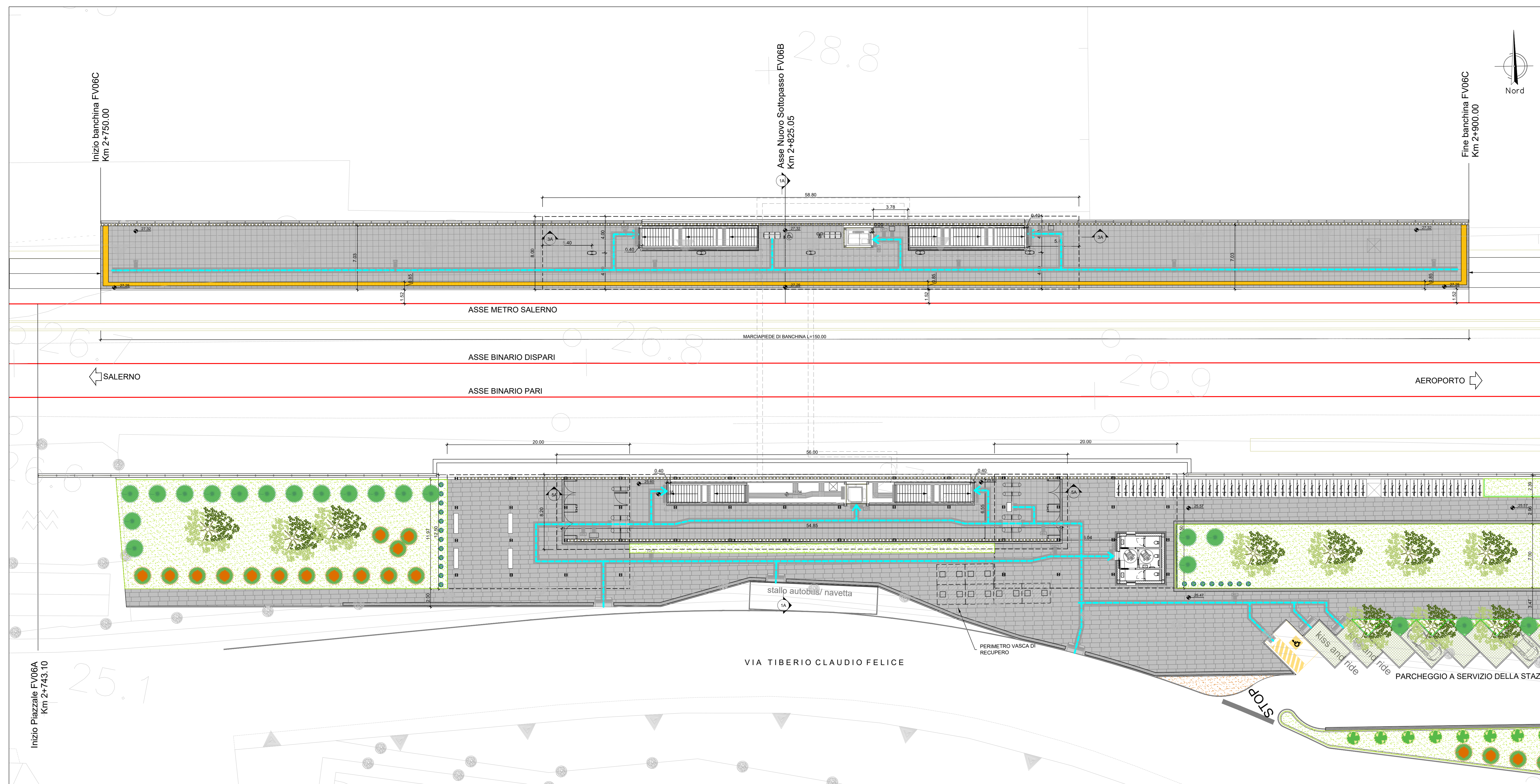
Pianta quota banchina con individuazione percorso privo di ostacoli 1 : 200
