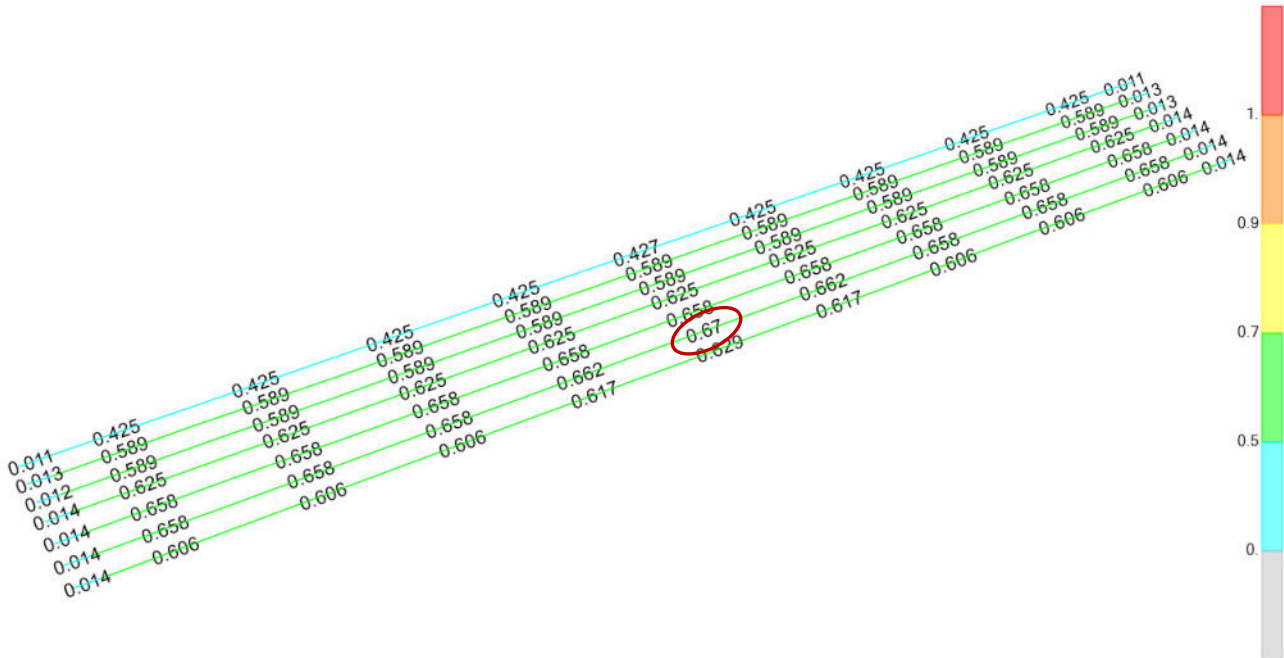
Arcarecci IPE 180 – Coefficienti di sfruttamento relativi alle verifiche di resistenza e instabilità per sforzi assiali e flettenti
