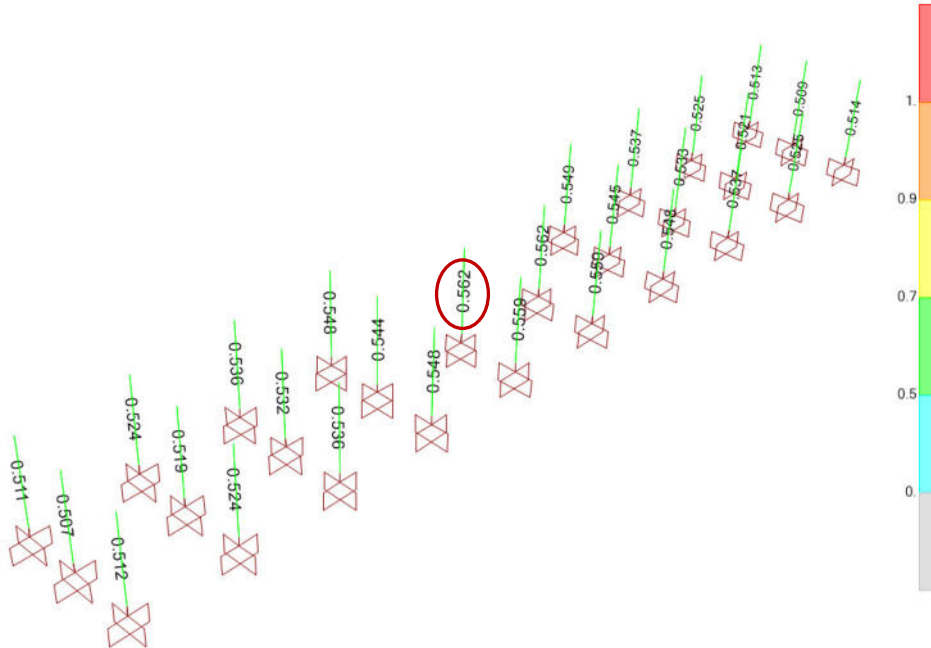
Colonne HEA 240 – Coefficienti di sfruttamento relativi alle verifiche di resistenza e instabilità per sforzi assiali e flettenti
