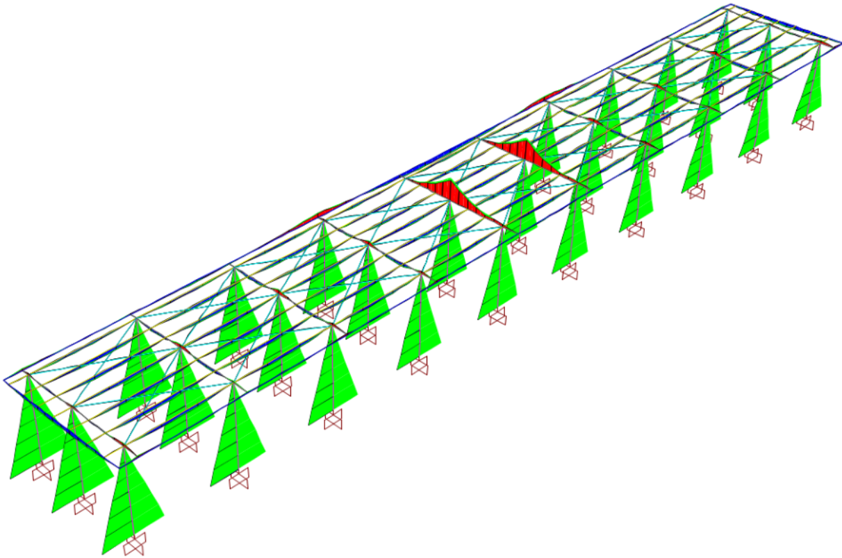
Inviluppo dei momenti flettenti (asse forte) – Combinazioni SLV
