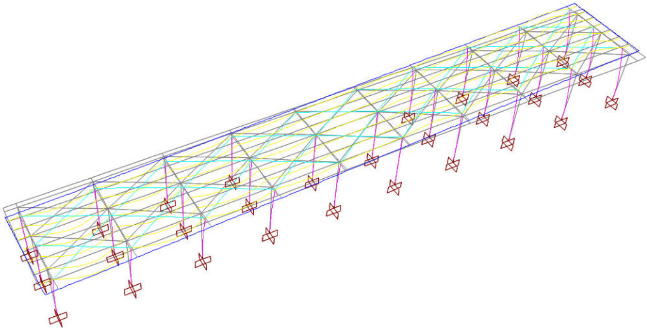
Modo 2 (rotazionale) – T=1.03s – Massa partecipante=86%
