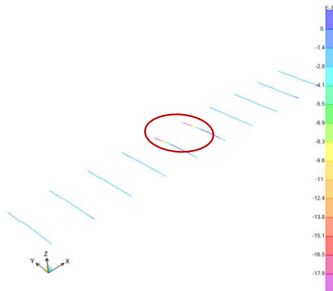
Travi 2UPN 240 – Spostamenti verticali massimi Travi principali
