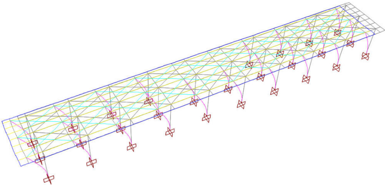
Modo 3 (traslazionale dir. X) – T=0.574s – Massa partecipante=96%
