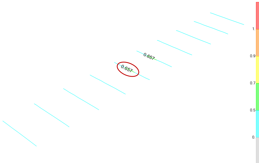
Travi UPN 240 – Coefficienti di sfruttamento relativi alle verifiche di resistenza e instabilità per sforzi assiali e flettenti
