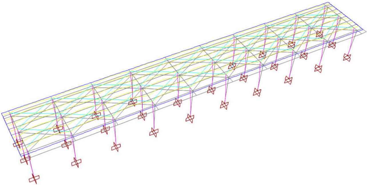
Modo 1 (traslazionale dir. Y) – T=1.13s – Massa partecipante=89%
