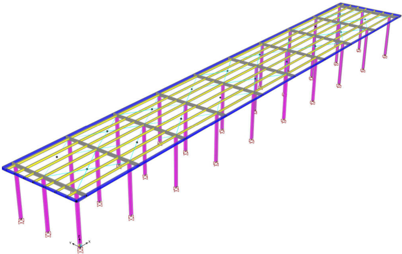
Modello F.E.M. – Vista 3D con elementi estrusi
