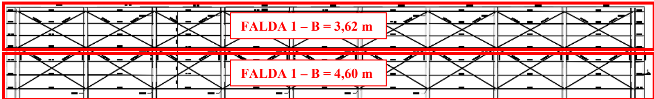
Fig. 1 – Planimetria con particolare orditura di copertura e individuazione falde
