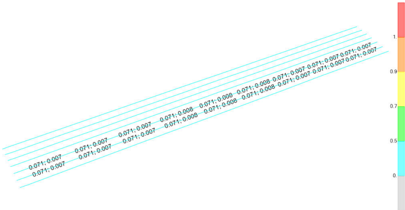
Arcarecci IPE 180 – Coefficienti di sfruttamento relativi alle verifiche di resistenza per sforzi di taglio
