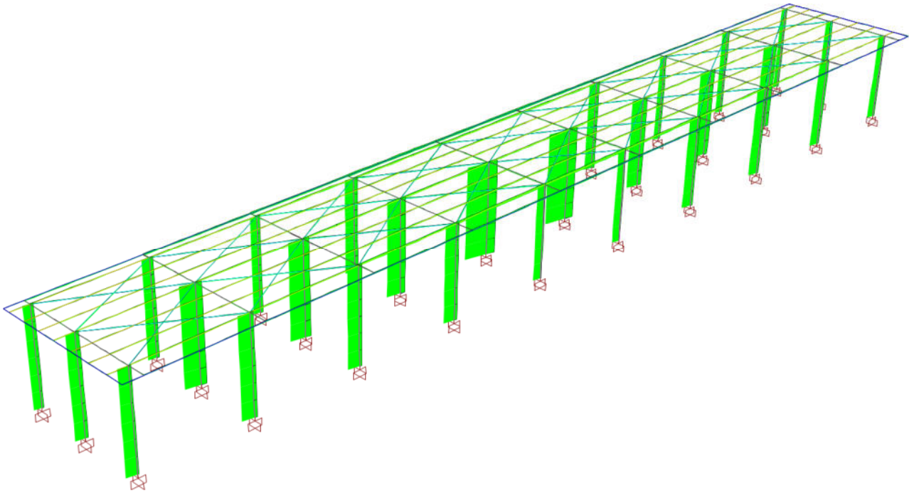
Involuppo degli sforzi assiali – Combinazioni SLU
