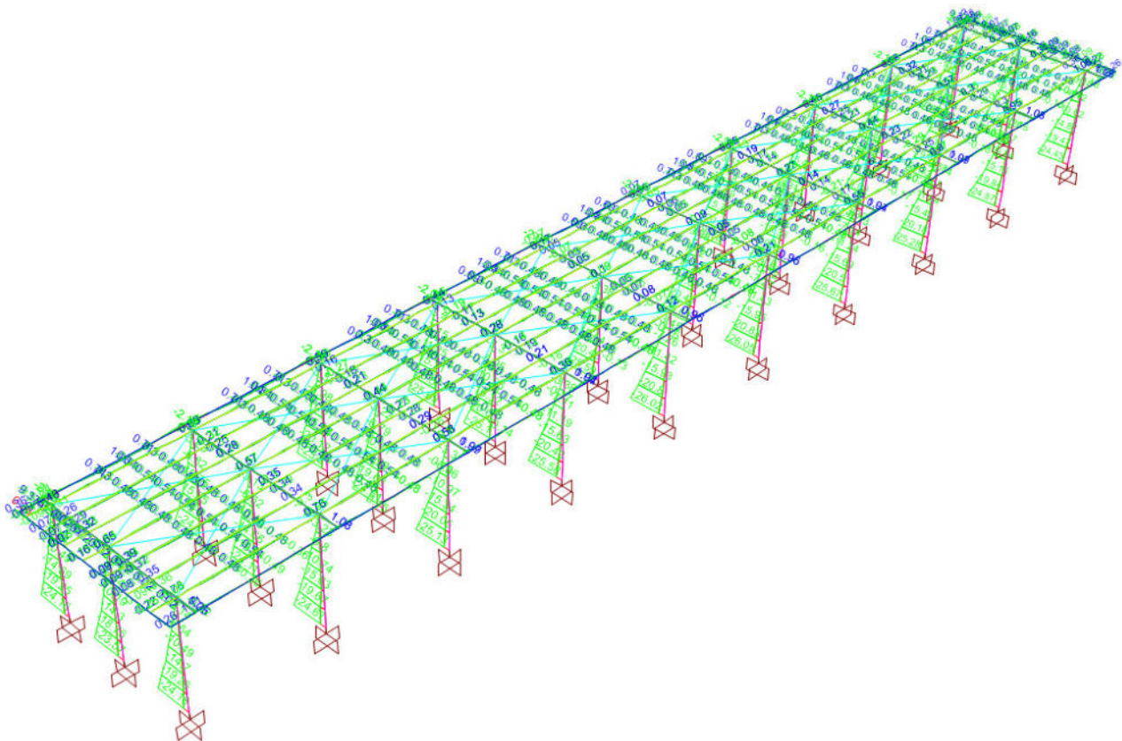
Valori delle sollecitazioni: Inviluppo dei momenti flettenti (asse debole) – Combinazioni SLU
