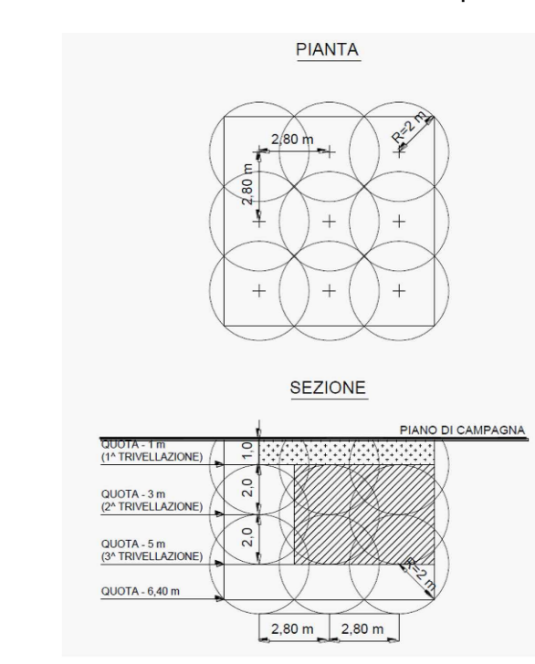
Schema di esecuzione bonifica profonda
