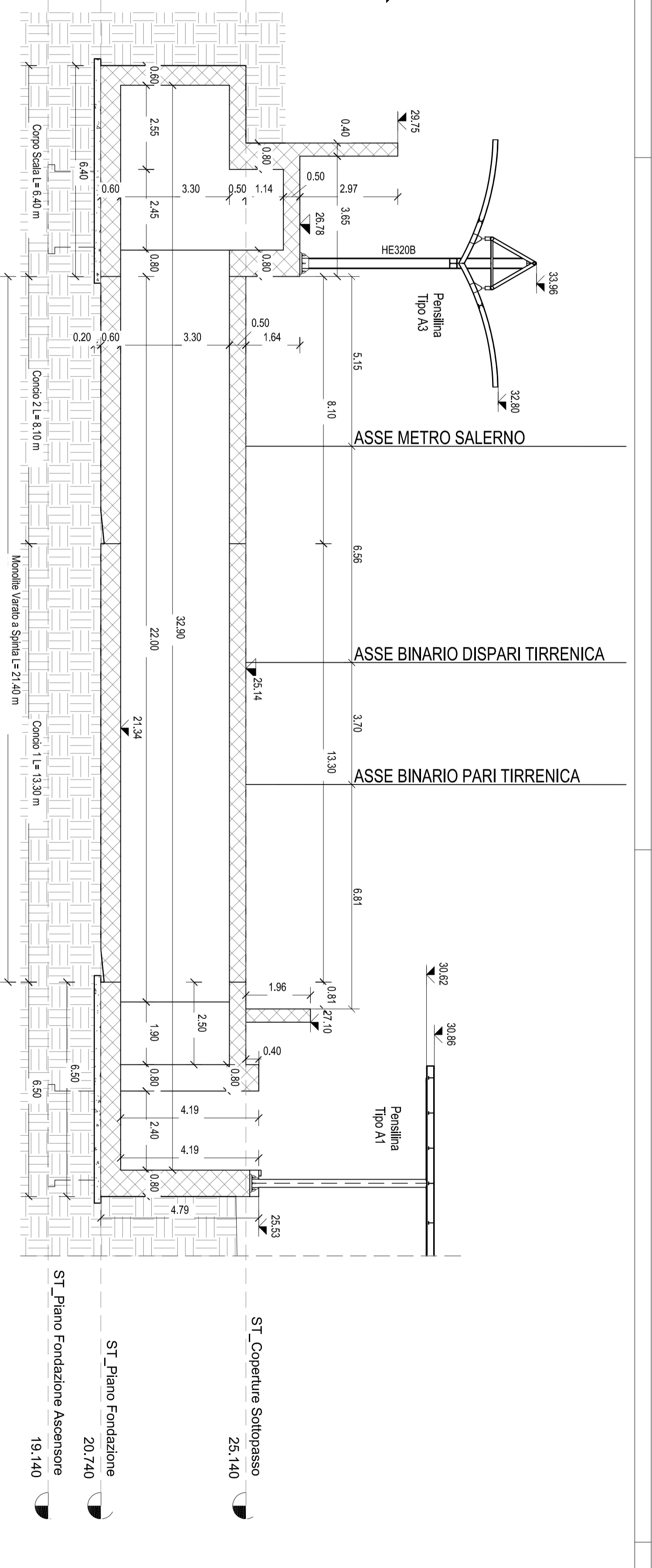
Sez.1A - Longitudinale Sottopasso Pedonale 1 : 100
