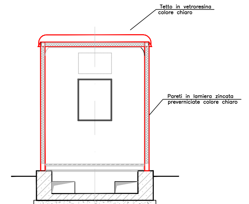
SEZIONE C-C
