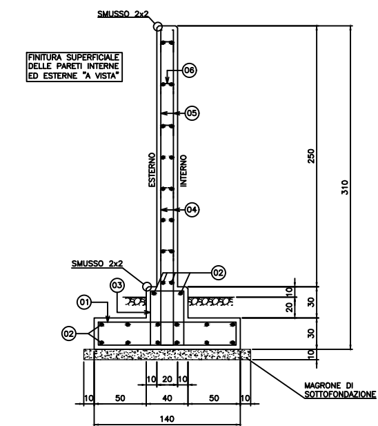
SEZIONE A-A
