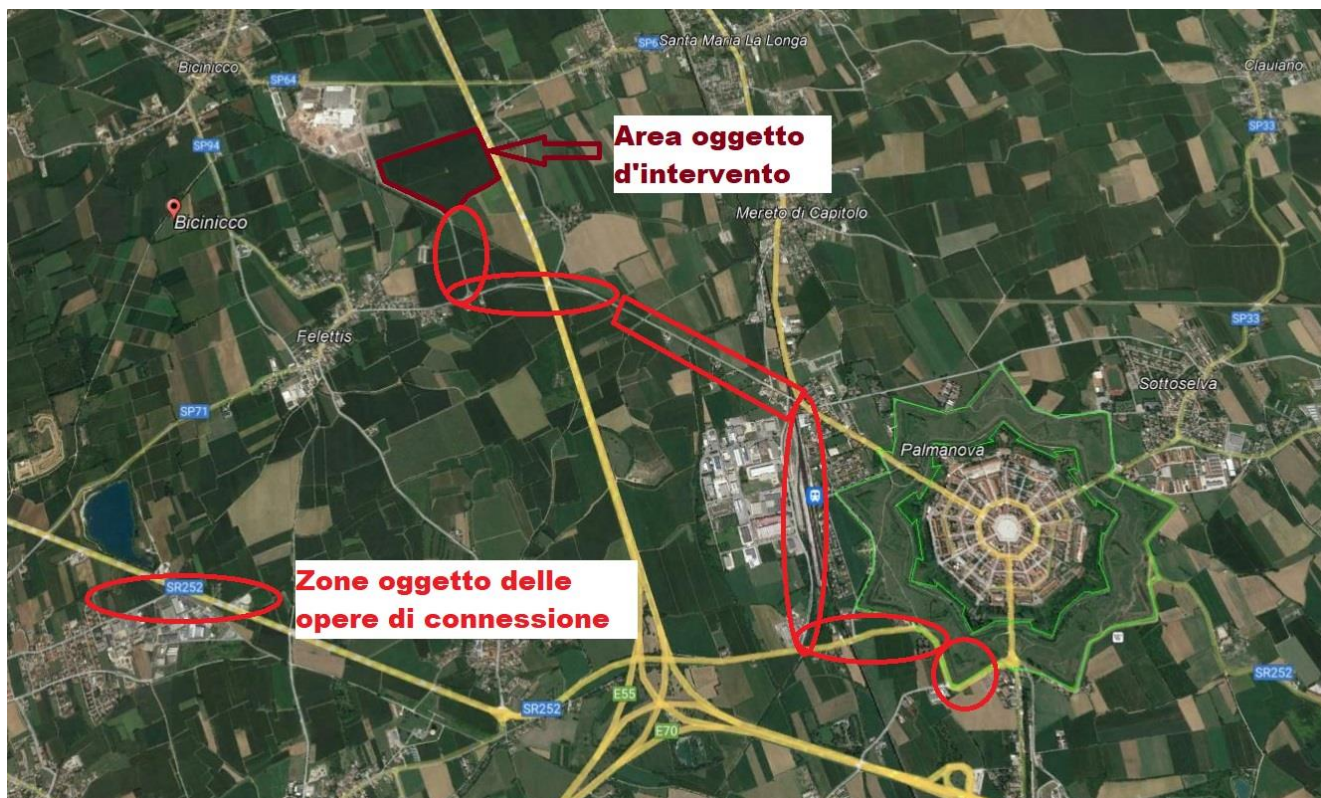
Vista d'insieme dell'impianto di connessione con collegamento cavi MT interrati su base ortofoto
