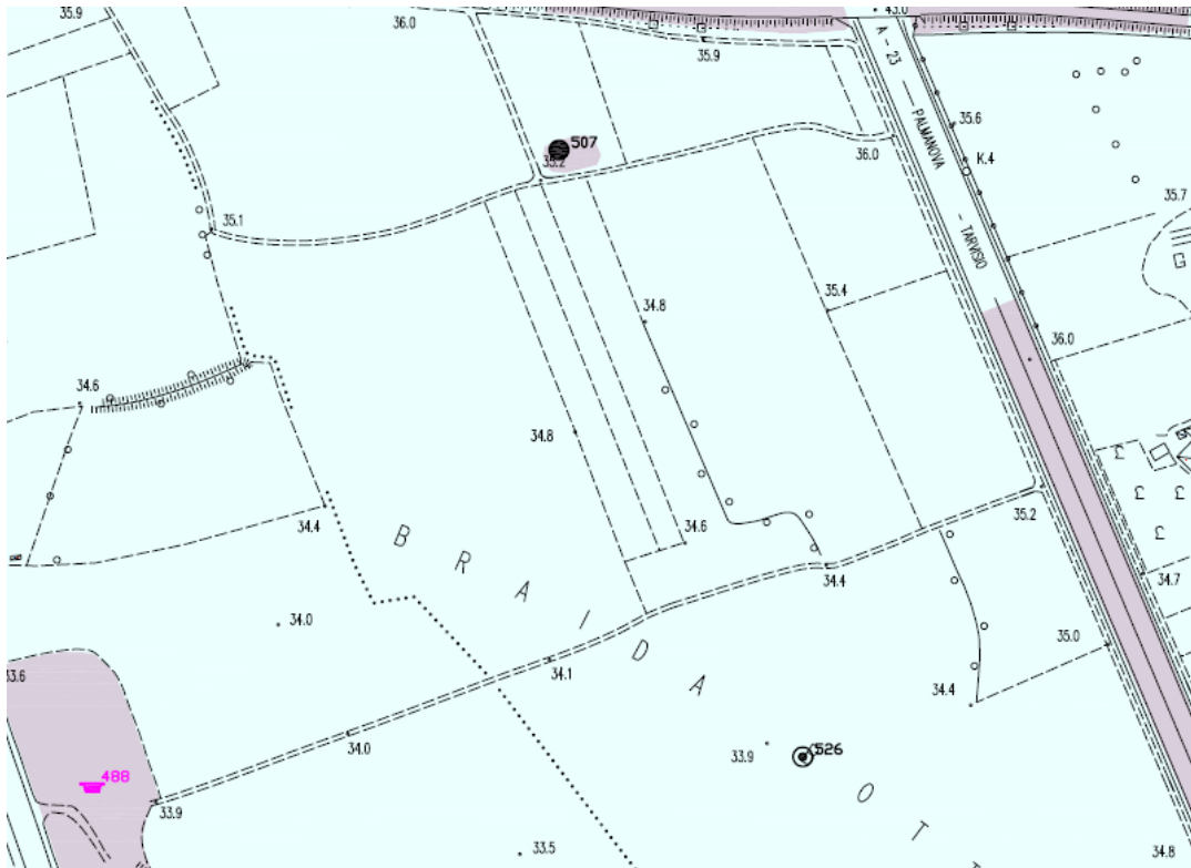
Estratto della carta geologica alla scala 1:5.000 – Servizio Geologico Regione FVG
