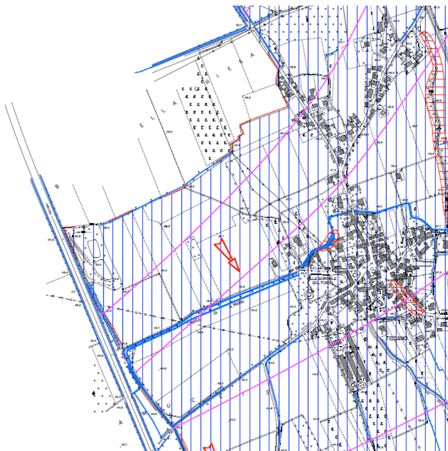
Carta idrogeologica allegata al PRGC del comune di Santa Maria la Longa
