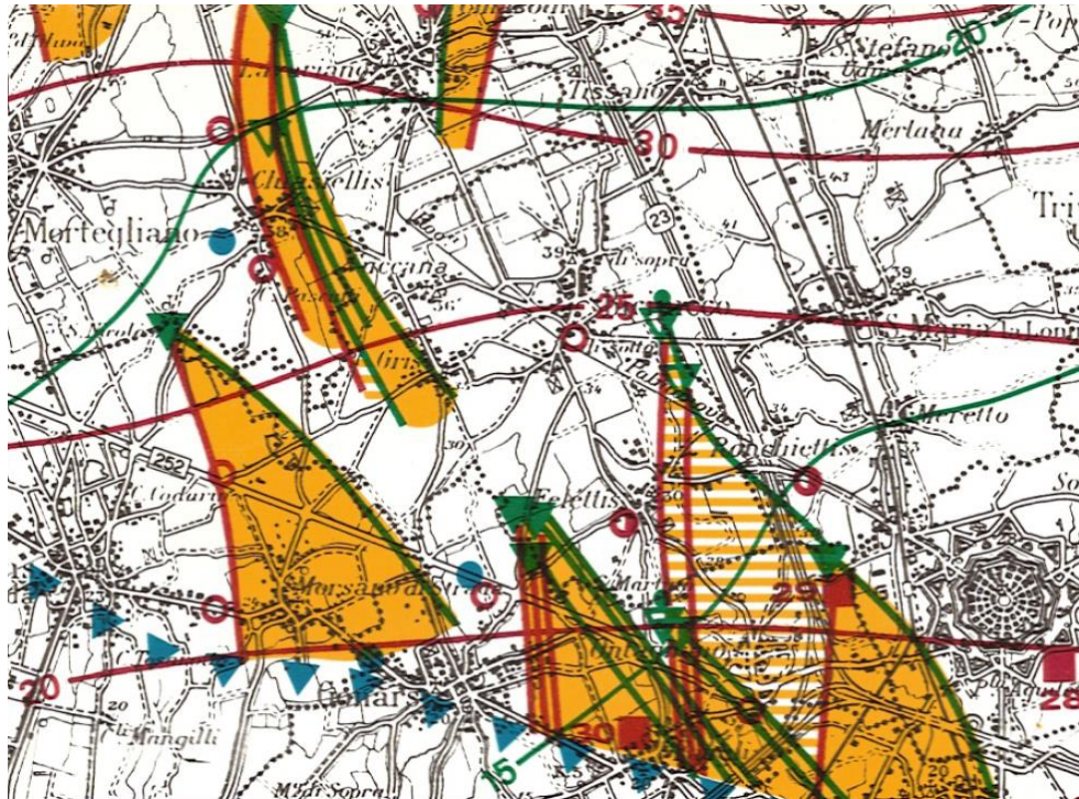
Estratto della Carta delle isofreatiche durante le fasi di massima e minima altezza della falda
