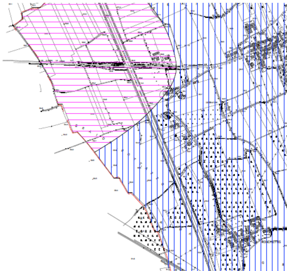
Carta geologica allegata al PRGC di Santa Maria la Longa
